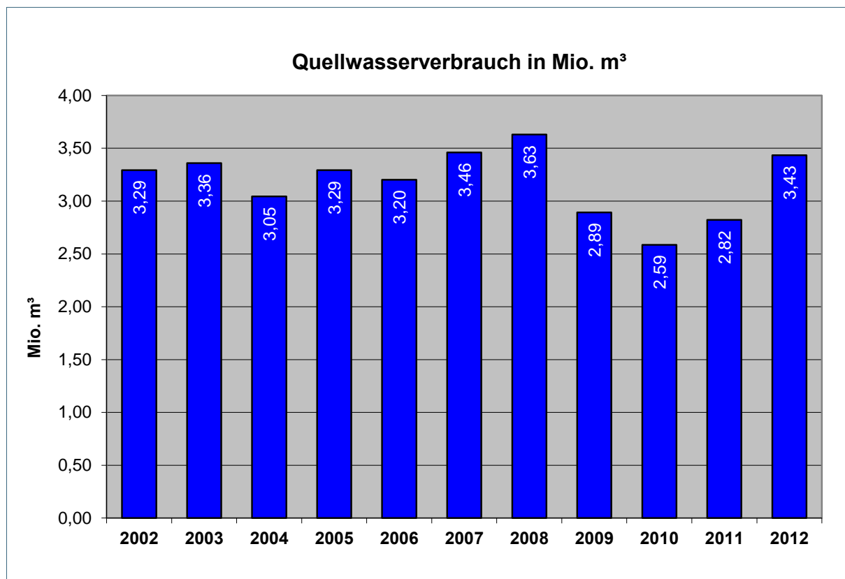
Abb. 59: Quellwasserverbrauch zur Versorgung der Salmonidenanlage
