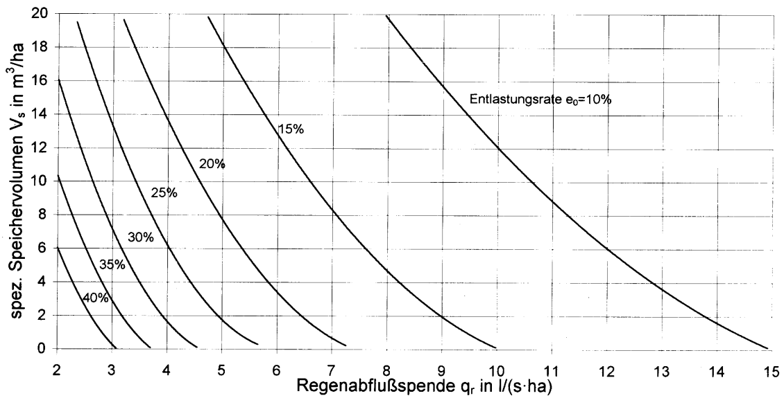
Erweitertes Bild 13 aus dem ATV-Arbeitsblatt A 128
