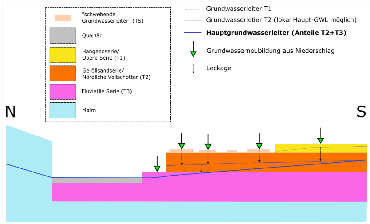
Abb. 32: Schemaprofil des hydrogeologischen Modells
