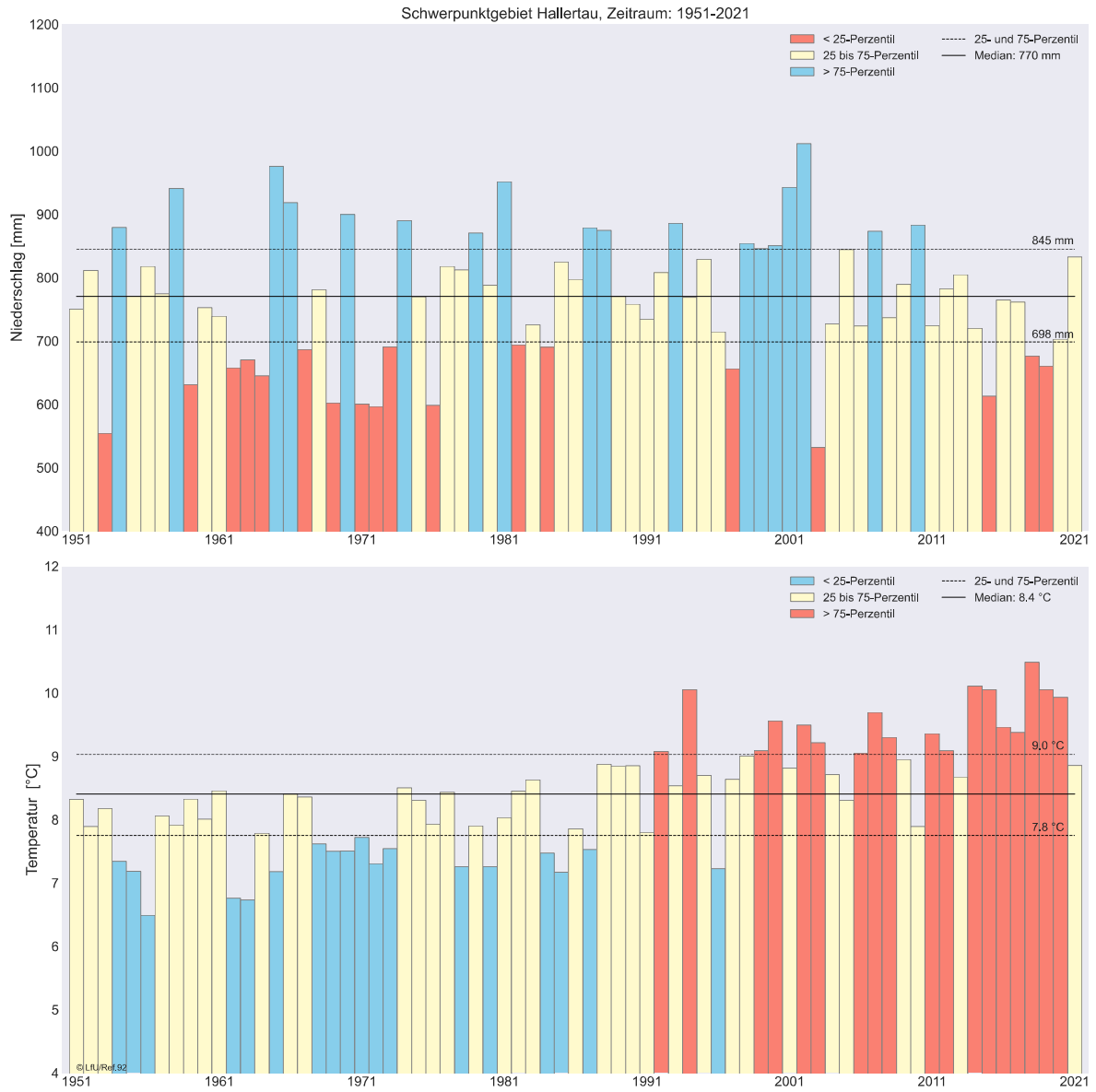
Abb. 3: Mittlere jährliche Niederschlagsmenge (oben) und mittlere Jahresdurchschnittstemperaturen (unten) im Untersuchungsgebiet im Zeitraum 1951-2021 (Temperatur: DWD Stationsdaten; Niederschlag: DWD HYRAS)
