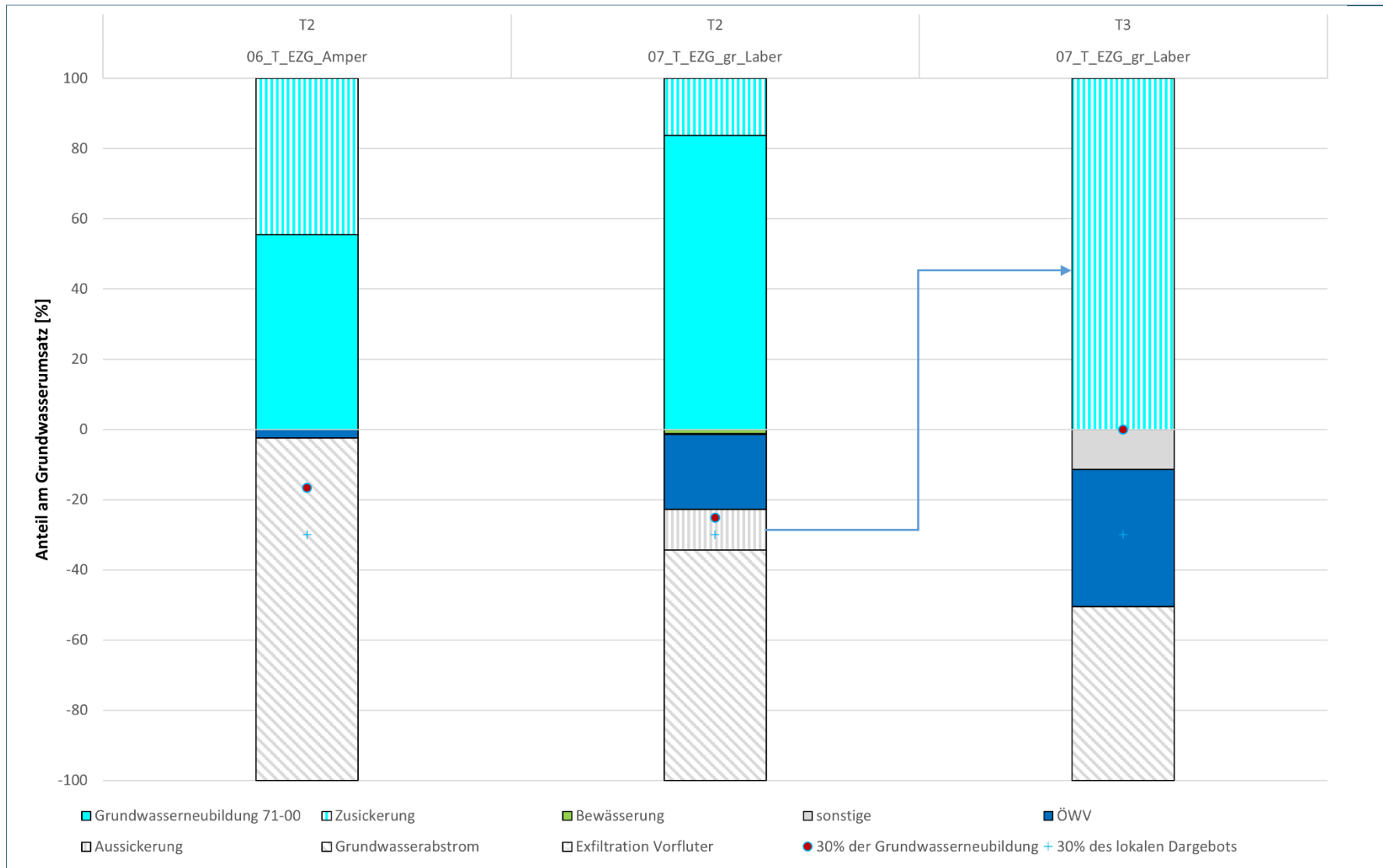
Abb. 41: Grundwasserbilanz der Tertiärterräume 06_T_EZG_Amper und 07_T_EZG_gr_Laber, in prozentualen Anteilen (mittlere Grundwasserneubildung 1971-2000)
