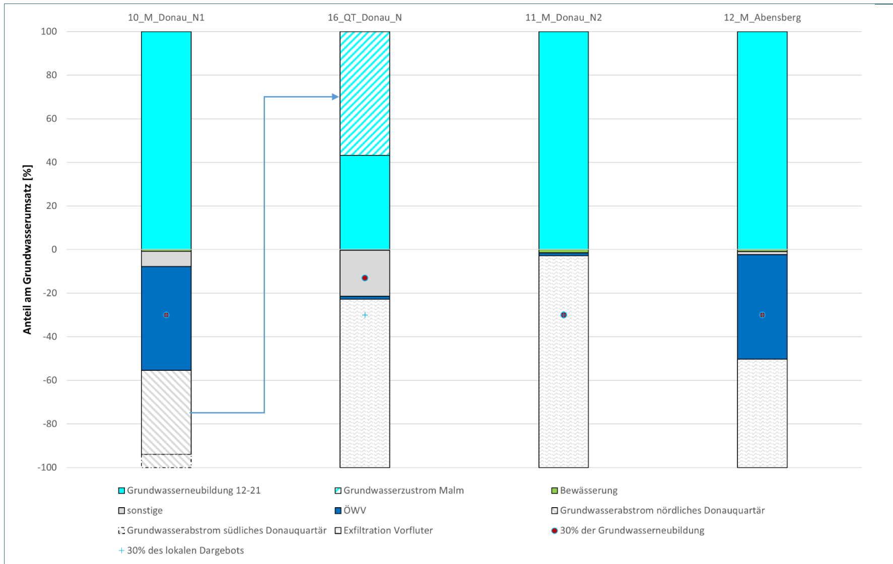
Abb. 45: Grundwasserbilanz der nördlich der Donau gelegenen Teilräume in prozentualen Anteilen (mittlere Grundwasserneubildung 2012-2021)
