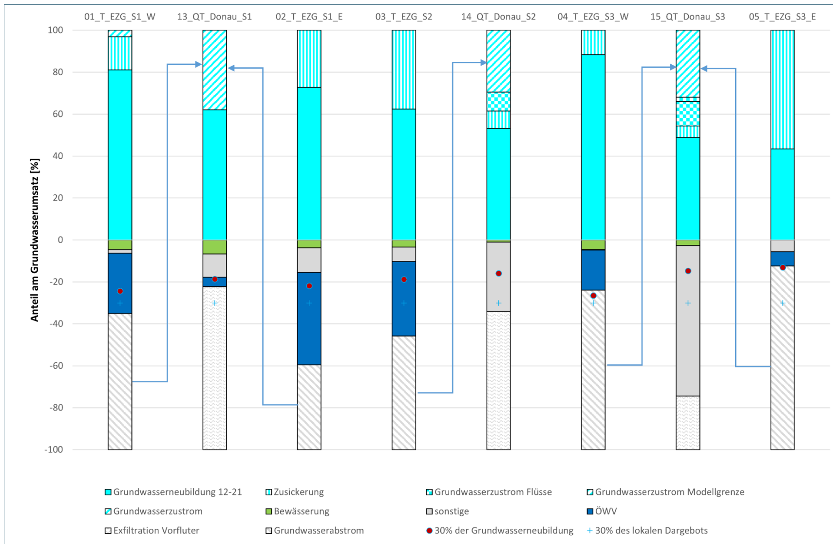
Abb. 43: Grundwasserbilanz der südlich der Donau gelegenen Teilräume in prozentualen Anteilen (mittlere Grundwasserneubildung 2012-2021)
