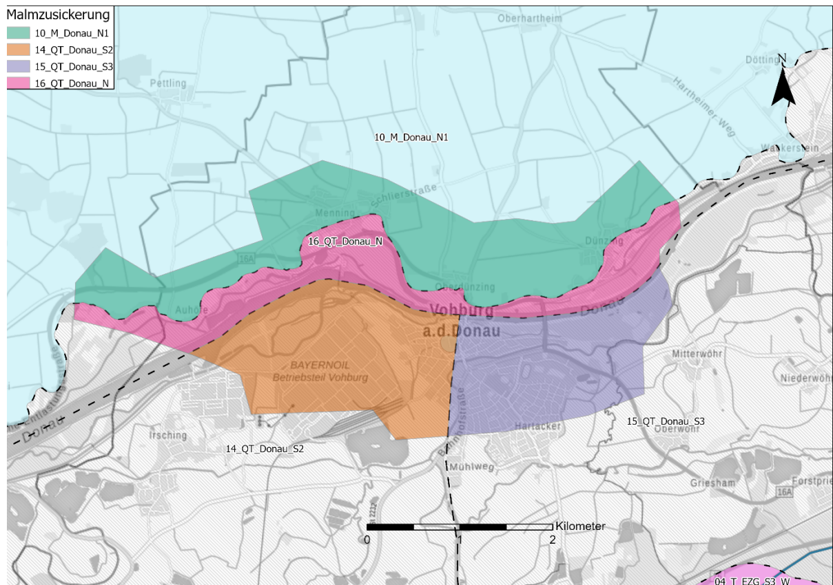
Abb. 33: Bereiche im Quartär, die Zusickerung aus dem Malm erfahren. Grafik abgeändert nach ISAR CONSULT, 1997
