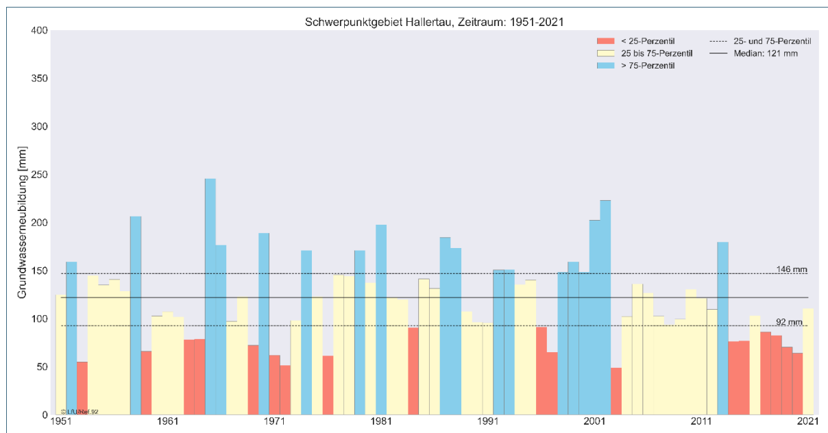
Abb. 28: Jährliche Grundwasserneubildung im Untersuchungsgebiet Hallertau im Zeitraum 1951-2021.
