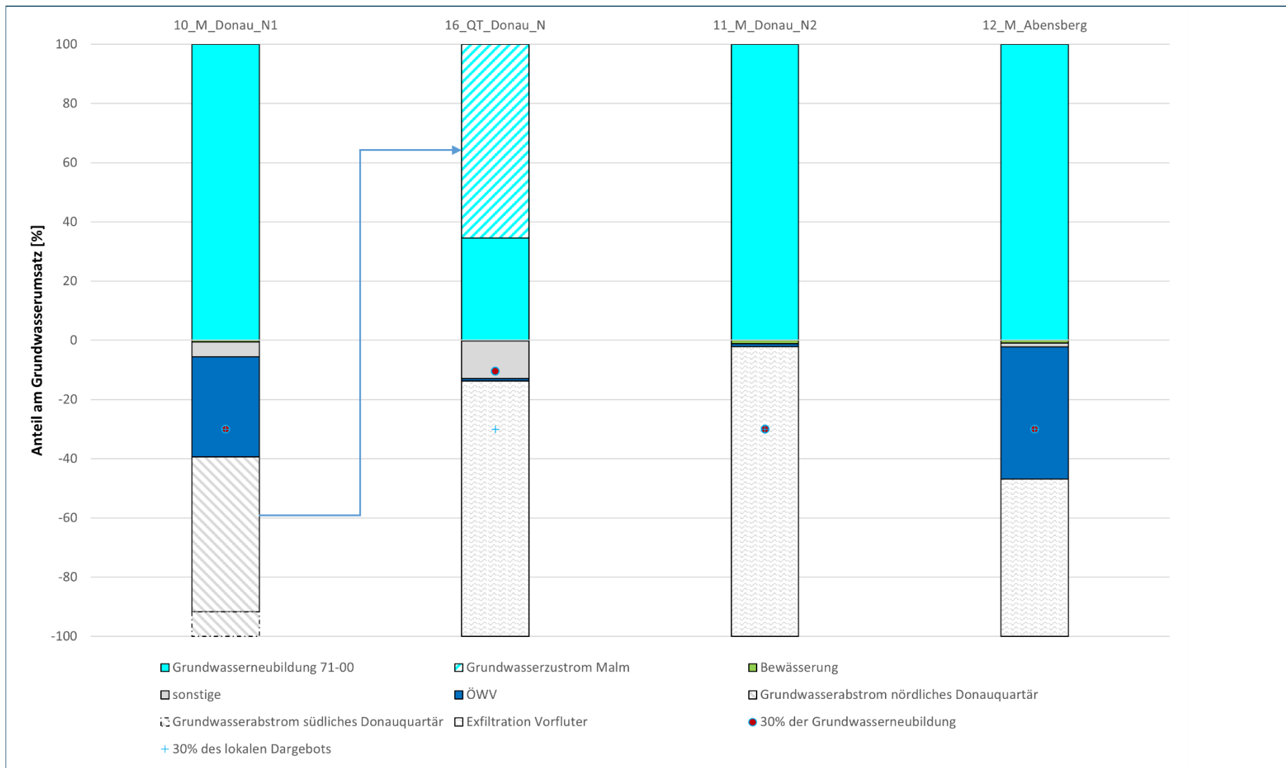
Abb. 37: Grundwasserbilanz der nördlich der Donau gelegenen Teilräume in prozentualen Anteilen (mittlere Grundwasserneubildung 1971-2000)
