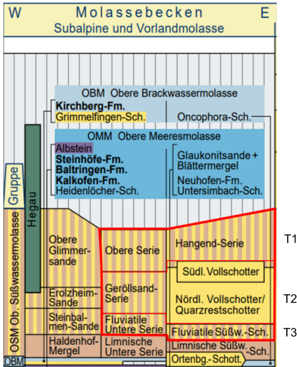
Abb. 8: Ausschnitt Stratigraphische Tabelle von Deutschland 2016, Kennzeichnung der drei im Tertiär berücksichtigten Grundwasserleiter
