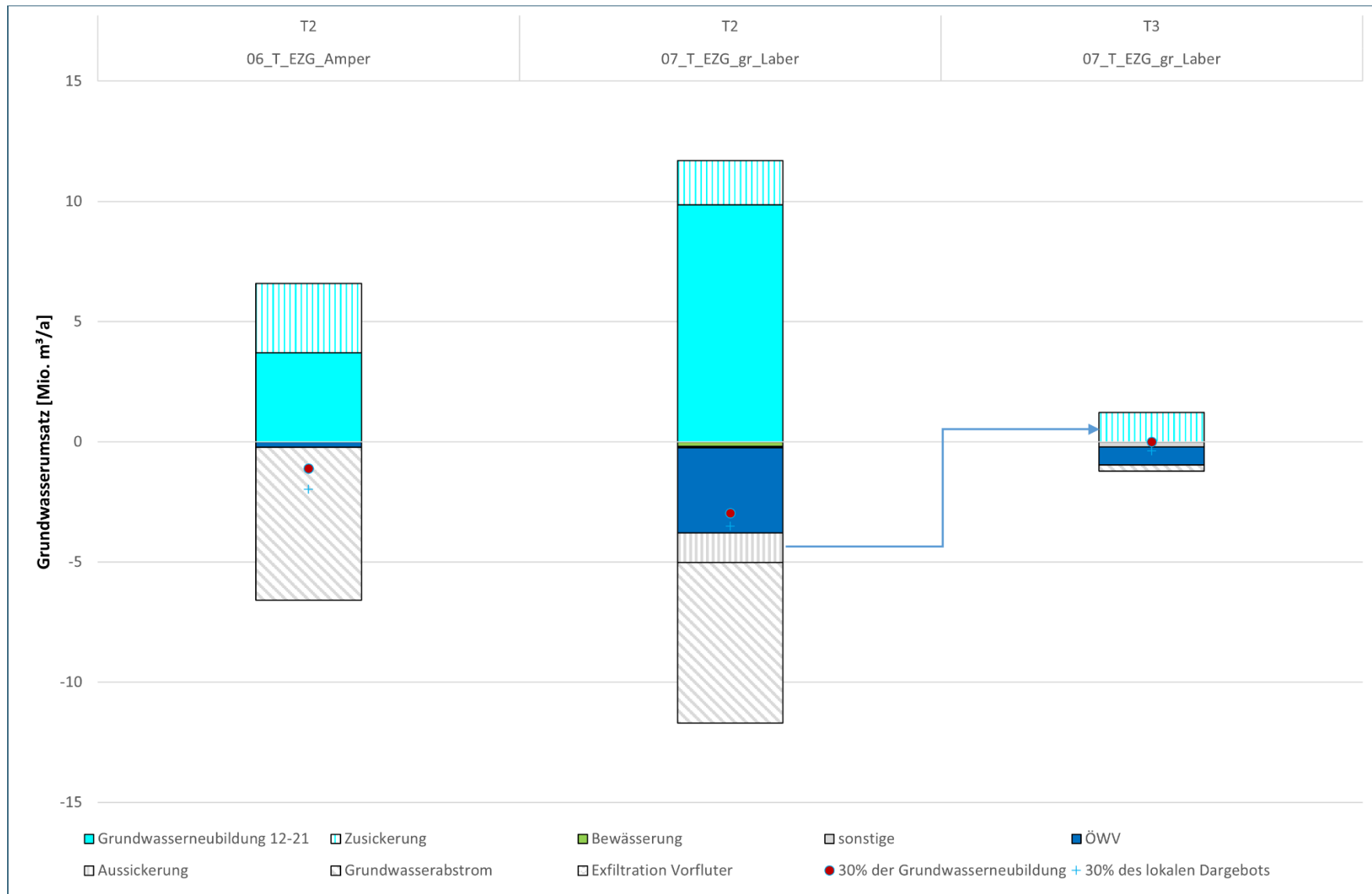
Abb. 48: Grundwasserbilanz der Tertiärterräume 06_T_EZG_Amper und 07_T_EZG_gr_Laber (mittlere Grundwasserneubildung 2012-2021)
