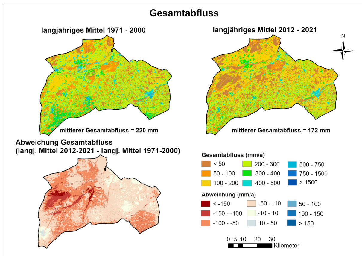
Abb. 26: Gesamtabfluss im Untersuchungsgebiet Hallertau im langjährigen Mittel 1971-2000 und 2012-2021
