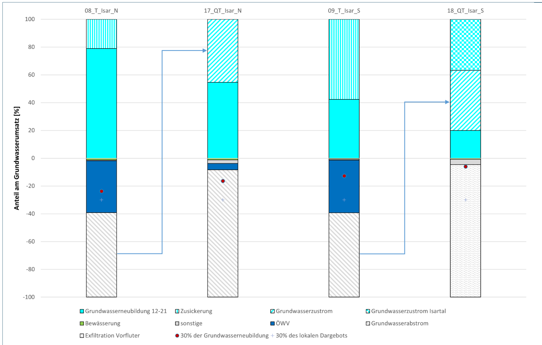
Abb. 47: Grundwasserbilanz des Isarquartärs und der umgebenden Teilräume in prozentualen Anteilen (mittlere Grundwasserneubildung 2012-2021)
