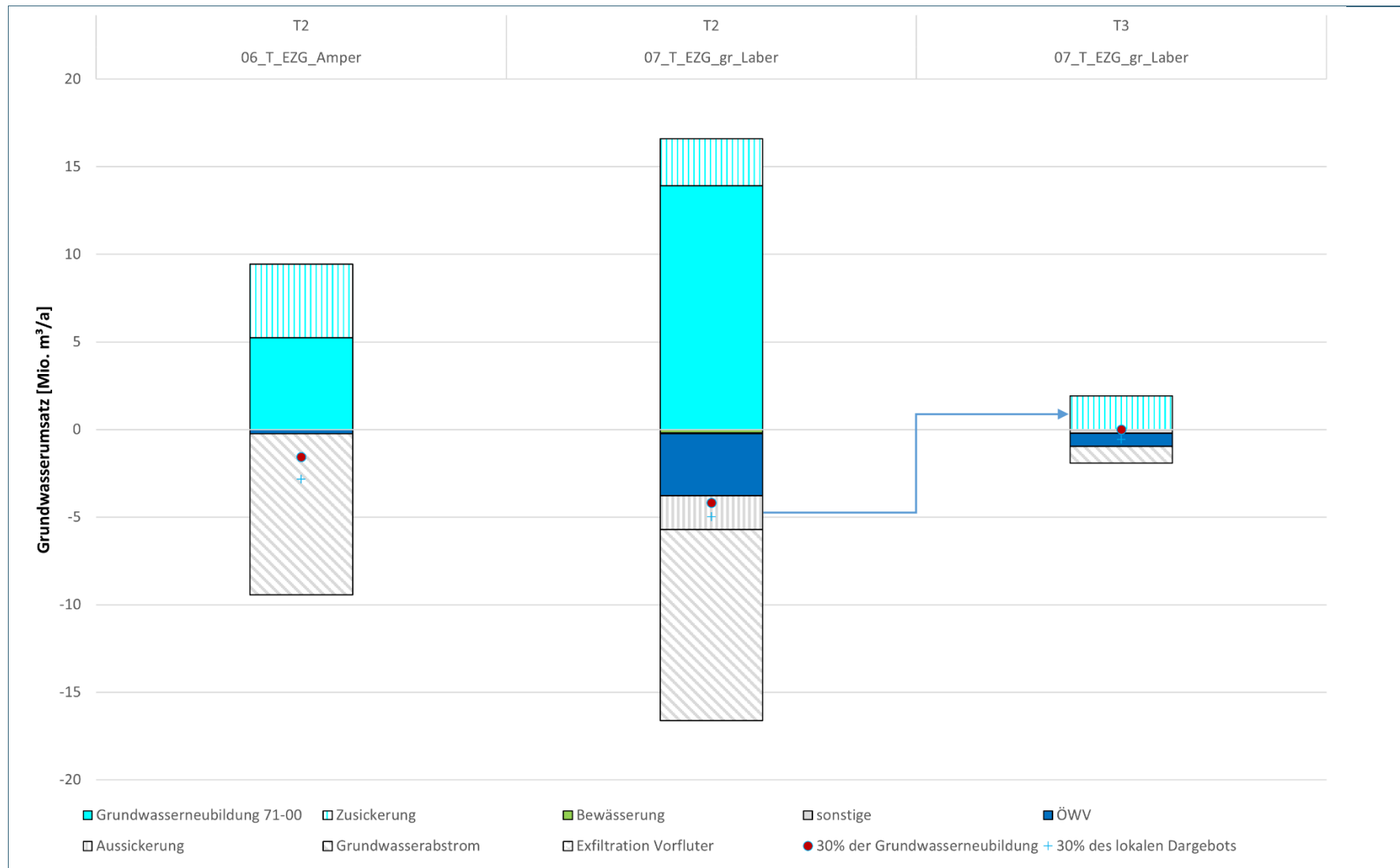
Abb. 40: Grundwasserbilanz der Tertiärteilräume 06_T_EZG_Amper und 07_T_EZG_gr_Laber (mittlere Grundwasserneubildung 1971-2000)
