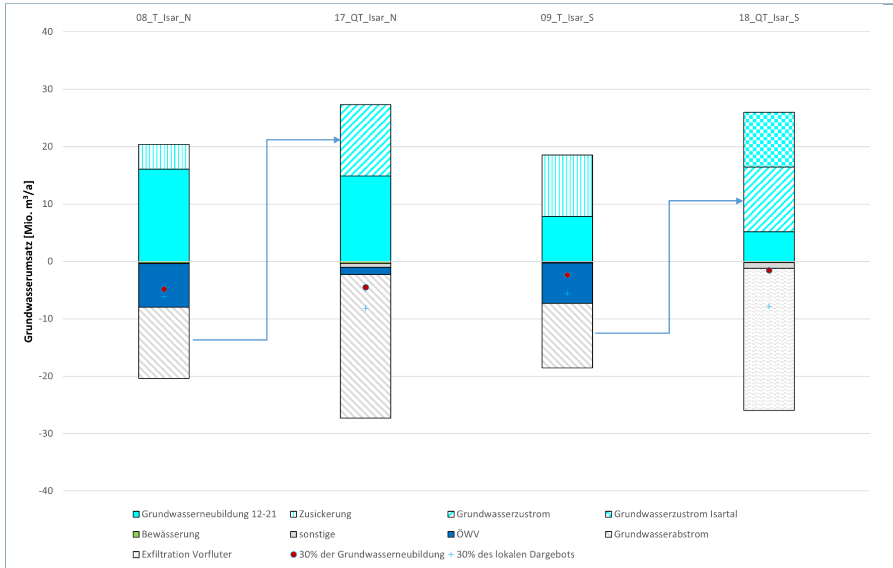
Abb. 46: Grundwasserbilanz des Isarquartärs und der umgebenden Tertiärteilräume (mittlere Grundwasserneubildung 2012-2021)
