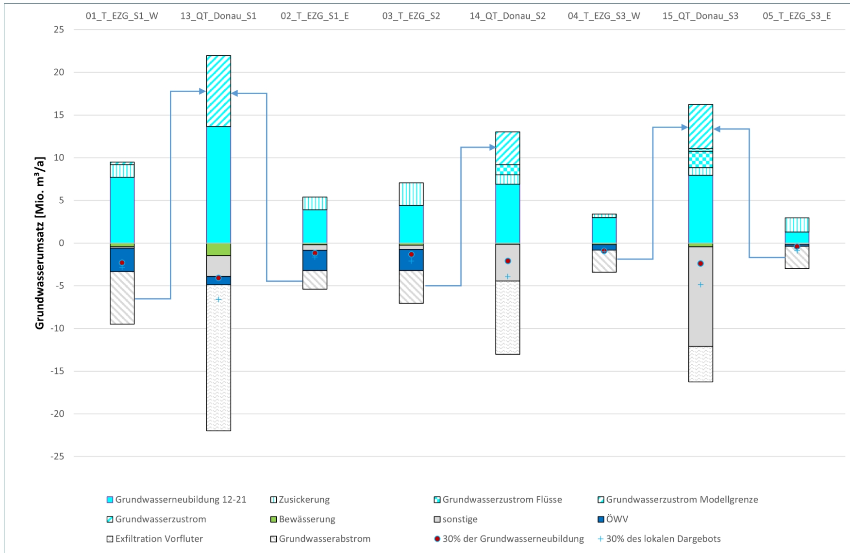
Abb. 42: Grundwasserbilanz der südlich der Donau gelegenen Teilräume (mittlere Grundwasserneubildung 2012-2021)
