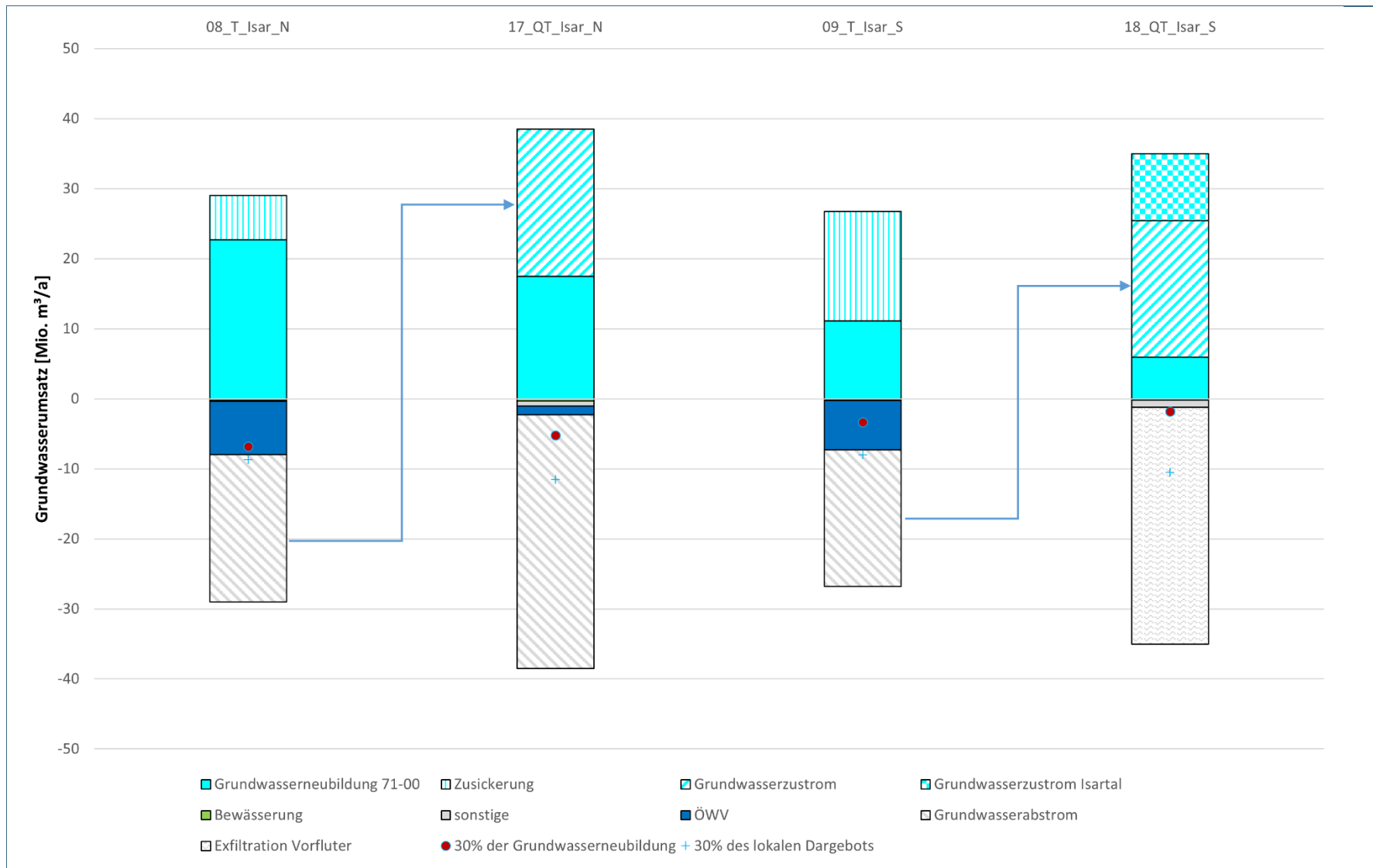
Abb. 38: Grundwasserbilanz des Isarquartärs und der anliegenden tertiären Teilräume (mittlere Grundwasserneubildung 1971-2000)
