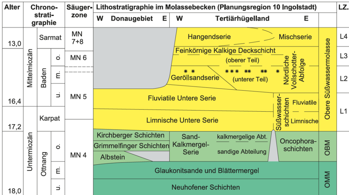
Abb. 4: Schichtenfolge des Tertiärs im Bereich der Planungsregion 10 Ingolstadt (LFU, 2002, HK100)
