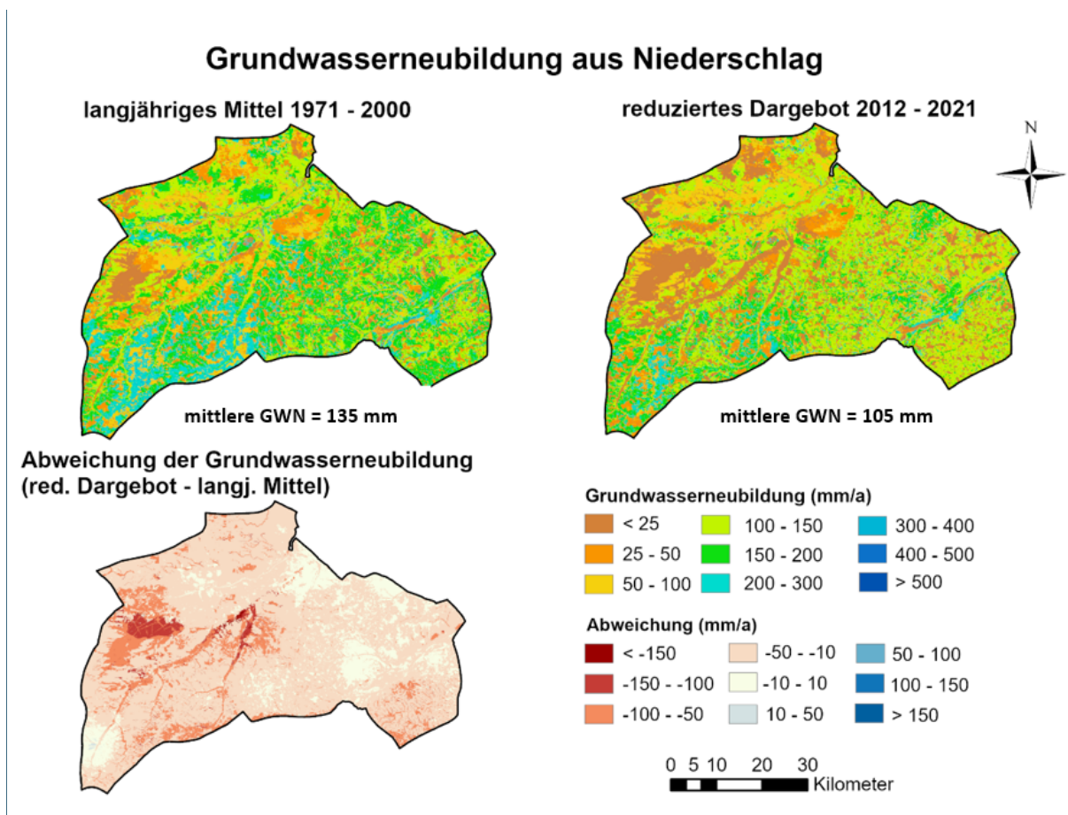
Abb. 27: Grundwasserneubildung aus Niederschlag im Untersuchungsgebiet Hallertau. Gegenüberstellung des langjährigen Mittels und des reduzierten Dargebots
