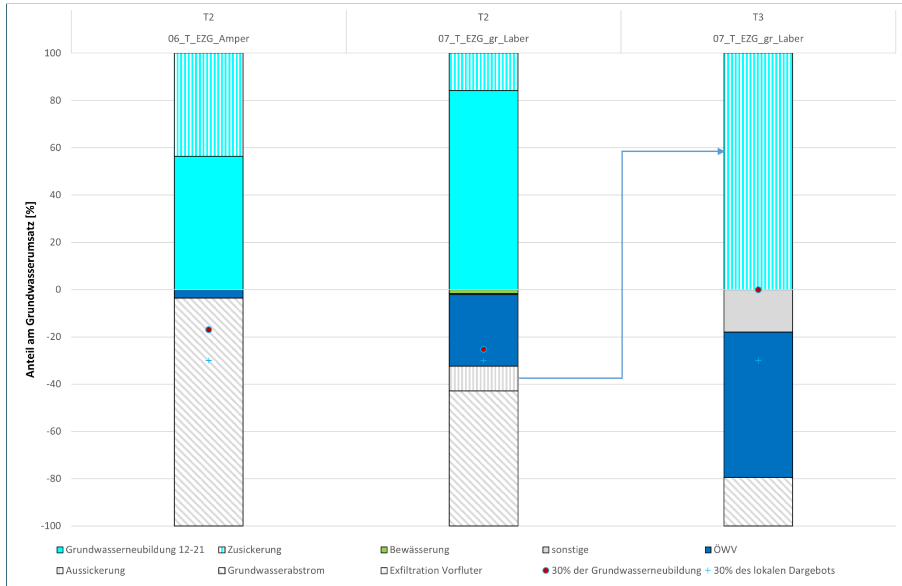
Abb. 49: Grundwasserbilanz der Tertiärteilräume 06_T_EZG_Amper, 07_T_EZG_gr_Laber in prozentualen Anteilen (mittlere Grundwasserneubildung 2012-2021)
