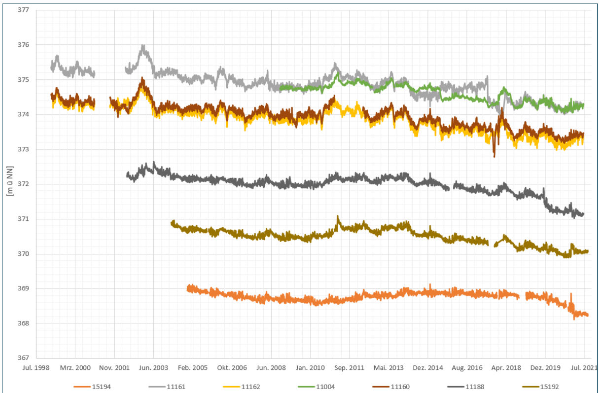
Abb. 15: Ausgewählte Grundwasserganglinien im Bereich des überdeckten Malm
