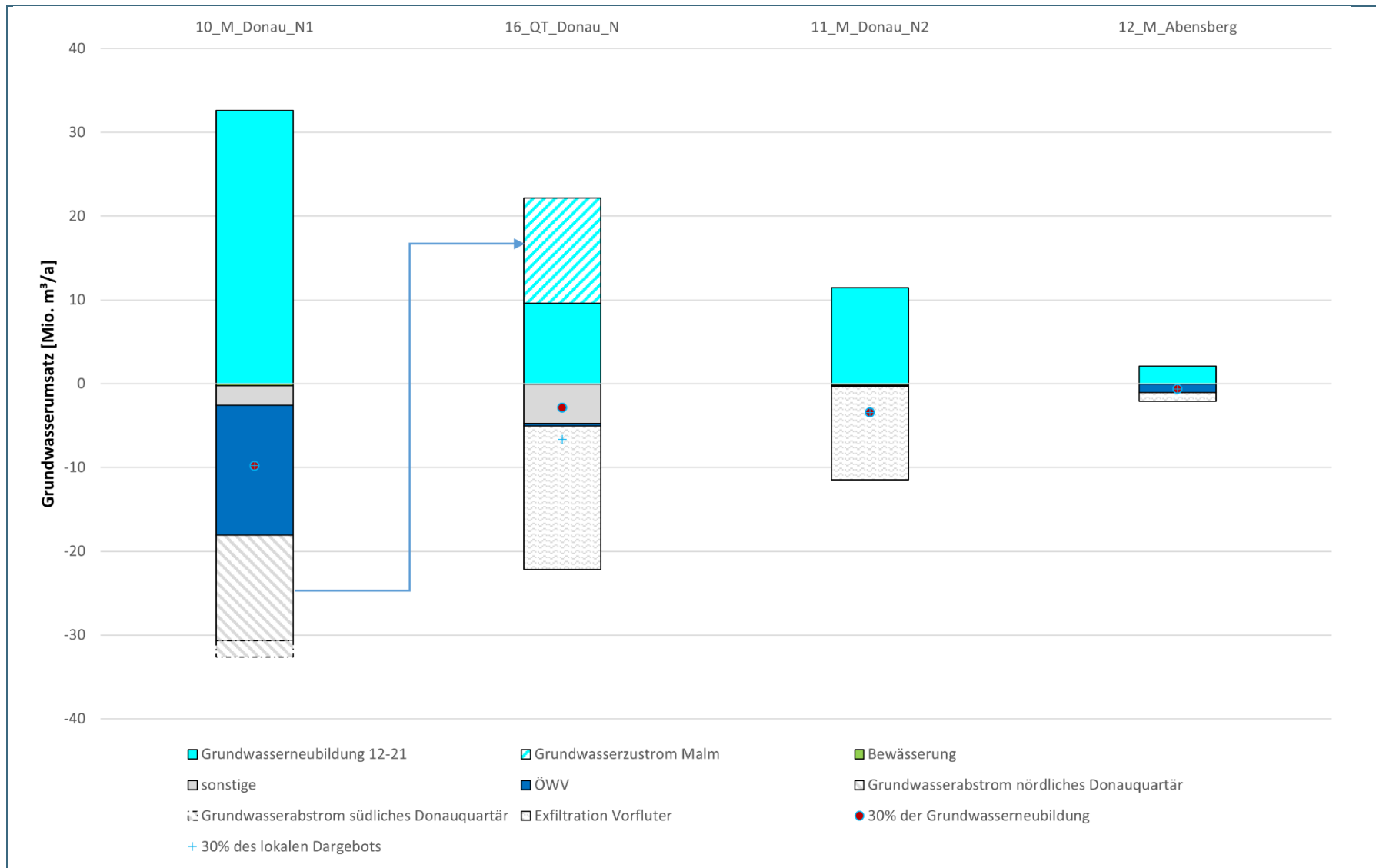
Abb. 44: Grundwasserbilanz der nördlich der Donau gelegenen Teilräume (mittlere Grundwasserneubildung 2012-2021)
