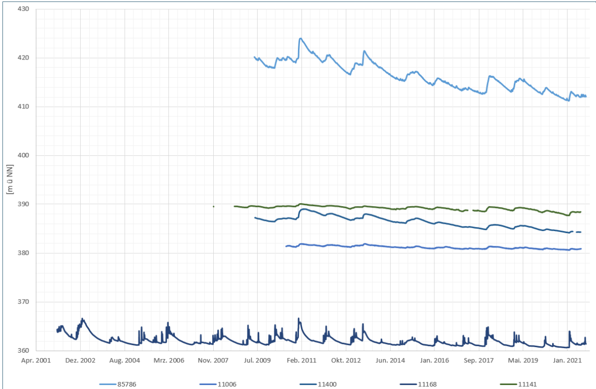
Abb. 14: Ausgewählte Grundwasserganglinien im Bereich des offenen Malm
