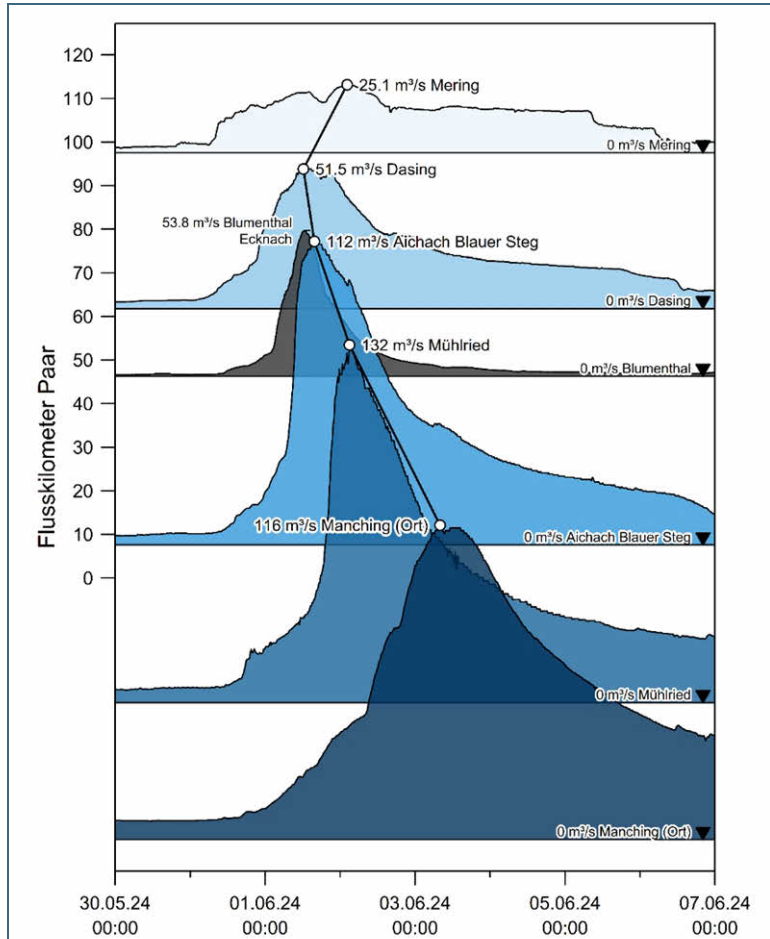
Abb. 27: Hochwasserwellenplan für die Paar (vorläufige Werte, Stand 31. März 2025)
