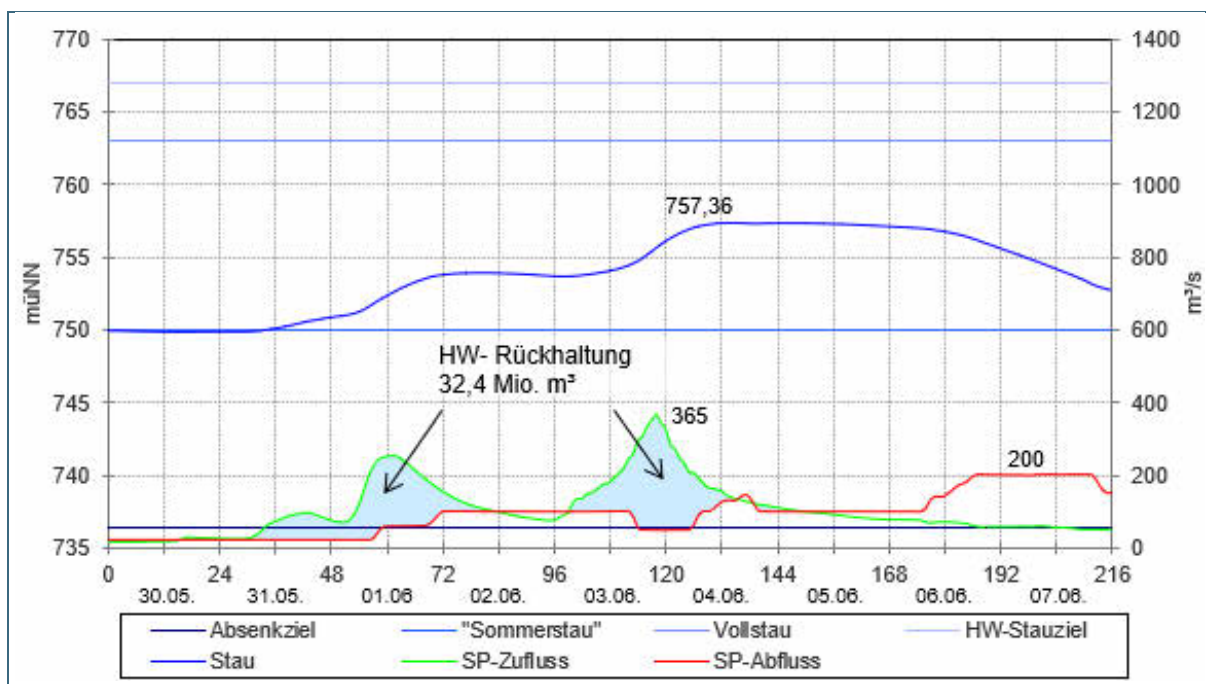
Abb. 35: Hochwasserbetrieb Sylvensteinspeicher (Quelle: WWA Weilheim)
