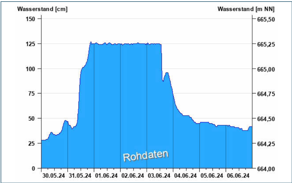
Abb. 89: Am Pegel gemessener Wasserstand in der Westlichen Günz unmittelbar unterhalb des HRB Eldern (Quelle: HND, Rohdaten)
