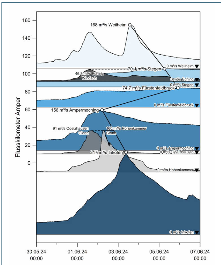
Abb. 29: Hochwasserwellenplan für die Amper/ Amper (vorläufige Werte, Stand 31. März 2025)
