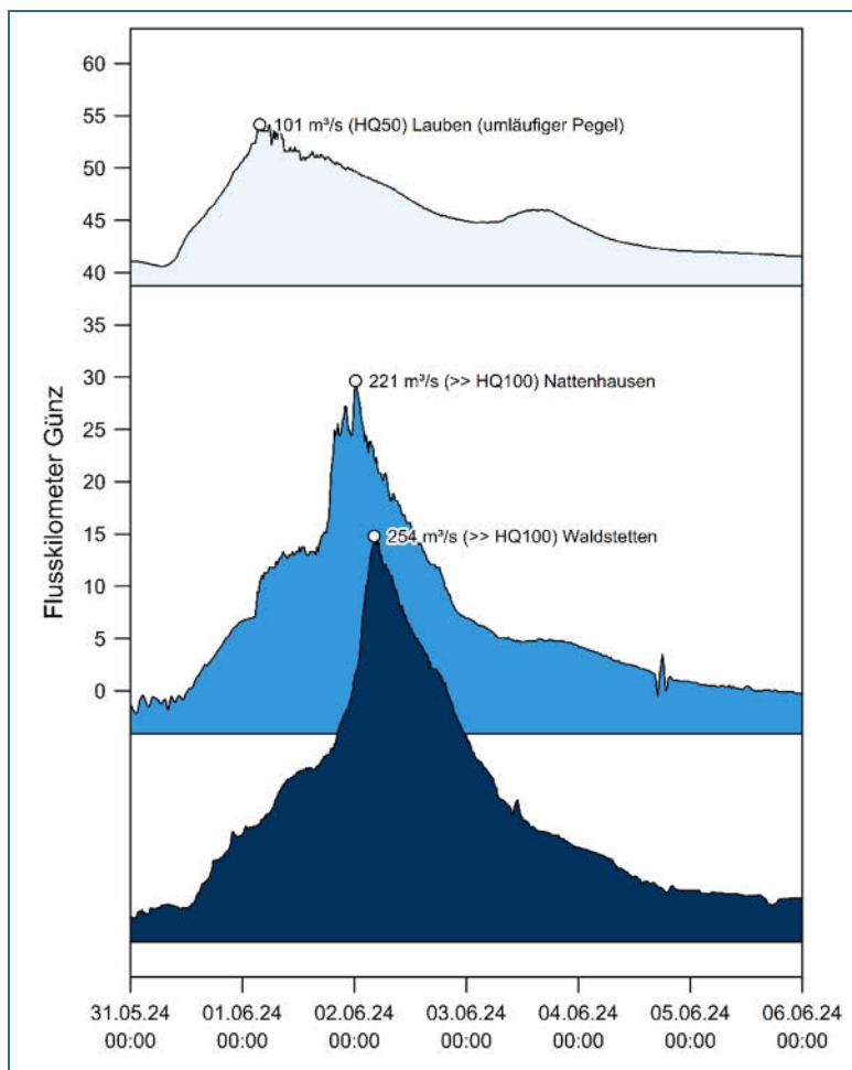
Abb. 24: Hochwasserwellenplan der Günz ab dem Zusammenfluss der westlichen und östlichen Günz (vorläufige Werte, Stand 31. März 2025); erhöhte Unsicherheit bei der Abflussbestimmung am Pegel Lauben/Günz durch Umläufigkeit im Hochwasserfall
