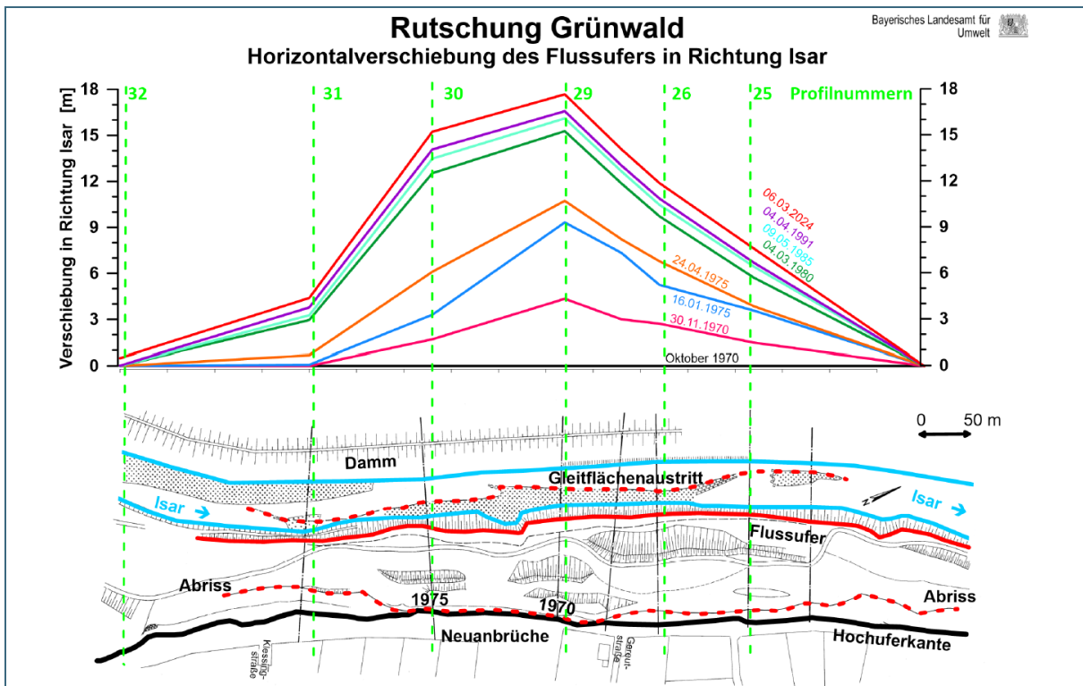
Abb. 67: Verschiebungen der Rutschmassen am Isarufer unterhalb Grünwald
