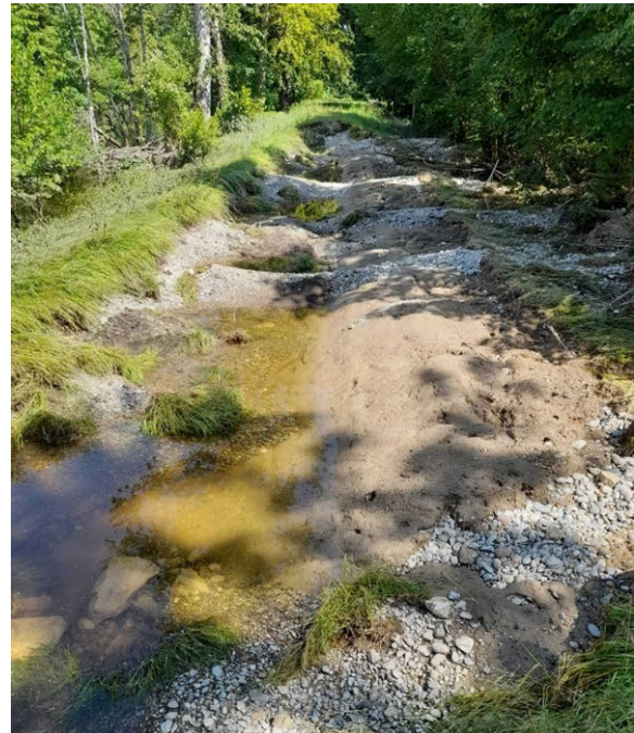
Abb. 44: erodierte Deichstrecke bei Steinheim (Foto: WWA Donauwörth)
