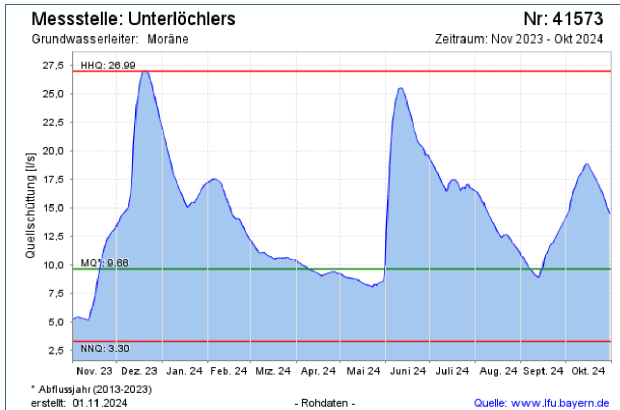
Abb. 78: Quellmessstelle Unterlöchlers (Gemeinde Rettenbach am Auerberg, Landkreis Unterallgäu)
