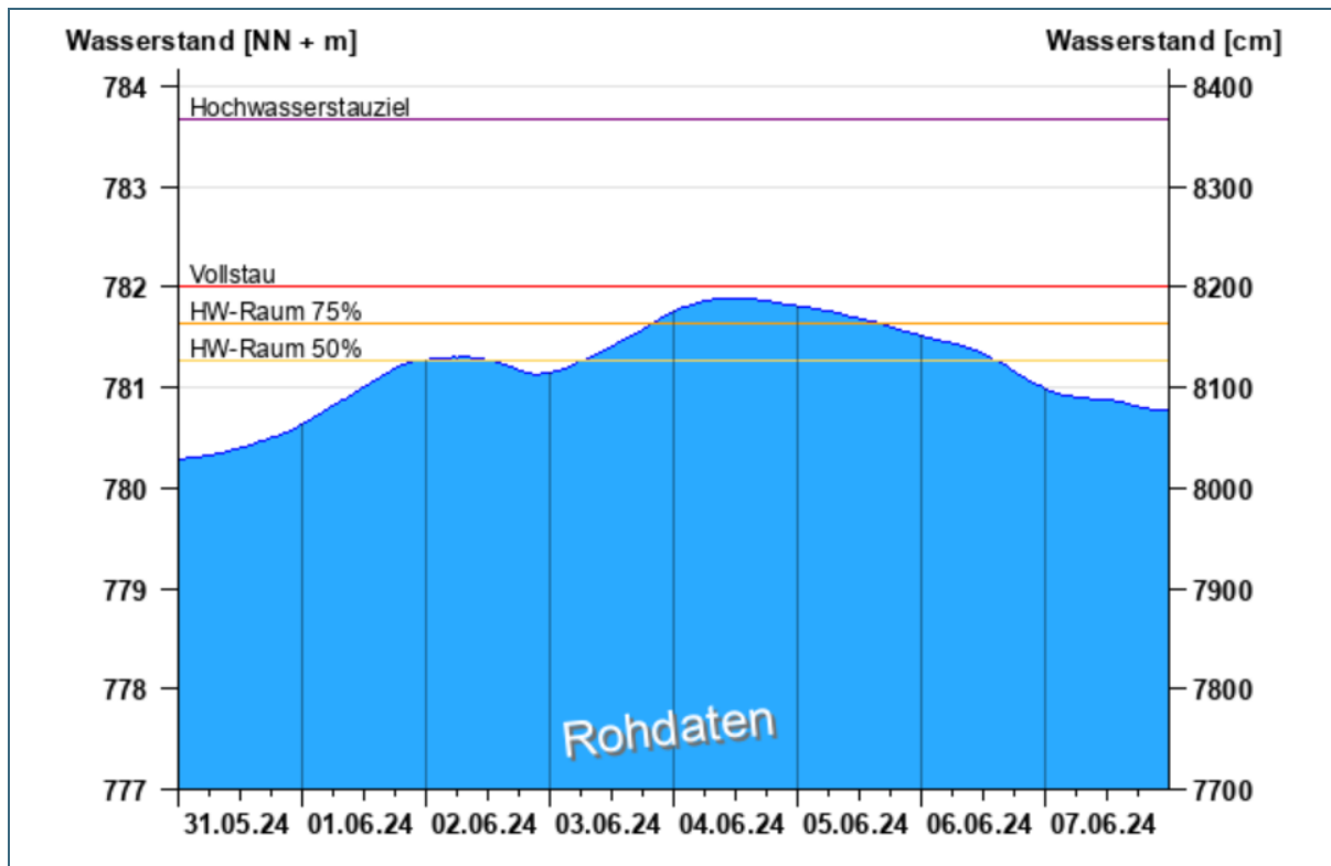
Abb. 41: Seepegel Forggensee (Quelle: HND, Rohdaten)
