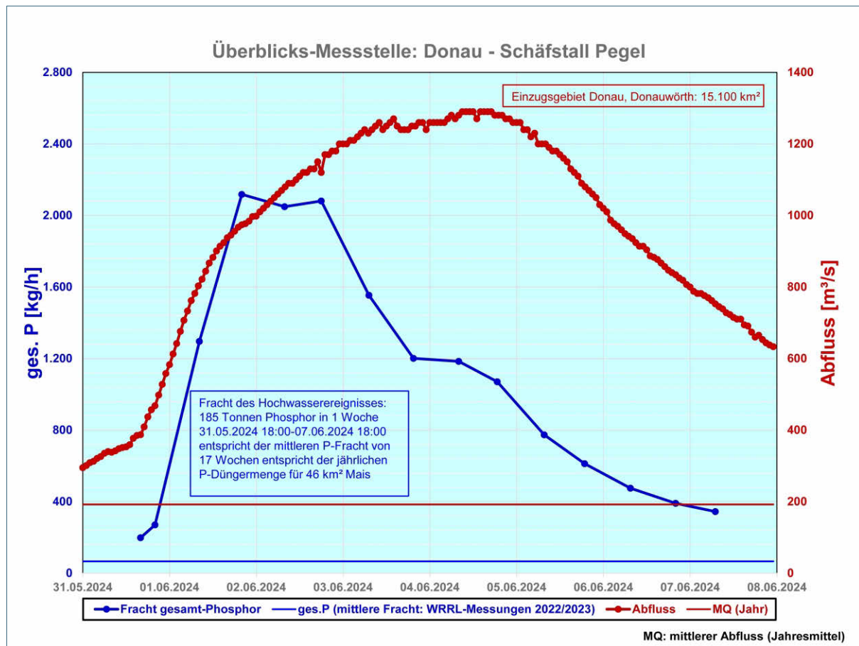
Abb. 79: Zusammenhang zwischen der Fracht Phosphor gesamt und dem Abfluss an der Donau am Pegel Schäfstall vom 31. Mai bis 7. Juni 2024 (Quelle: WWA Donauwörth)
