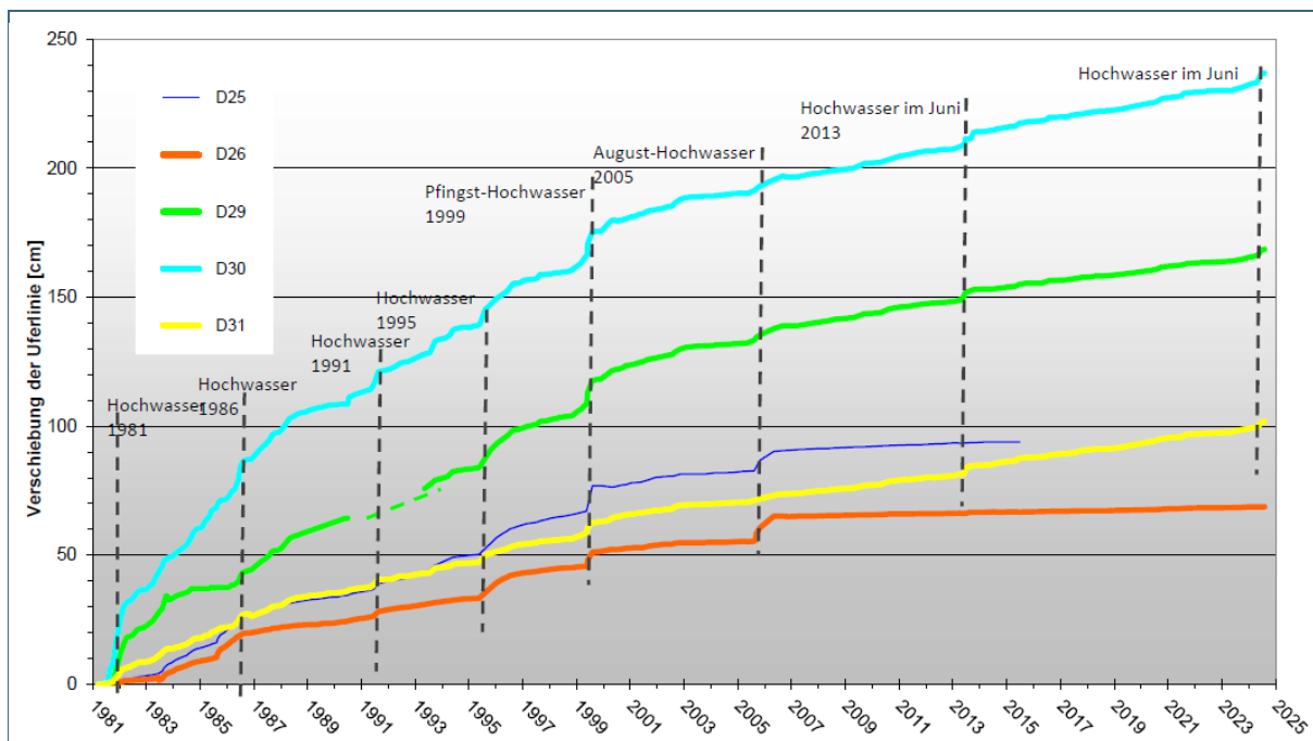
Abb. 68: Verschiebungen am Isarufer über den Messzeitraum mit eingetragenen Hochwasserereignissen
