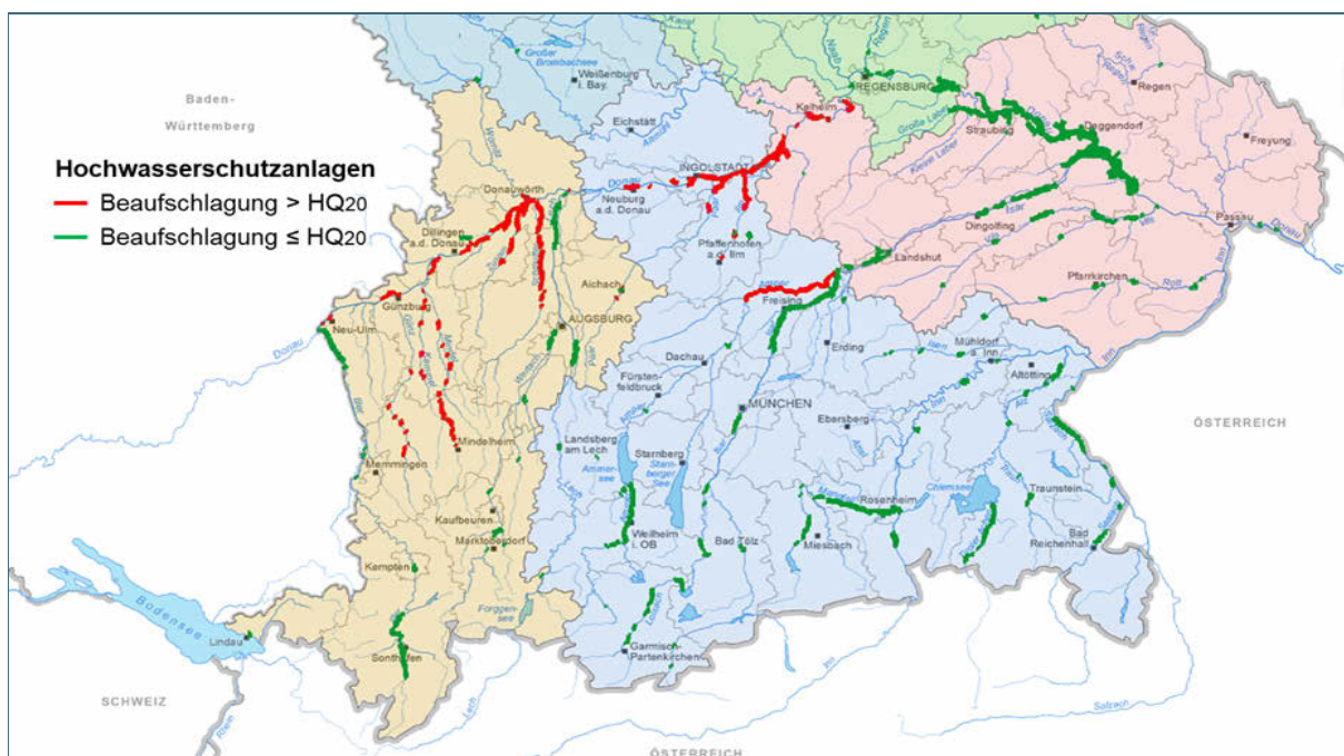
Abb. 42: HWS-Anlagen an Gewässern erster und zweiter Ordnung an der Donau und im südlichen Einzugsgebiet (Hintergrundkarte © Geobasisdaten: Bayerische Vermessungsverwaltung 2024)
