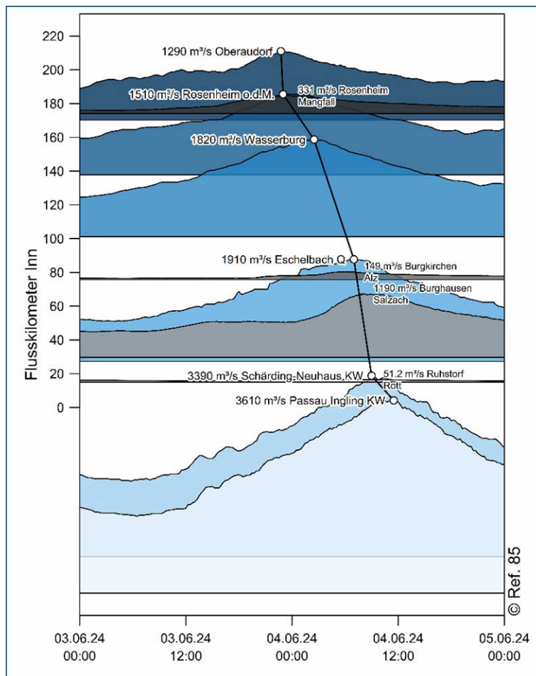
Abb. 31: Hochwasserwellenplan für den Inn mit den Zuflüssen aus Mangfall, Alz, Salzach und Rott (vorläufige Werte, Stand 31. März 2025)
