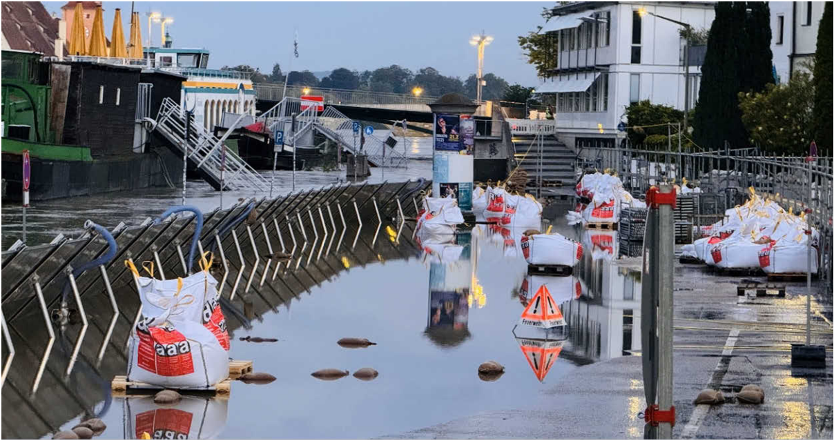
Abb. 47: Mobiles Hochwasserschutzsystem der Stadt Regensburg im Bereich Unterer Wöhrd; punktuelle Auflast gegen steigenden Auftriebsdruck (Foto: WWA Regensburg)
