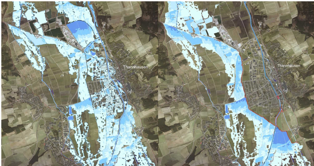
Abb. 95: Hydraulische Berechnung eines 100-jährlichen Hochwassers der Mindel ohne (links) und mit (rechts) Hochwasserschutzmaßnahmen (Quelle: WWA Donauwörth)
