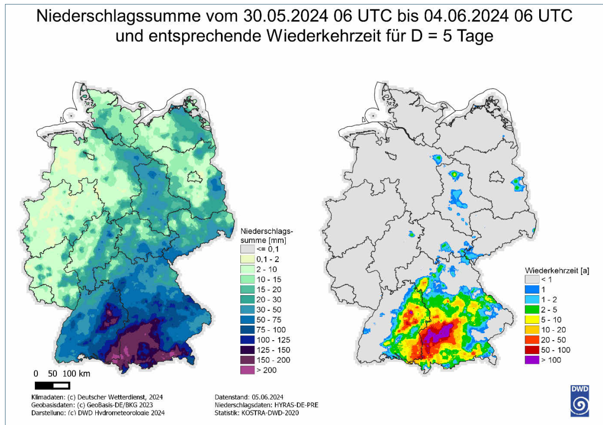
Abb. 12: 5-Tages-Niederschlagssumme vom 30. Mai bis 4. Juni 2024 06:00 Uhr UTC und die entsprechende Wiederkehrzeit gemäß KOSTRA-DWD-2020 (Quelle: DWD, Hydrometeorologie).
