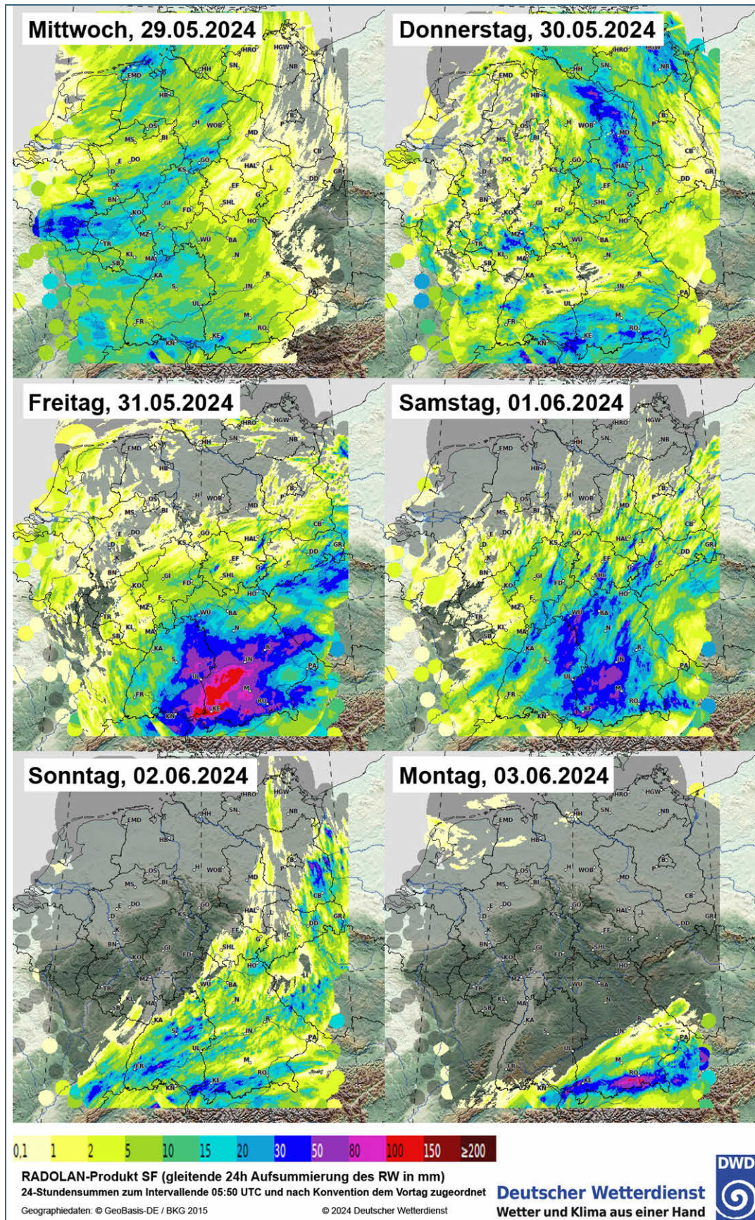
Abb. 6: Tagesniederschlagssummen aus der Radarerfassung (DWD-RADOLAN-Produkt SF) für den Zeitraum 29. Mai bis 3. Juni 2024 (24-Stundensummen zum Intervallende 05:50 UTC) (Quelle: DWD, Zusammenstellung: LfU).
