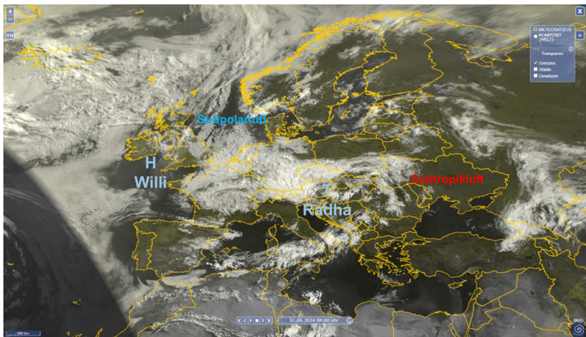
Abb. 3: Satellitenbild Deutscher Wetterdienst (DWD) vom 1. Juni 2024 um 08:00 Uhr (Quelle: Internet DWD) mit Ergänzungen der maßgeblichen Hoch- und Tiefdruckgebiete sowie der Luftmassentypisierungen (LfU).
