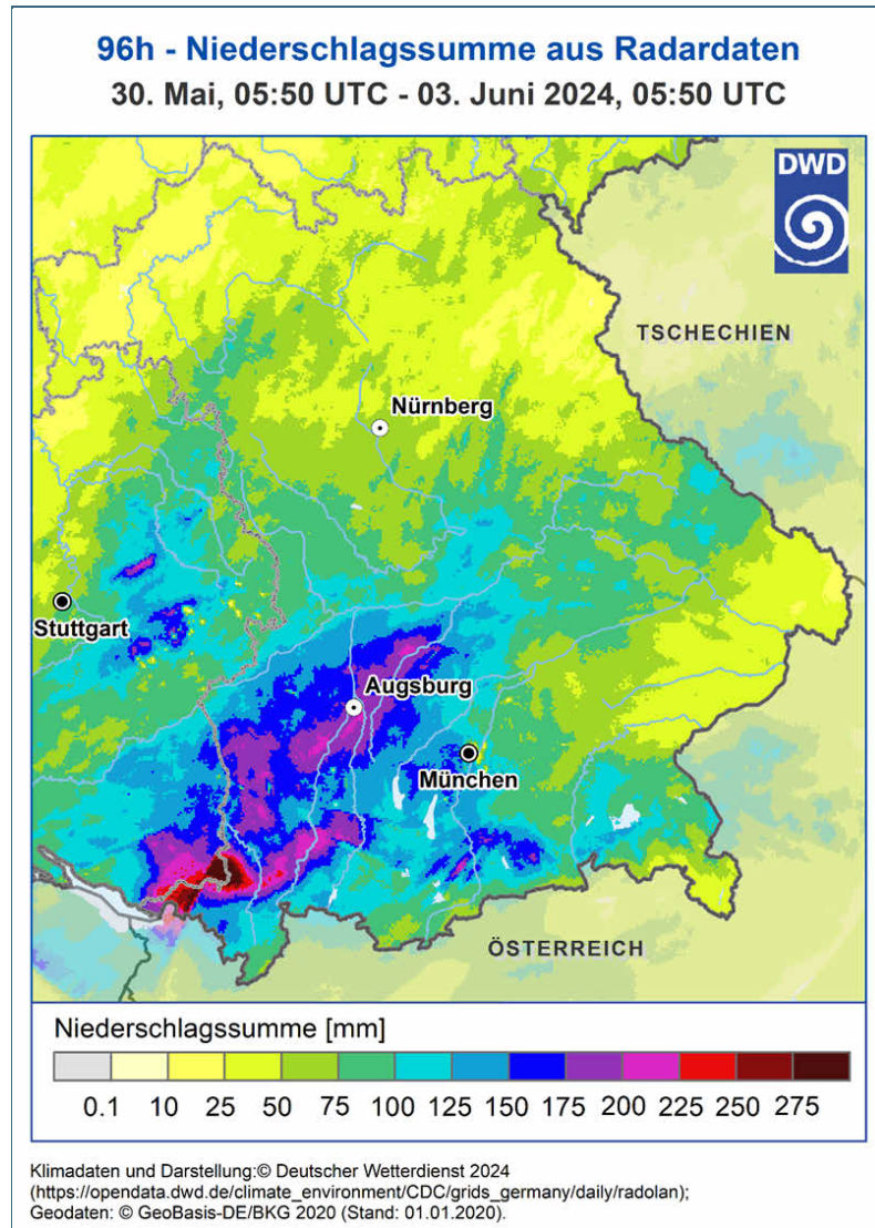
Abb. 13: 96-Stunden-Radarniederschlags- summe vom 30. Mai bis 3. Juni 2024 05:50 Uhr UTC (Quelle: DWD, Hydrometeorologie).
