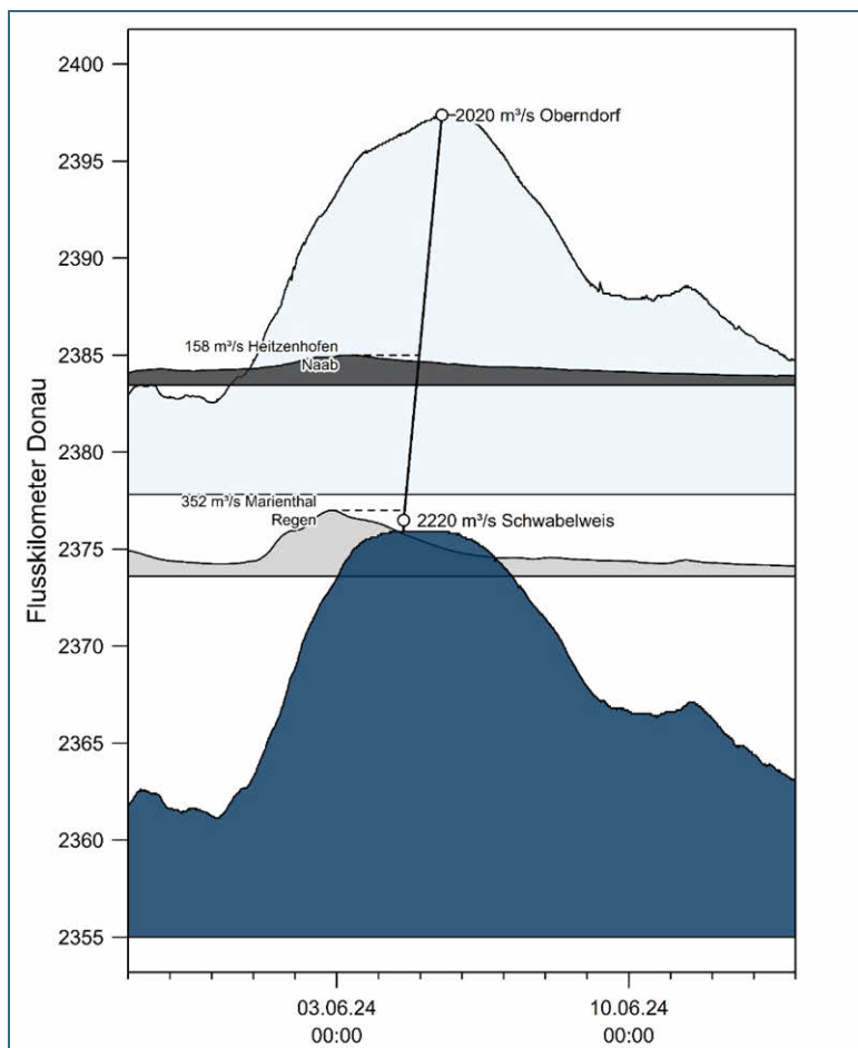
Abb. 26: Wellenüberlagerung in Regensburg (Zusammenfluss von Donau, Naab und Regen) (vorläufige Werte, Stand 31. März 2025)
