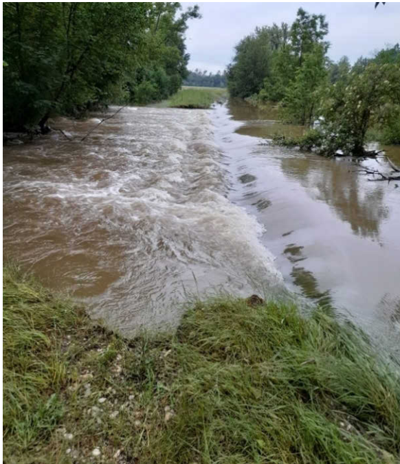
Abb. 43: Überströmung des Sommerdeichs bei Steinheim (Foto: WWA Donauwörth)
