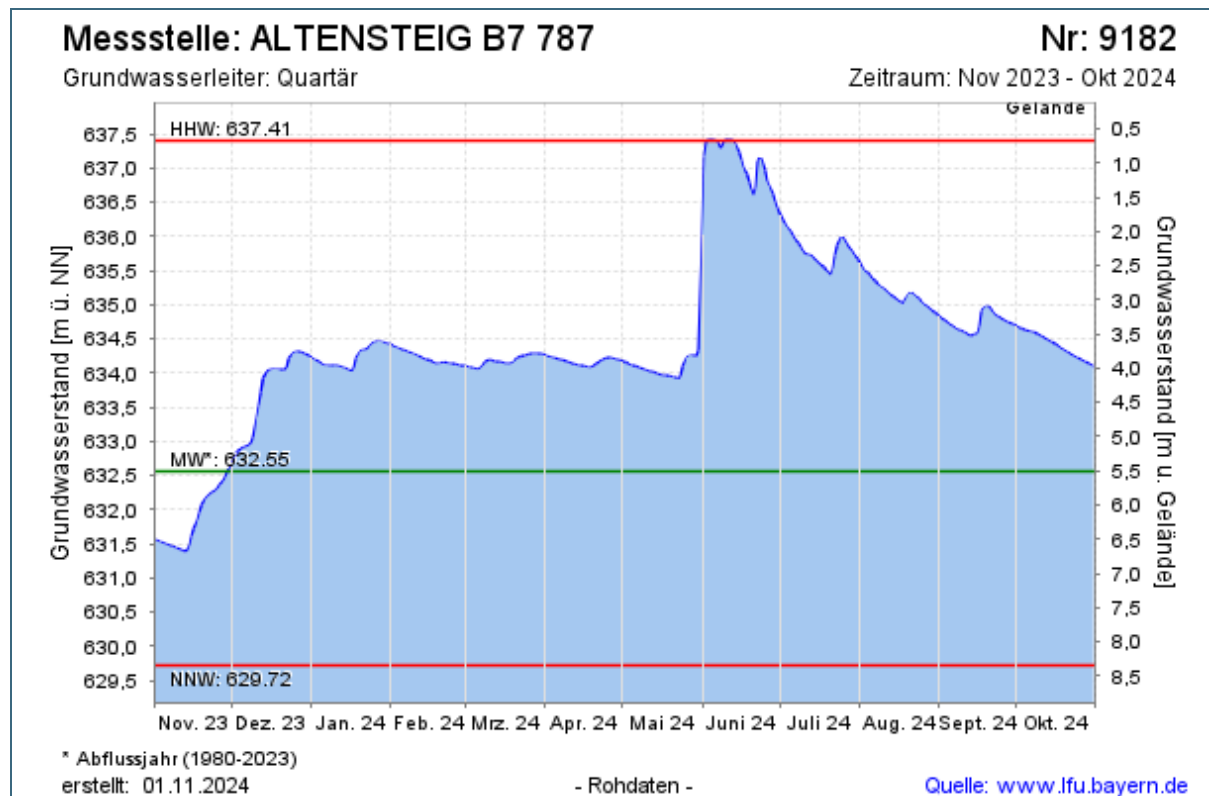
Abb. 76: Grundwassermessstelle ALTENSTEIG B7 787 (Gemeinde Dirlewang, Landkreis Unterallgäu)
