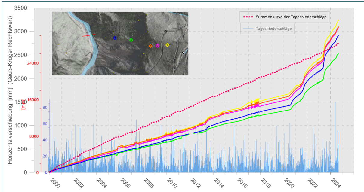
Abb. 66: Verschiebungsbeträge ausgewählter Messpunkte, Tagesniederschläge, sowie Summenkurve der Tagesniederschläge aufgetragen über den Beobachtungszeitraum an der Rutschung Brechries
