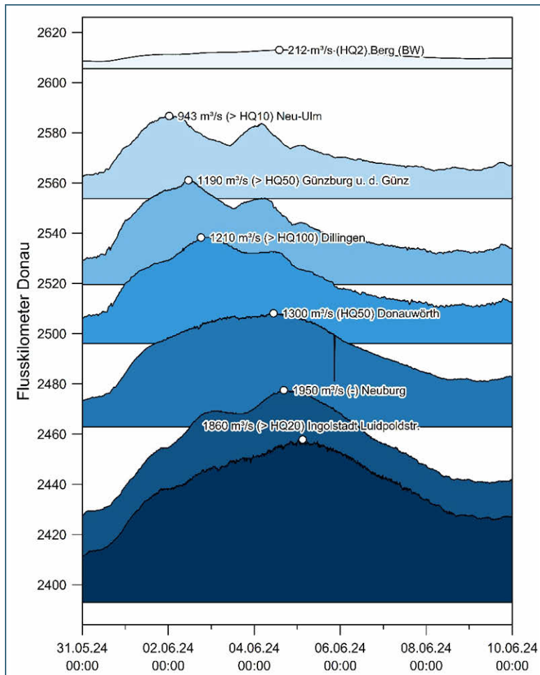
Abb. 23: Hochwasserwellenplan des Donauabschnitts zwischen Berg (Baden-Württemberg) und Ingolstadt (vorläufige Werte, Stand 31. März 2025). Für Neuburg/Donau liegt nur eine provisorische Abflussermittlung und keine HQ-Statistik vor.
