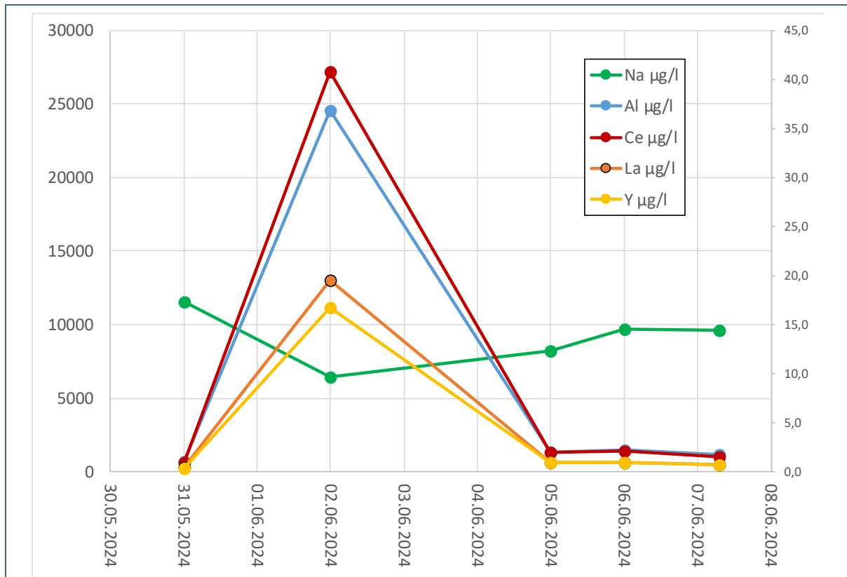
Abb. 80: Konzentrationen der Elemente Aluminium, Cer, Lanthan, Yttrium und Natrium in den aufgeschlossenen Wasserproben an der Messstelle Donau/Schäfstall während der Hochwasserwelle in µg/l.
