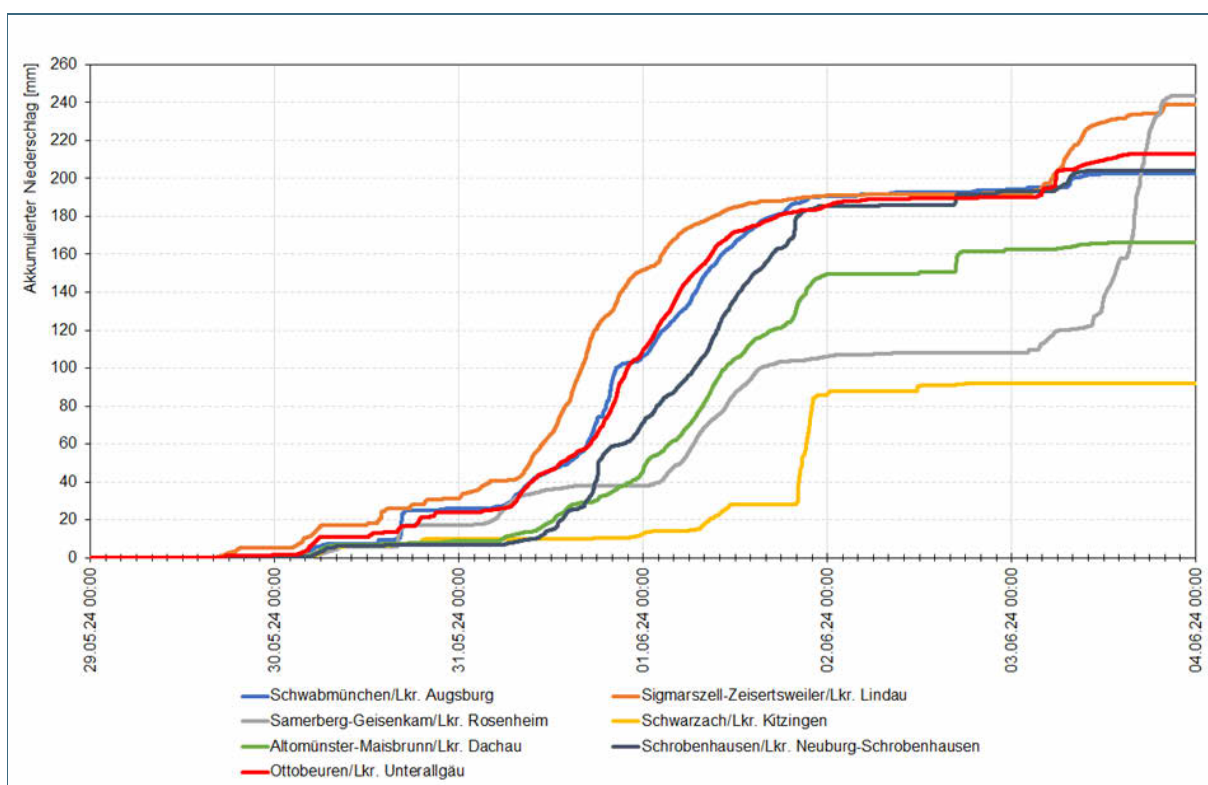
Abb. 7: Niederschlagssummenkurven ausgewählter Niederschlagsstationen
