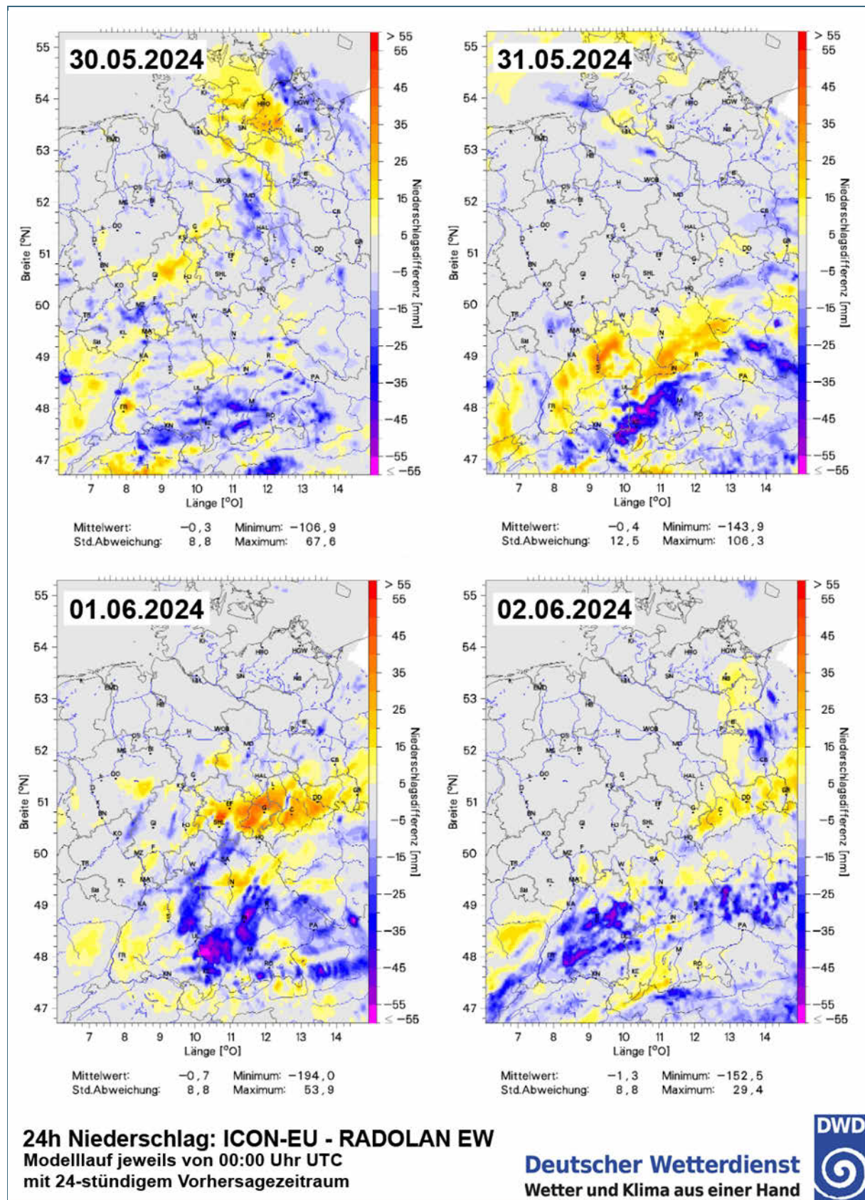
Abb. 14: Differenz zwischen erfasstem Radarniederschlag (RADOLAN-Produkt EW) und der 24-Stunden-Niederschlagssumme des DWD-Modells ICON-EU (0 UTC-Läufe) für 30. Mai, 31. Mai, 1. Juni und 2. Juni 2024 (Quelle: DWD, Zusammenstellung: LFU)
