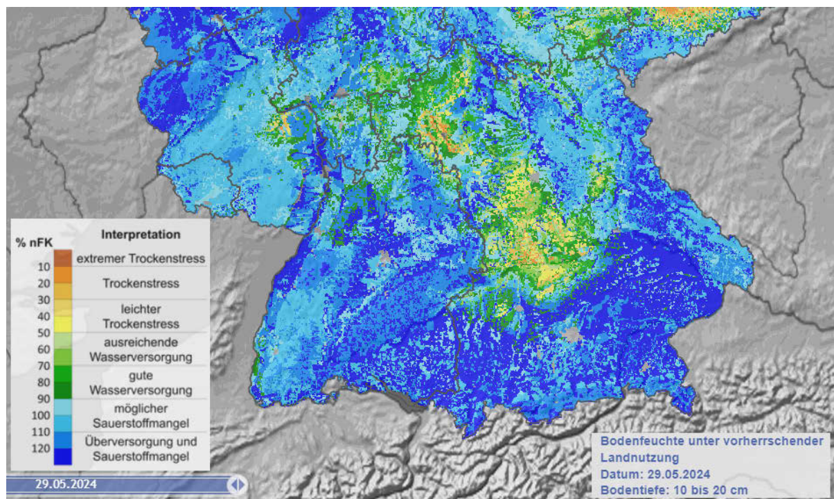
Abb. 4: Bodenfeuchteviewer des DWD vom 29. Mai 2024: insbesondere für Südbayern sehr hohe Bodenfeuchten, Bodentiefe 10 bis 20 cm (Quelle: DWD).
