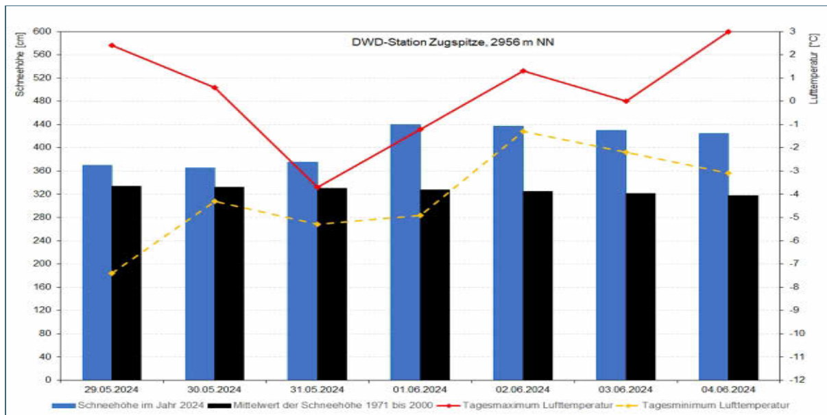
Abb. 5: Schnee- und Lufttemperaturmessungen der DWD-Station Zugspitze (Datenbasis: DWD, Datenaufbereitung: LfU).
