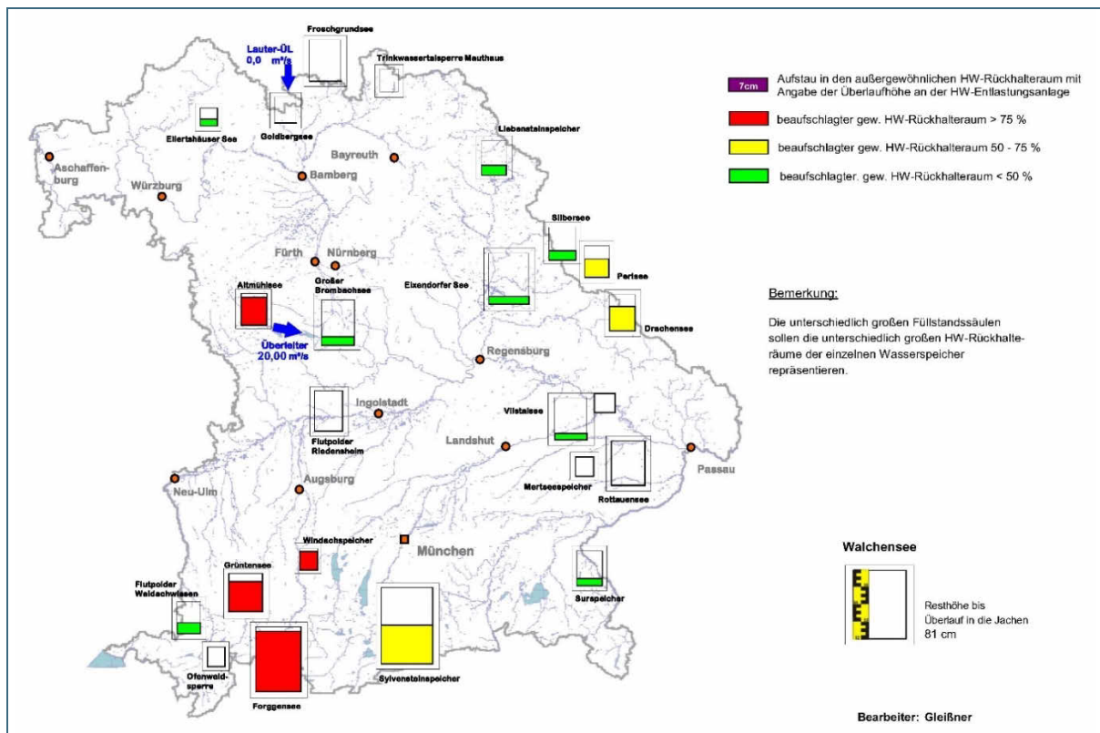
Abb. 34: Staatliche WSP mit Hochwasserschutzfunktion und der nicht-staatliche Speicher Förgensee – maximale Füllgrade gewöhnlicher Hochwasserrückhalteräume (Hintergrundkarte © Geobasisdaten: Bayerische Vermessungsverwaltung)
