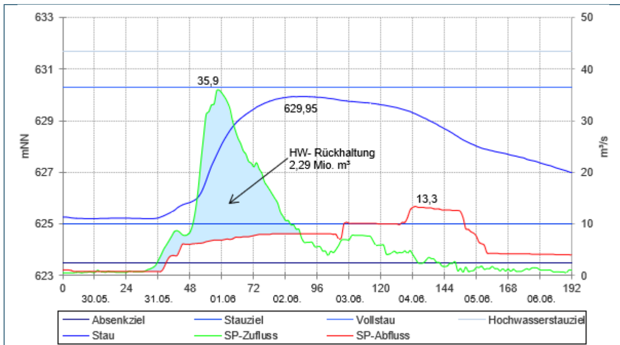
Abb. 36: Hochwasserbetrieb Windachspeicher (Quelle: WWA Weilheim)
