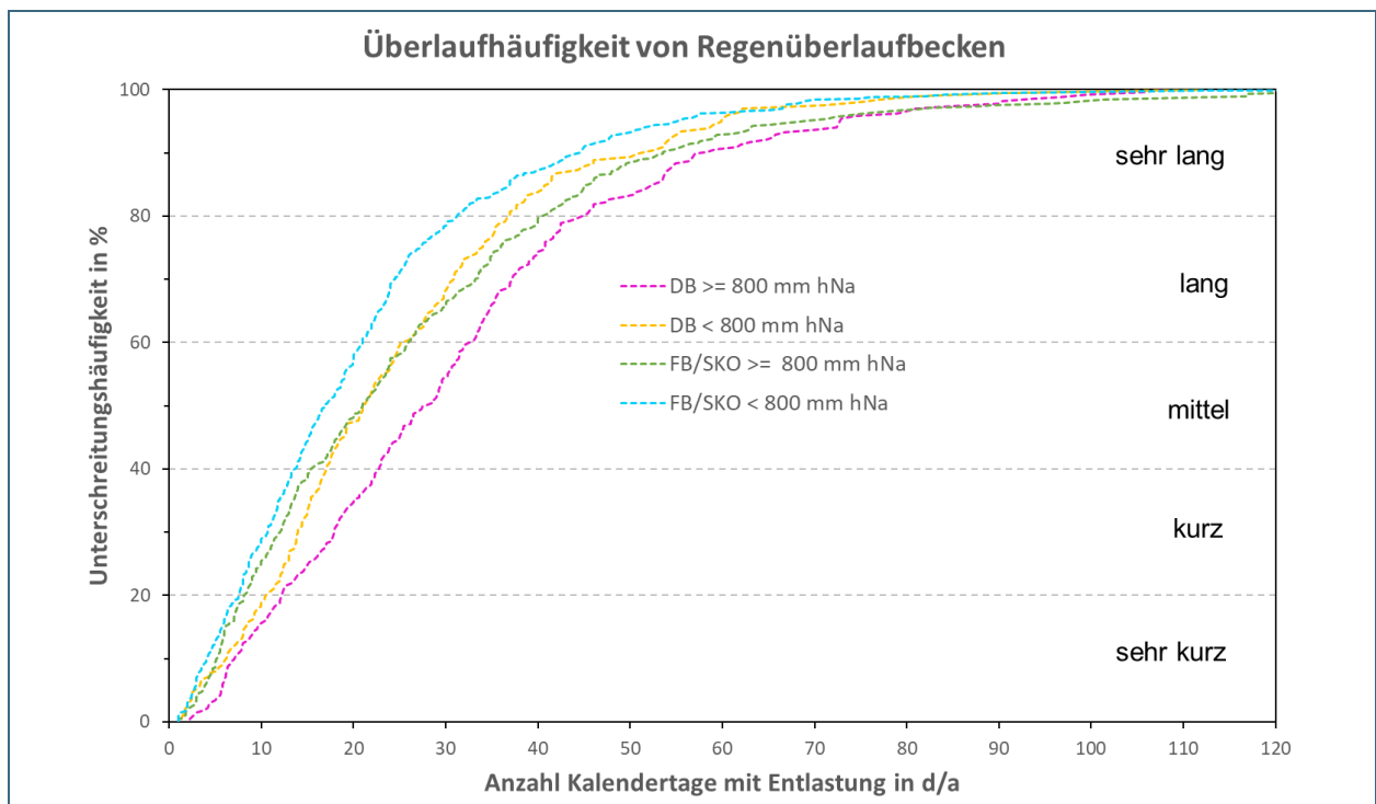
Abb. 4: Ranking-Kurve für die Anzahl der Tage mit Überlauf pro Jahr für Durchlaufbecken (DB), Fangbecken (FB) und Stauraumkanäle mit oberliegender Entlastung (SKO); Auswertung für unterschiedliche Bereiche der mittleren Jahresniederschlagshöhe (Stand Auswertung: August 2024)
