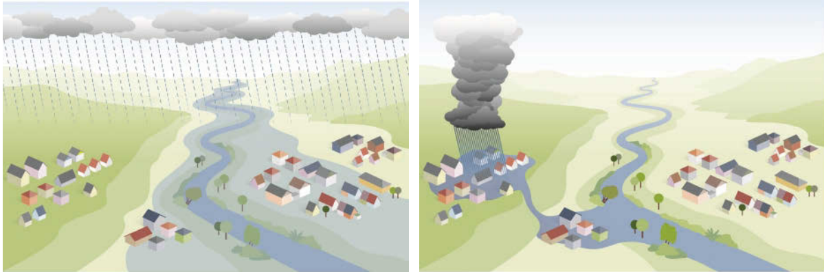
Abb. 6: Entstehung von fluvialem Hochwasser (links) und pluvialen Überflutungen (rechts): Fluviales Hochwasser an Fließgewässern entsteht durch länger anhaltenden Regen und geht von einem Gewässer aus; pluviale Überflutungen entstehen durch lokal begrenzten Starkregen direkt auf der Geländeoberfläche und können daher überall auftreten.
