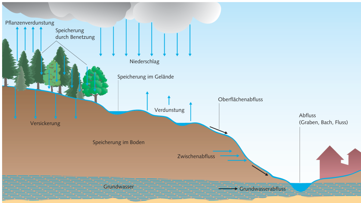
Abb. 3: Wichtige Prozesse, die Einfluss auf die Bildung von Oberflächenabfluss haben.
