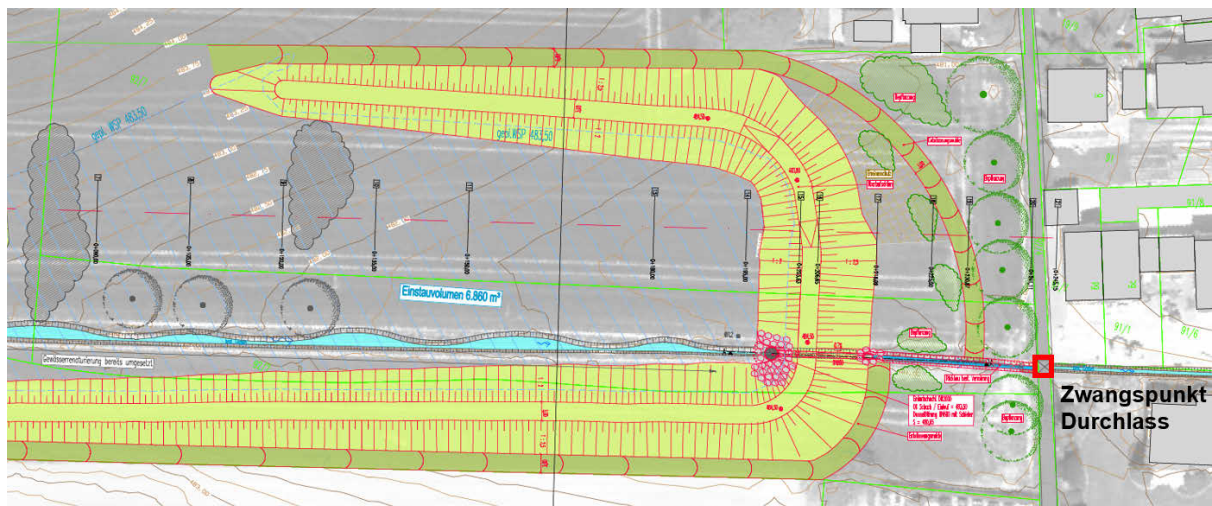
Abb. 23: Ausschnitt aus der Entwurfsplanung für das noch nicht gebaute Hochwasserrückhaltebecken. Im rechten Bereich befindet sich die Bebauung. Der Bereich des Durchlasses ist ein Zwangspunkt der den Wasserabfluss begrenzt und erhalten werden soll (ohne Maßstab). © Geobasisdaten: Bayerische Vermessungsverwaltung.
