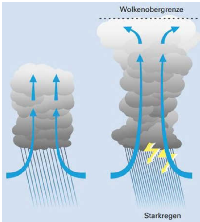
Abb. 2: Wolkenbildung durch Konvektion und Entstehung eines Starkregens.
