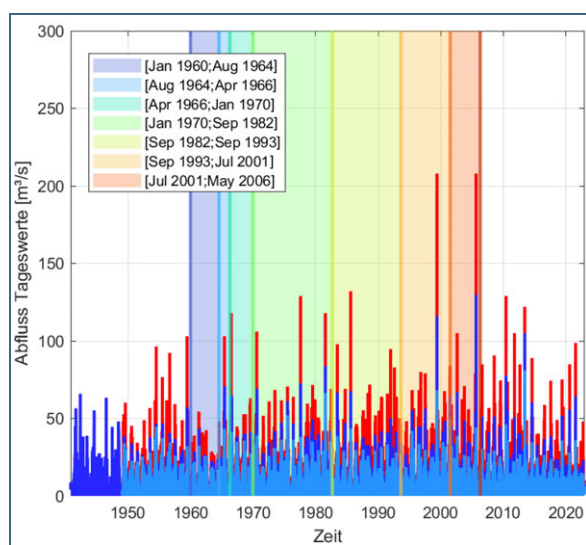
Abb. 47: Abflusstageswerte am Pegel Reißbachklamm (Minimum: hell- blau, Mittelwert: blau, Maxi- mum: rot) mit farbig hinterlegten Auswertepochen
