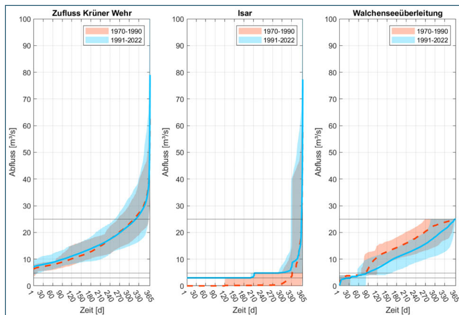
Abb. 29: Abflussdauerlinien am Krüner Wehr, für den Zufluss (links), den verbleibenden Abfluss in der Isar (mittig) und die Ausleitungsmenge in den Kanal zum Walchensee (rechts) für den Zeitraum bis 1990 (rot) und ab 1991 (blau) (Beginn Mindestwasserabgabe). Farbige hinterlegte Flächen spiegeln die Bandbreite zwischen Minimum und Maximum der jeweiligen Epoche wieder.
