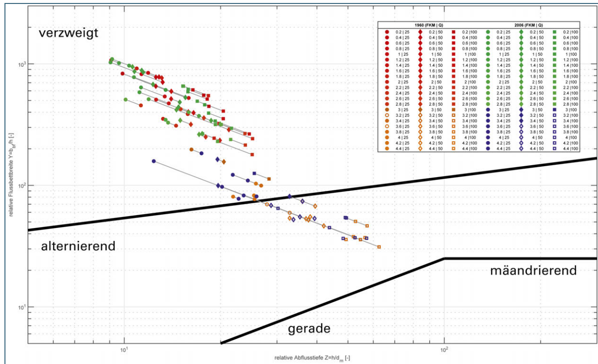
Abb. 63: Rißbach: Abgrenzung nach Da Silva (1991) entlang des Flusslaufs FKM 0,2 – 4,4 für die Profile aus dem Jahr 1960 (rot-orange) und dem Jahr 2006 (grün-blau) für je drei Abflüsse Q 25 m^3/s (Kreis), 50 m^3/s (Raute) und 100 m^3/s (Viereck). Datenpaare sind entsprechend nach FKM|Q benannt.
