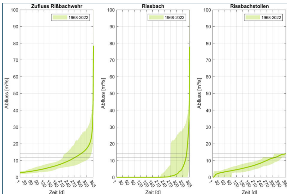
Abb. 31: Abflussdauerlinien am Rißbachwehr, für den Zufluss (links), den Rißbach unterhalb des Wehrs (mittig) und die Ausleitungsmenge in den Stollen (rechts). Die farbig hinterlegte Fläche spiegelt die Bandbreite zwischen Minimum und Maximum wieder.
