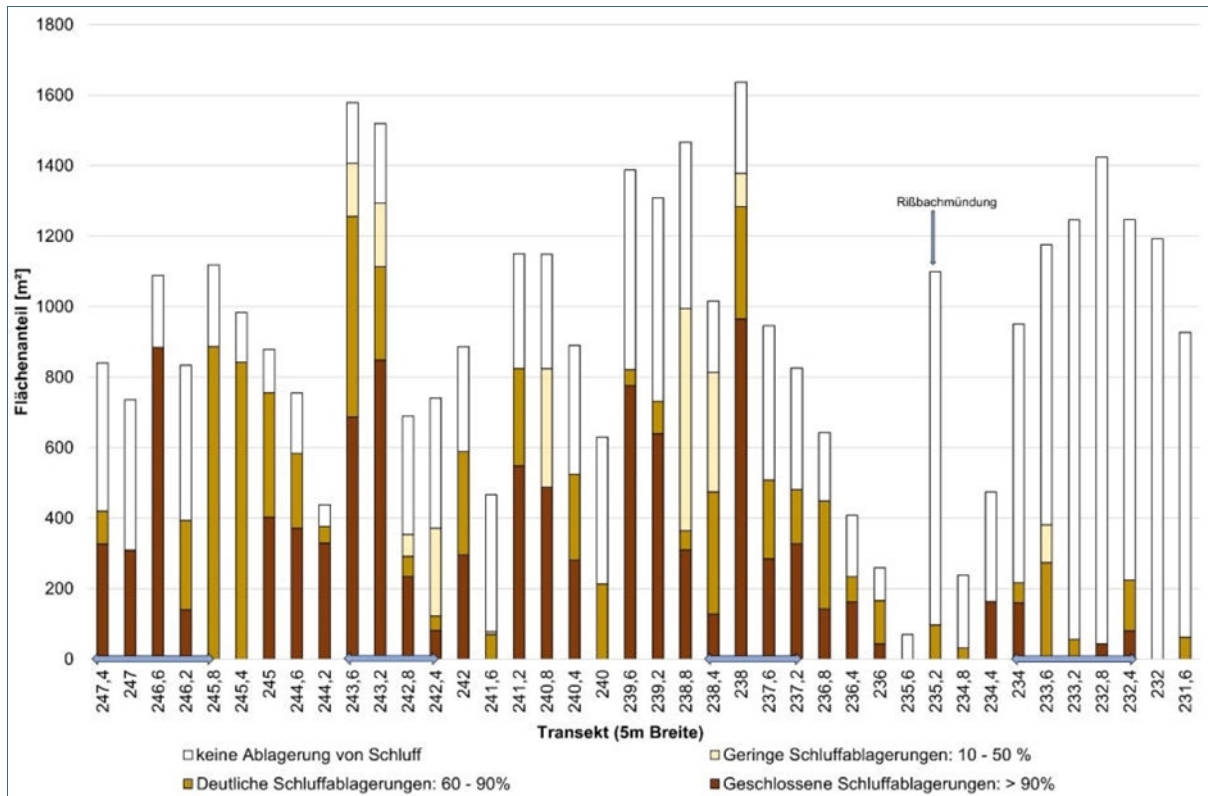
Abb. 59: Isar (Krün bis Reißbachmündung): Verteilung von Schluffablagerungen im Längsverlauf
