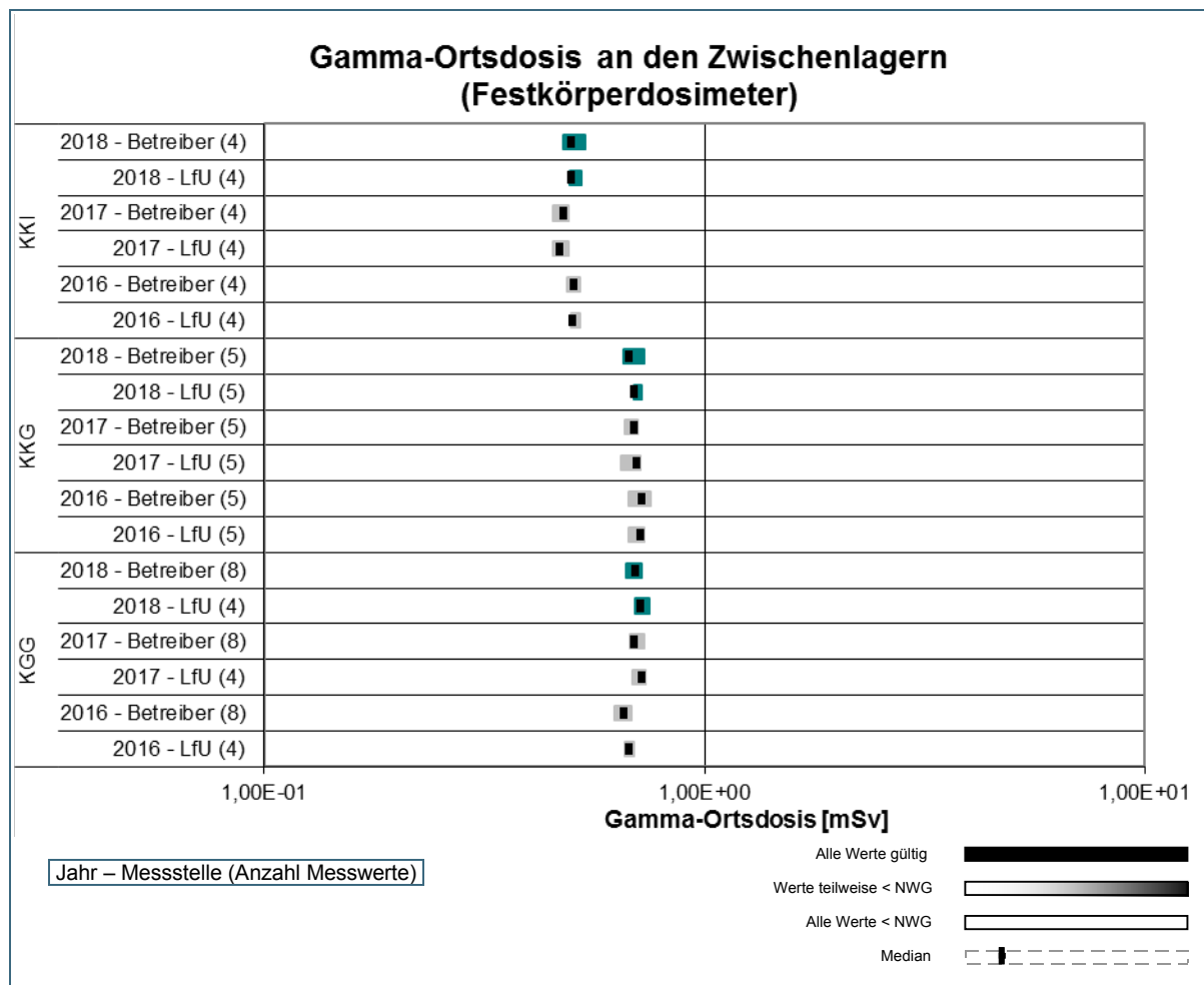
Abb. 13: Übersicht über die Wertebereiche der Gamma-Ortsdosis (G-OD) an den Brennelementzwischenlagern gem. REI, Tabelle C1.1, Punkt 1.2 und Tabelle C1.2, Punkt 1.1 im Jahr 2018 im Vergleich zu den Vorjahren 2017 und 2016.
