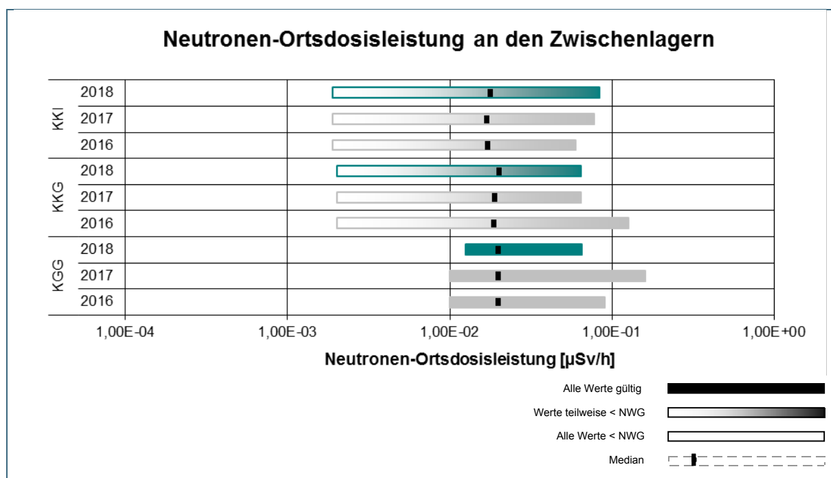
Abb. 12: Übersicht über die Wertebereiche der Neutronen-Ortsdosisleistung (N-ODL) an den Brennelementzwischenlagern gem. REI, Tabelle C1.1, Punkt 1.3 im Jahr 2018 im Vergleich zu den Vorjahren 2017 und 2016
