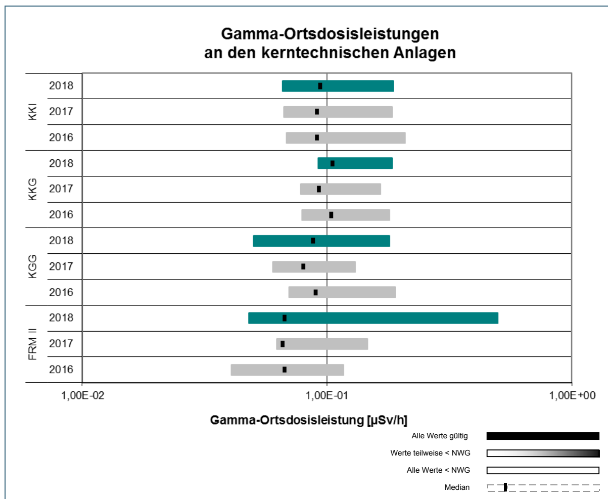
Abb. 9: Übersicht über die Wertebereiche der Gamma-Ortsdosisleistung an den kerntechnischen Anlagen (aus 10-Minuten-Messwerten) gem. REI, Tabelle A1, Punkt 1.1a im Jahr 2018 im Vergleich zu den Vorjahren 2017 und 2016
