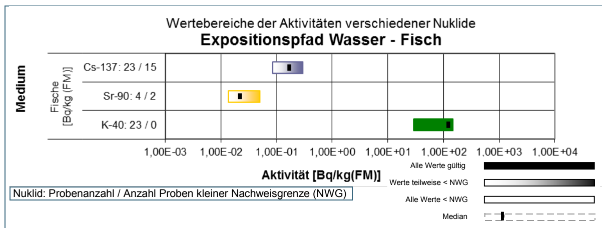
Abb. 3: Wertebereiche der in Bayern gemessenen Aktivitäten des Expositionspfads Ernährungskette Wasser im Jahr 2018
