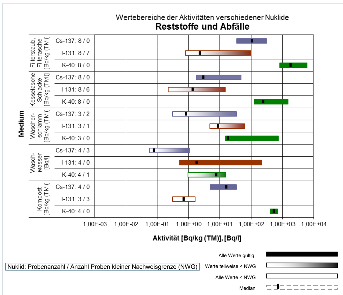
Abb. 8: Wertebereiche der in Bayern gemessenen Aktivitäten von Reststoffen und Abfällen im Jahr 2018
