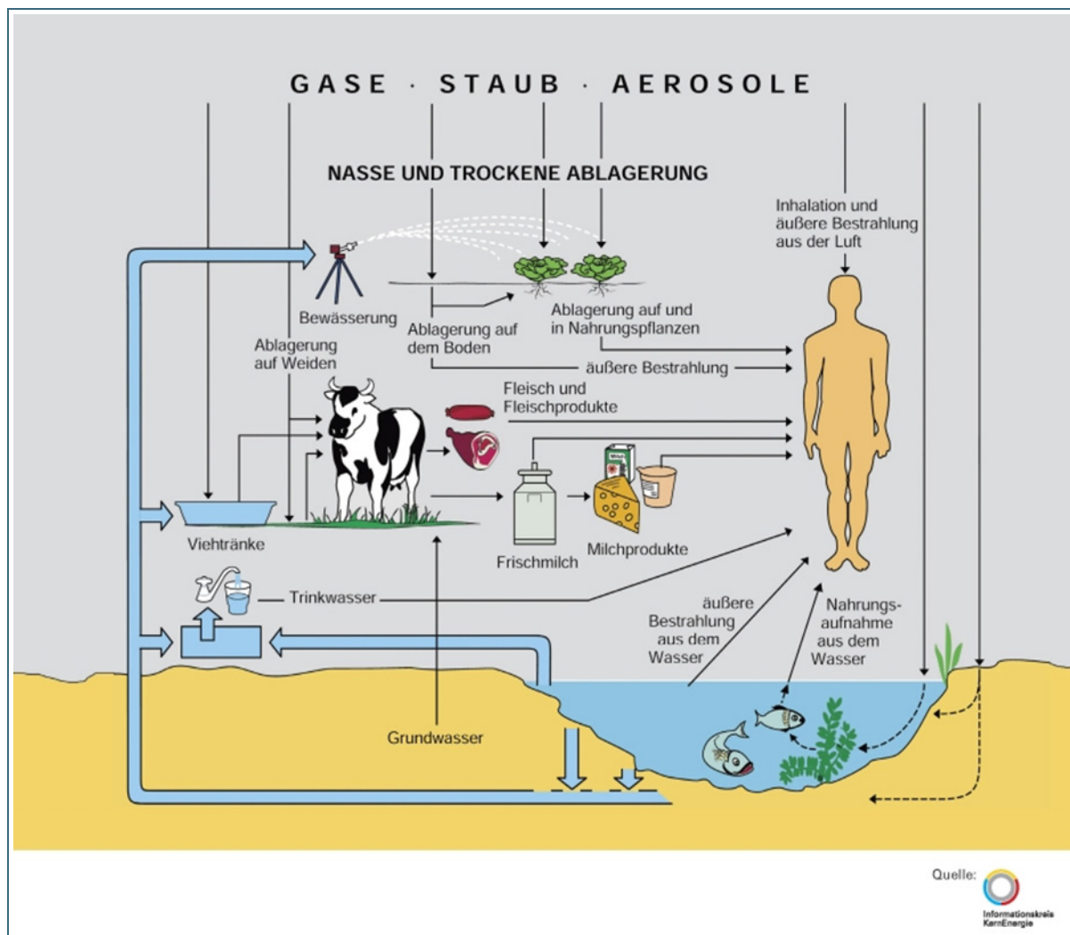
Abb. 1: Mögliche Transportwege radioaktiver Stoffe zum Menschen Quelle: Informationskreis Kernenergie
