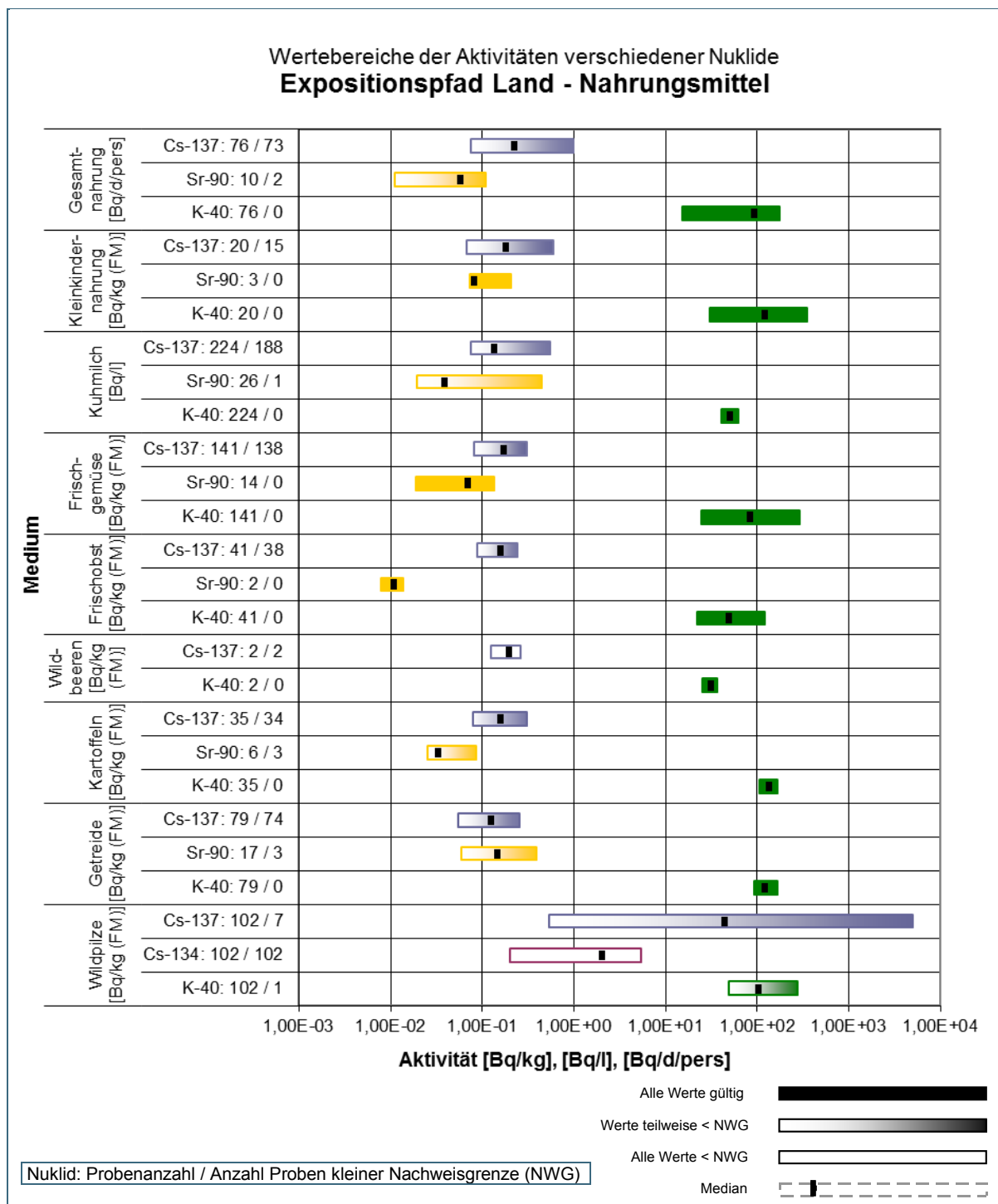
Abb. 5: Wertebereiche der in Bayern gemessenen Aktivitäten des Expositionspfads Ernährungskette Land – Nahrungsmittel (ohne tierische Lebensmittel) im Jahr 2018
