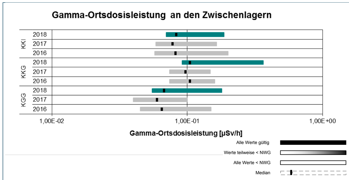
Abb. 11: Übersicht über die Wertebereiche der Gamma-Ortsdosisleistung (G-ODL) an den Brennelementzwischenlagern gem. REI, Tabelle C1.1, Punkt 1.1 im Jahr 2018 im Vergleich zu den Vorjahren 2017 und 2016
