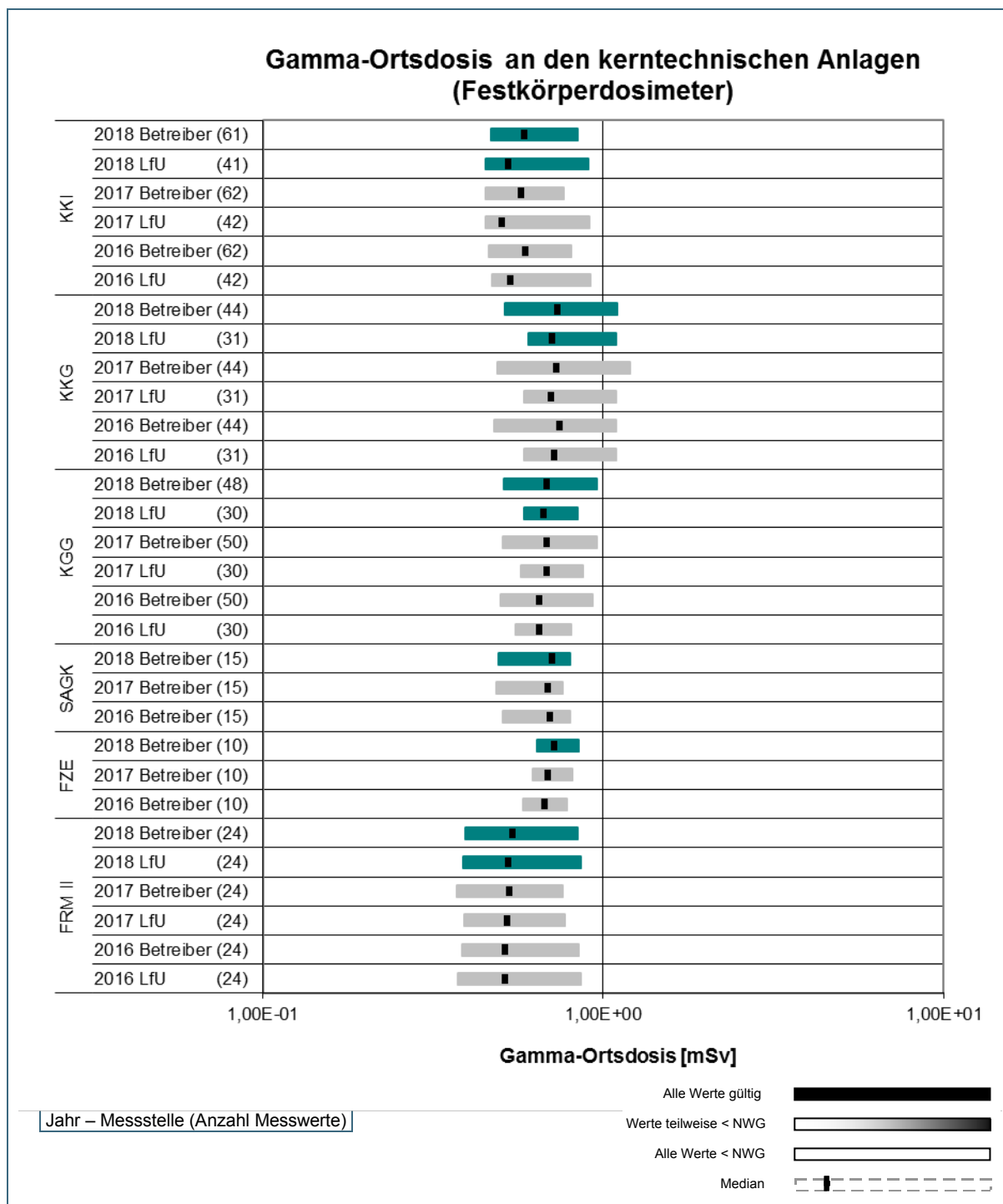
Abb. 10: Übersicht über die Wertebereiche der Gamma-Ortsdosis (Jahresdosis von Festkörperdosimetern) gem. REI, Tabelle A1, Punkt 1.1b und Tabelle A2, Punkt 1.1 im Jahr 2018 im Vergleich zu den Vorjahren 2017 und 2016.
