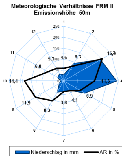
Abb. 15: Häufigkeitsverteilung der Ausbreitungsrichtung (AR) in % sowie die Niederschlagsmenge in mm pro Sektor der überwachten kerntechnischen Anlagen im Jahr 2018
