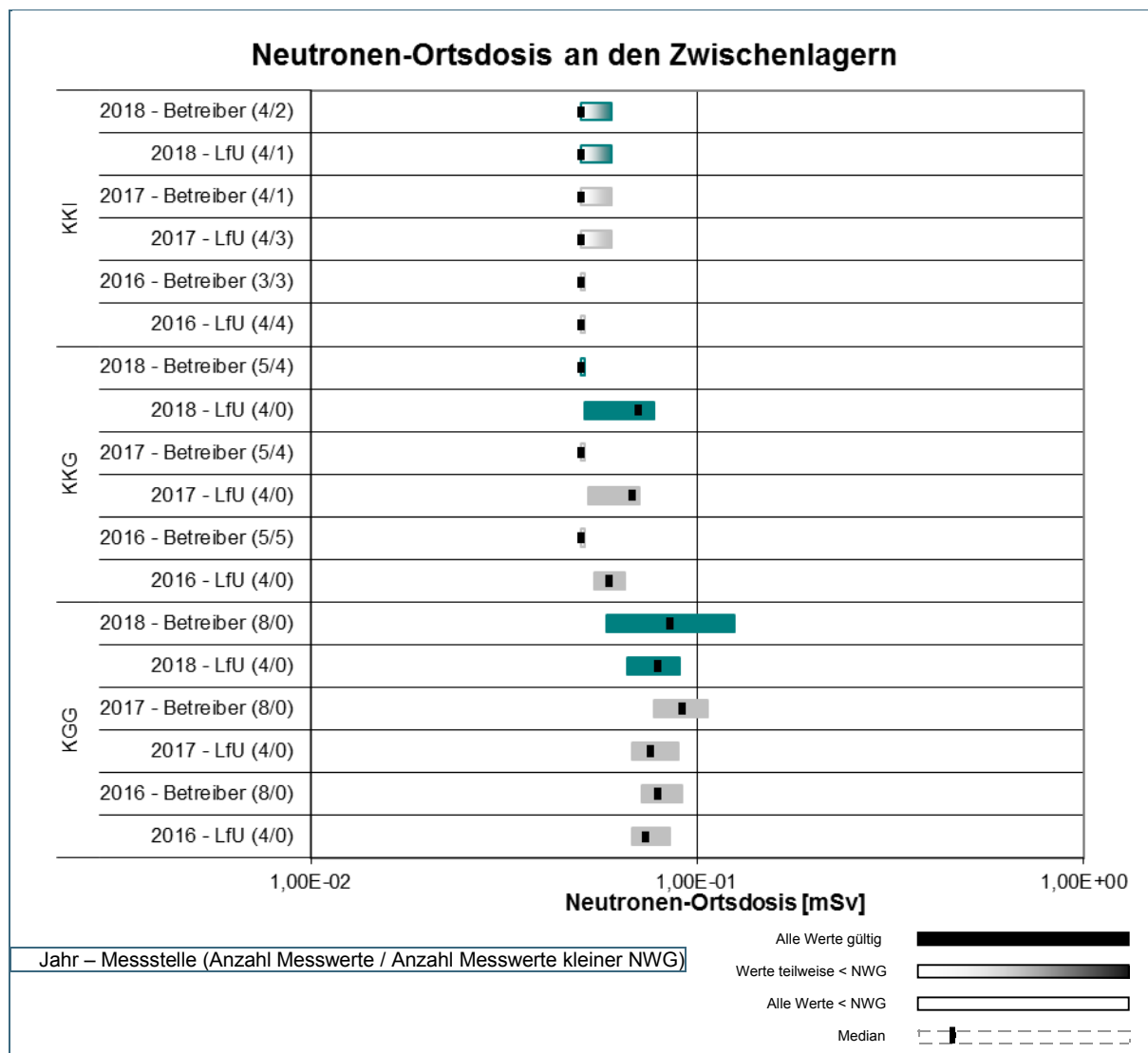
Abb. 14: Übersicht über die Wertebereiche der Neutronen-Ortsdosis (N-OD) an den Brennelementzwischenlagern gem. REI, Tabelle C.1.1, Punkt 1.4 und Tabelle C.1.2, Punkt 1.2 im Jahr 2018 im Vergleich zu den Vorjahren 2017 und 2016
