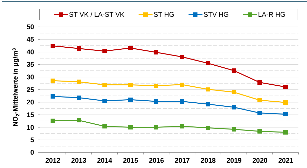
Abb. 11: Stickstoffdioxid (NO 2 ) – Entwicklung der Belastung in den Belastungsniveaus verkehrsorientierter (ST VK / LA-ST VK), städtischer (ST HG), vorstädtischer (STV HG) und ländlicher Messstationen (LA-R HG). Vergleiche Tab. 1, S. 8, zur Erläuterung der Abkürzungen.
