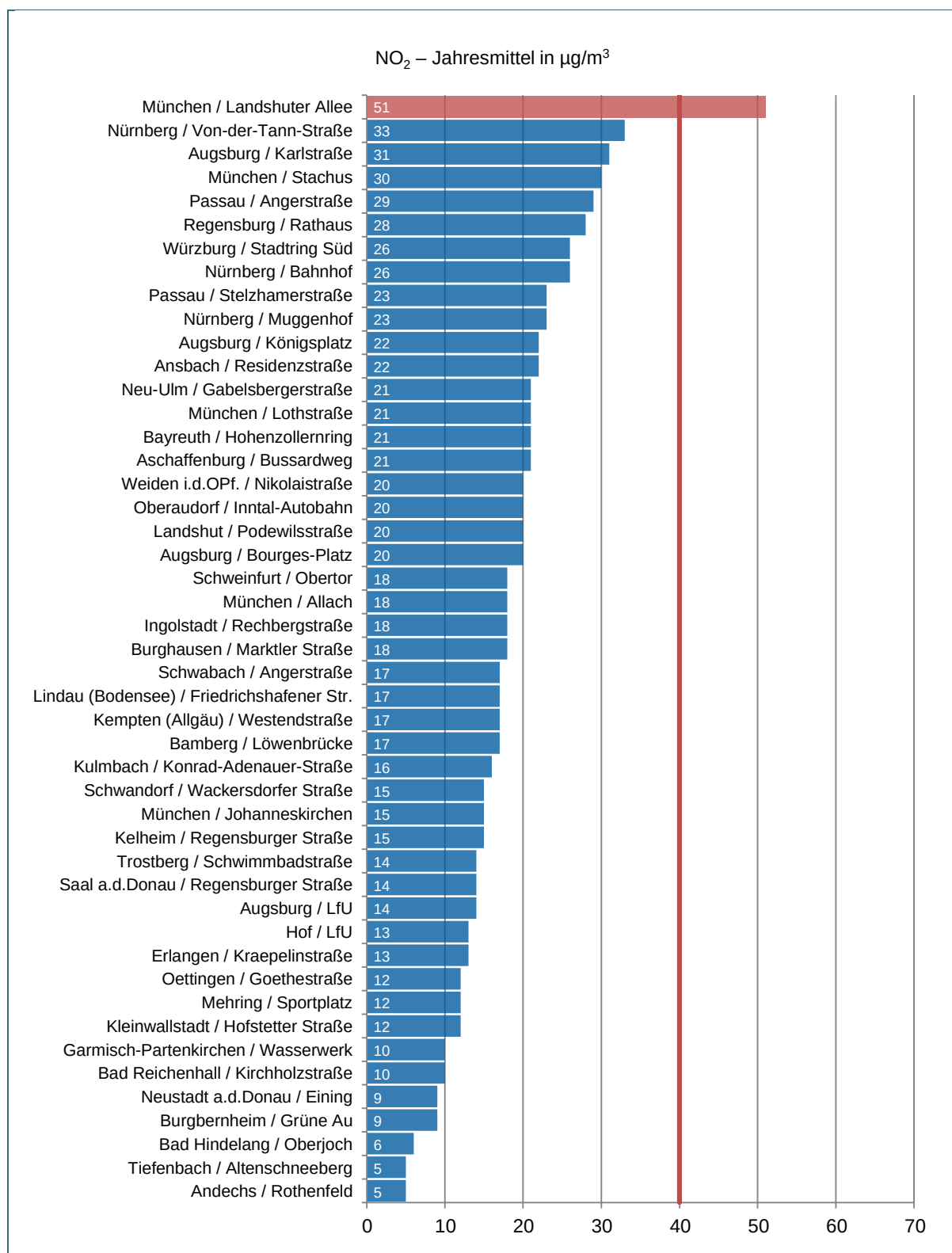
Abb. 3: Stickstoffdioxid (NO 2 ) – Jahresmittelwerte (absteigend sortiert); die rote Linie markiert den Grenzwert der 39. BImSchV [3] von 40 µg/m 3 .
