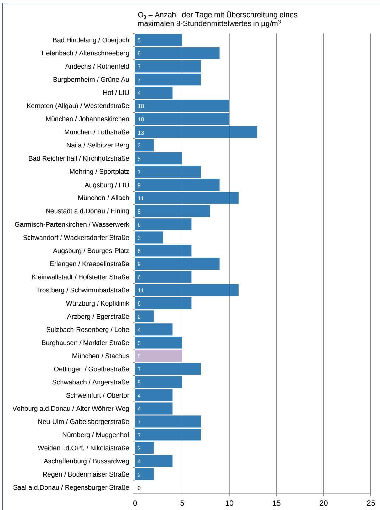
Abb. 8: Ozon (O 3 ) – Anzahl der Tage mit Überschreitung des maximalen 8-Stundenmittelwerts (im Kalenderjahr, absteigend sortiert nach dem Jahresmittelwert entsprechend Abb. 7). Die Ozonmessung an der verkehrsnahen Station München/Stachus (Balken lila eingefärbt) ist nicht für die Beurteilung vorgesehen und dient Zwecken der Qualitätssicherung und Ursachenforschung.
