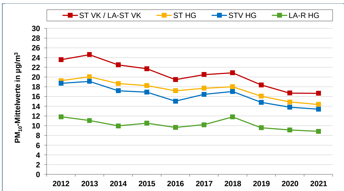
Abb. 12: Feinstaub PM 10 – Entwicklung der Belastung in den Belastungsniveaus verkehrsorientierter (ST VK / LA-ST VK), städtischer (ST HG), vorstädtischer (STV HG) und ländlicher Messstationen (LA-R HG). Vergleiche Tab. 1, S. 8, zur Erläuterung der Abkürzungen.
