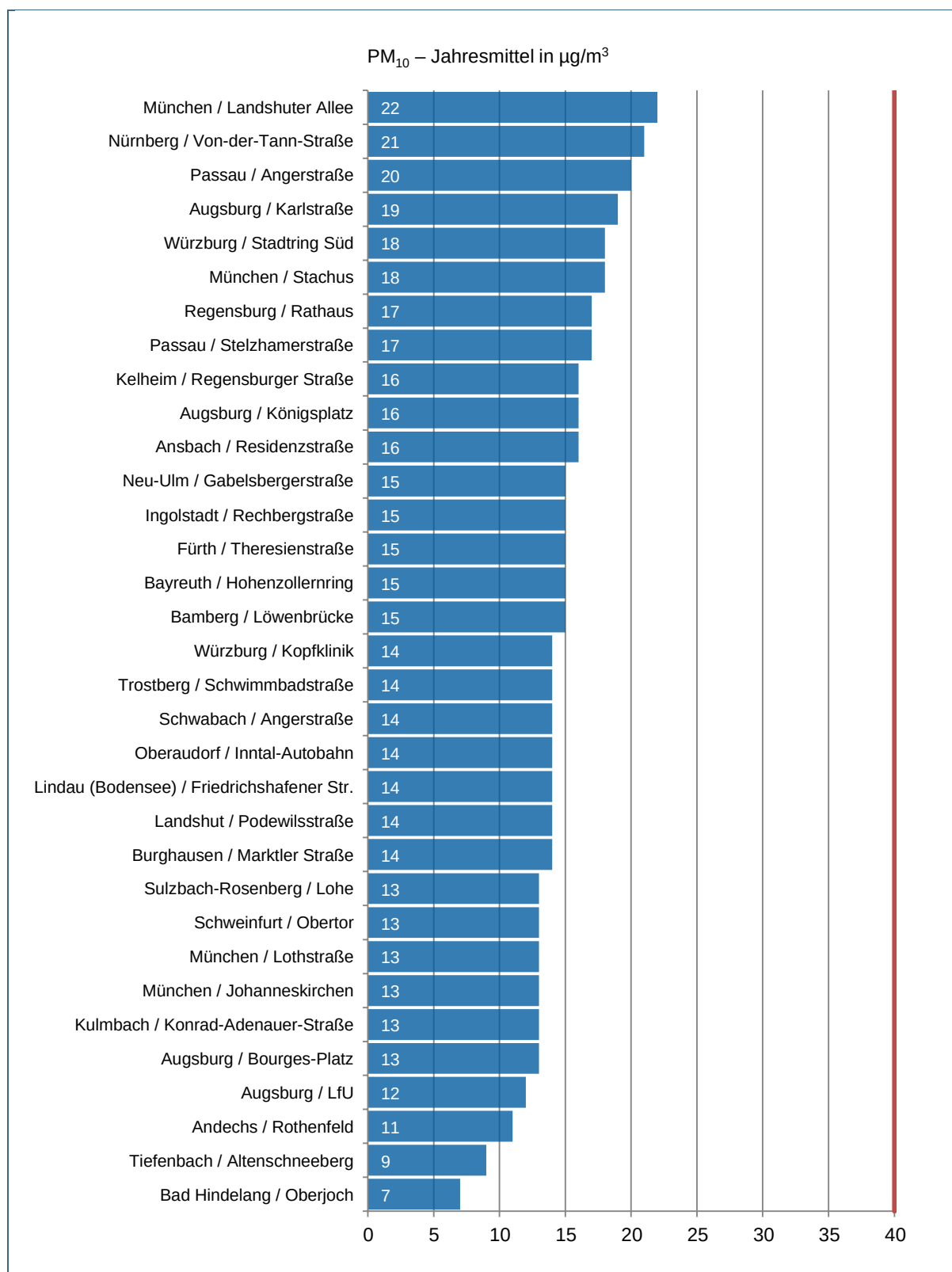
Abb. 4: Feinstaub PM 10 – Jahresmittelwerte (absteigend sortiert); die rote Linie markiert den Grenzwert der 39. BImSchV [3] von 40 µg/m 3 .
