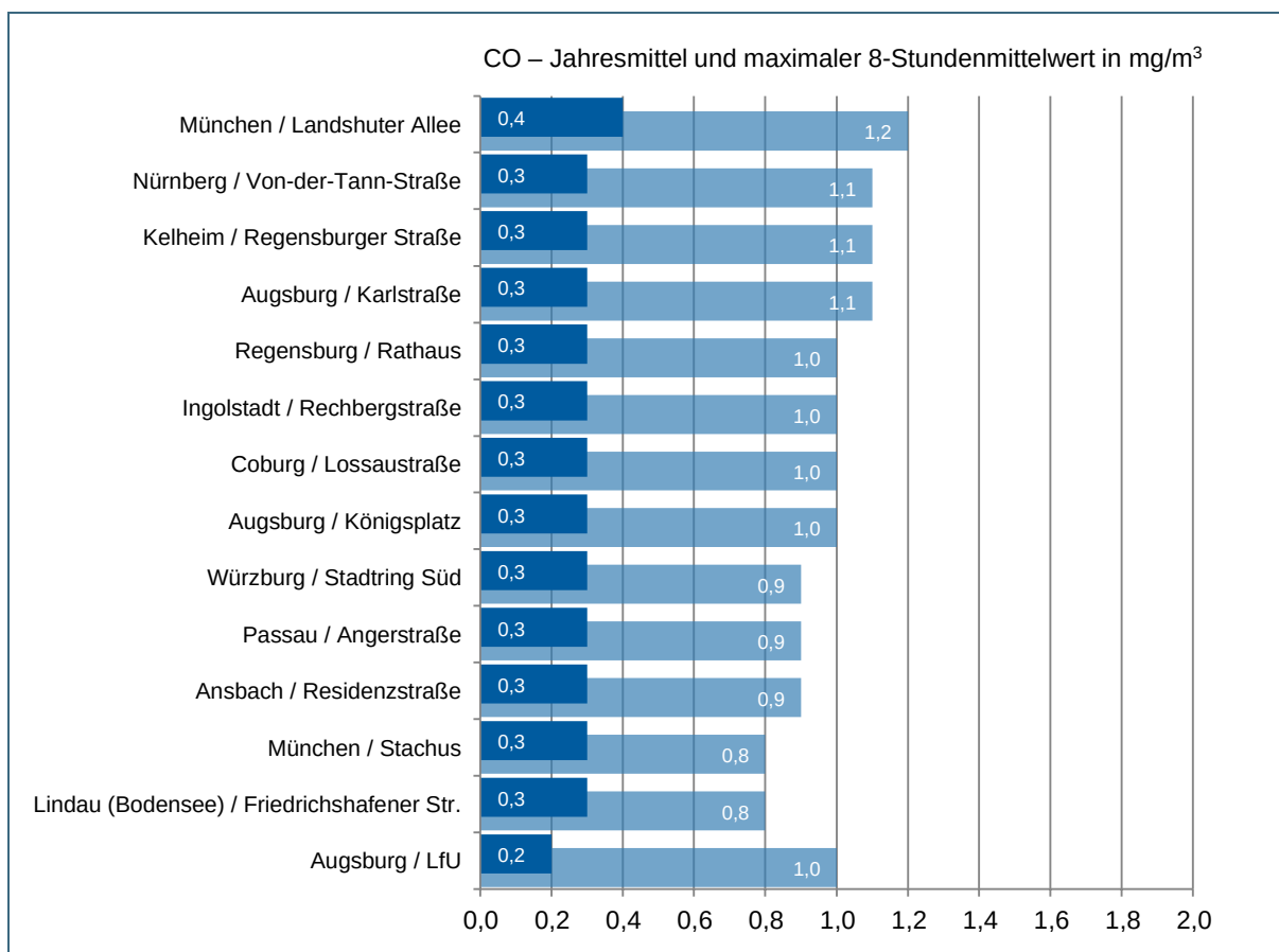
Abb. 10: Kohlenmonoxid (CO) – Jahresmittelwerte (dunkelblau) und maximaler 8-Stundenmittelwert (hellblau) absteigend sortiert nach dem Jahresmittelwert; nicht enthalten ist aus Darstellungsgründen eine Markierung für den Grenzwert des maximalen 8-Stundenmittelwerts von 10 mg/m 3 nach der 39. BImSchV [3], der dem fünffachen der Länge der Abszisse entspricht.
