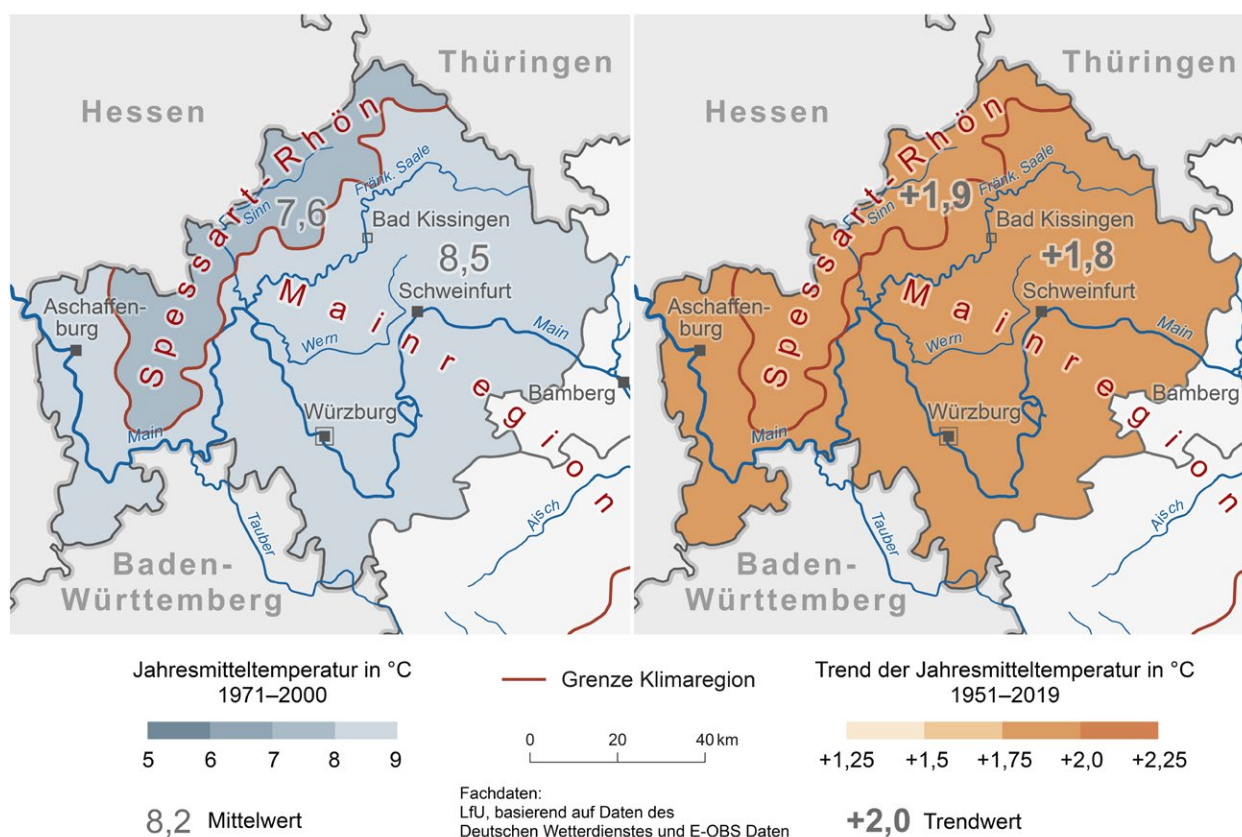
Abb. 2: Mittlere Lufttemperatur 1971–2000 (links) und Änderung der Temperatur 1951–2019 (rechts) in Unterfranken
