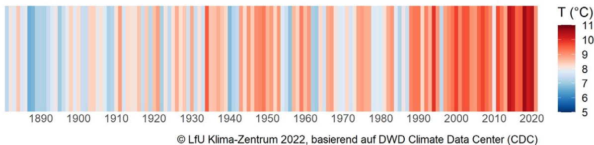
Abb. 1: Warming Stripes 1881–2021 für Unterfranken (Ein Jahr ist je nach mittlerer Temperatur mit einem farbigen Strich – von dunkelblau (kalt) über hellblau und hellrot bis dunkelrot (warm) – abgebildet.)
