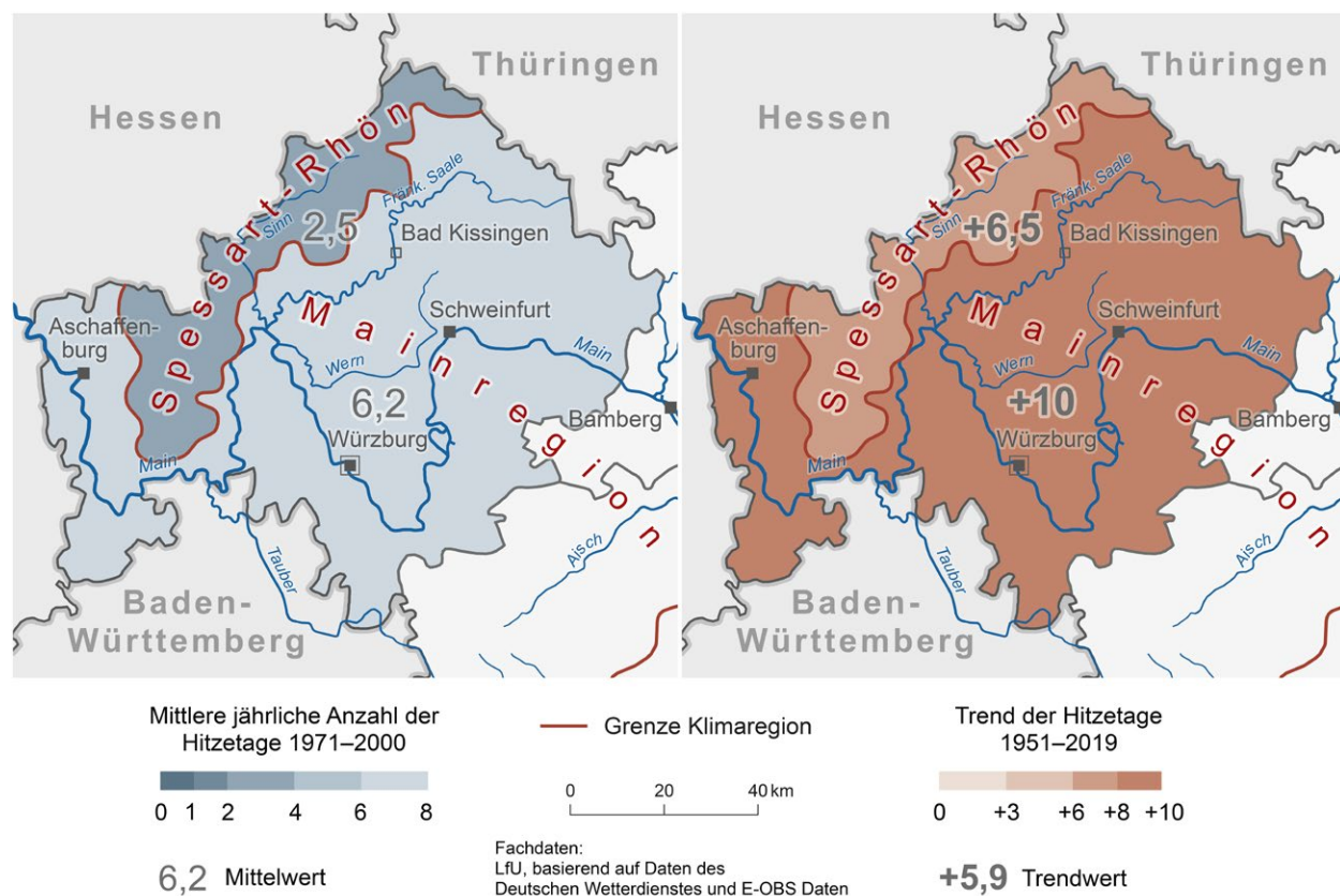
Abb. 4: Jährliche Anzahl der Hitzetage 1971–2000 (links) und Änderung der Hitzetage 1951–2019 (rechts) in Unterfranken
