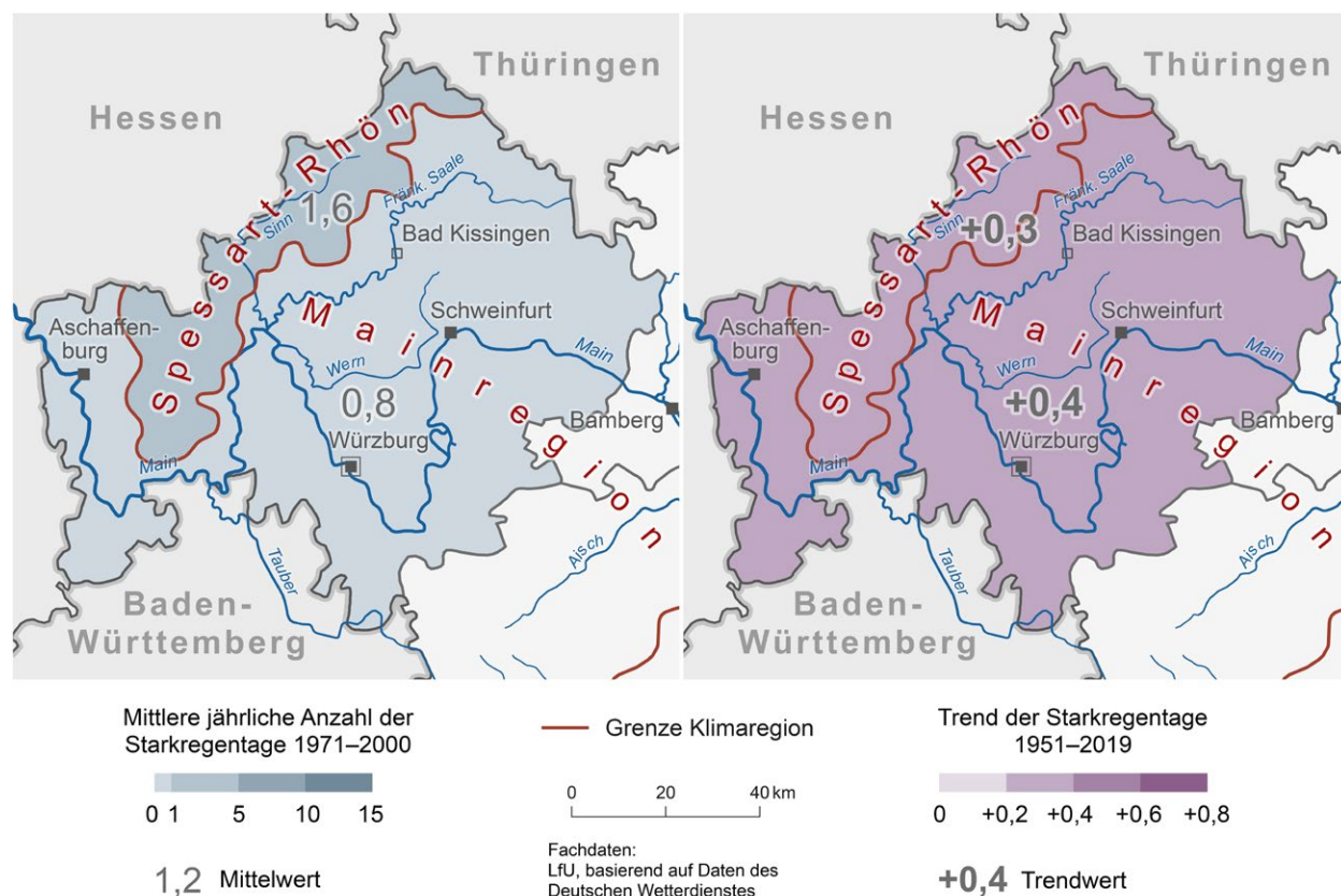
Abb. 3: Jährliche Anzahl der Starkregentage 1971–2000 (links) und Änderung der Starkregentage 1951–2019 (rechts) in Unterfranken
