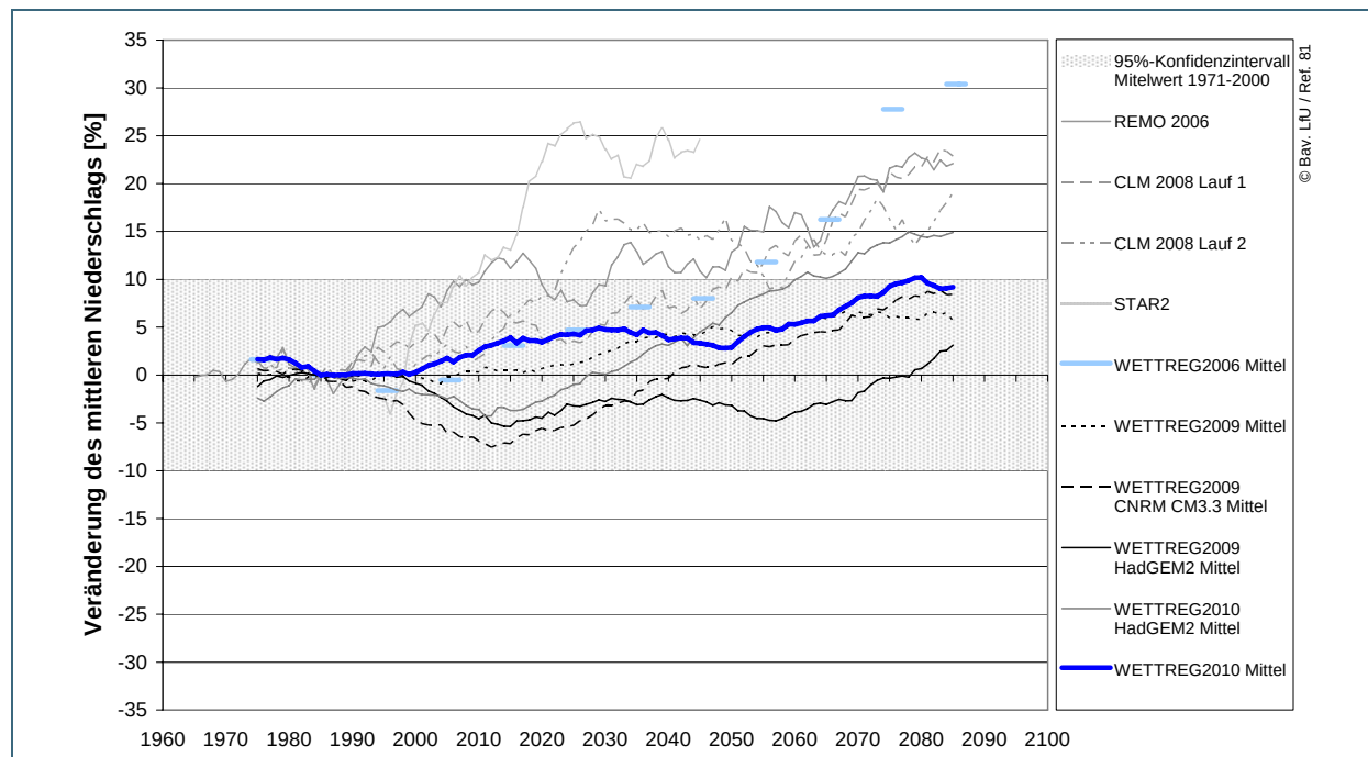
Abb. 9: Relative Änderung des 30-jährigen gleitenden Mittelwerts des Gebietsniederschlags im hydrologischen Winterhalbjahr gegenüber 1971–2000 in [%] für die Region Unterer Main. Der Vertrauensbereich des Mittelwerts 1971–2000 ( \pm 10\% , graues Band) berücksichtigt die natürliche Variabilität der Halbjahreswerte dieses Zeitraums und dient als Hinweis auf die Signifikanz des Änderungssignals. WETTREG2010 (blau) und WETTREG2006 (hellblau) sind hervorgehoben; für die WETTREG-Projektionen ist der Mittelwert aus zehn Realisationen dargestellt. Wenn nicht anders angegeben, ist ECHAM5 als antreibendes GCM genutzt.
