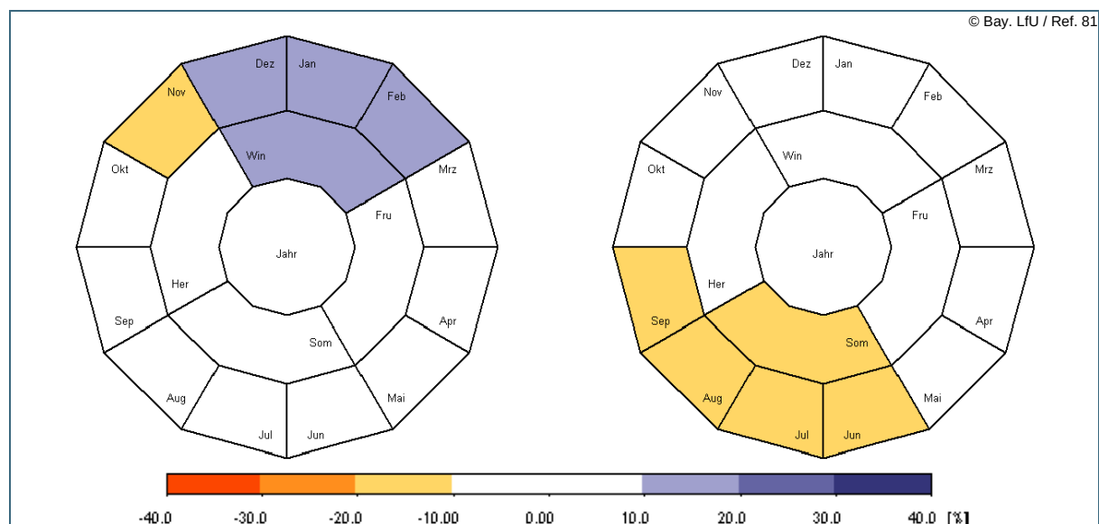
Abb. 12: Veränderung der Niederschlagssumme von 2021–2050 gegenüber 1971–2000 bei WETTREG2006 (links) und WETTREG2010 (rechts) für unterschiedliche Perioden; mittlere jährliche Änderung (innerer Ring), mittlere jahreszeitliche Änderung (mittlerer Ring) und mittlere monatliche Änderung (äußerer Ring) in [%].
