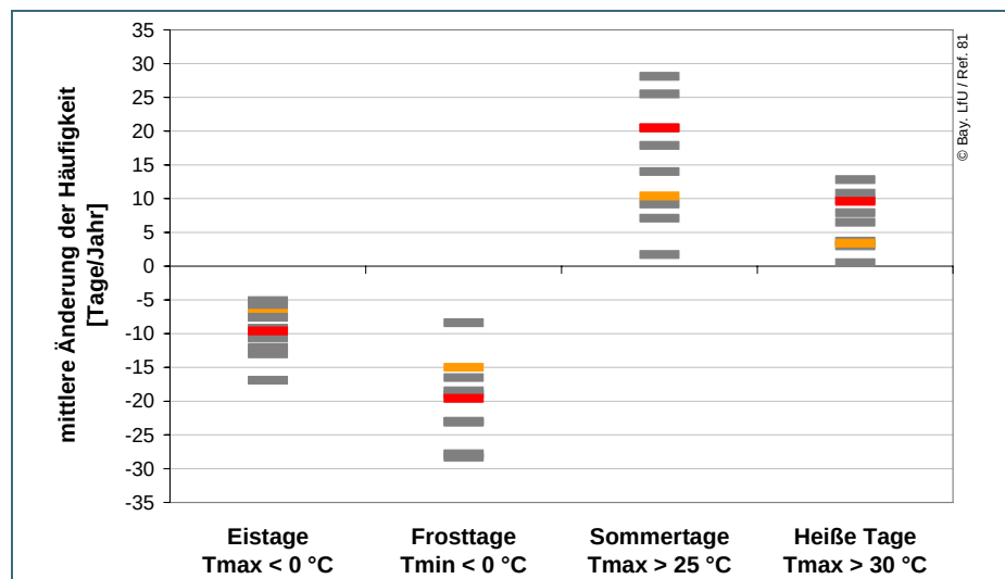
Abb. 8: Spannweite der mittleren Veränderung der Häufigkeit der Kenntage pro Jahr für die Region Unterer Main; Vergleich der Zeiträume 2021–2050 und 1971–2000; Auswertung von zehn regionalen Klimaprojektionen (in grau); WETTREG2006 (in orange) und WETTREG2010 (in rot) sind hervorgehoben.
