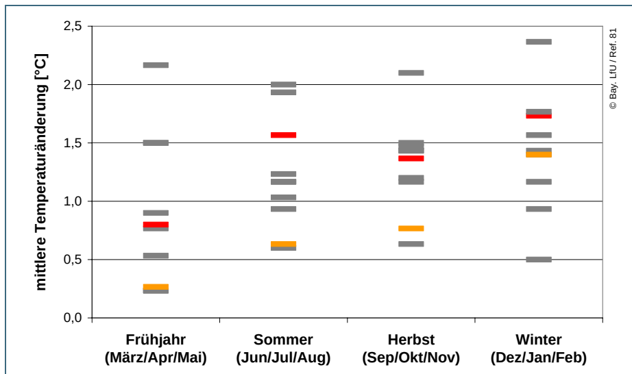
Abb. 6: Jahreszeitliche Spannweite der Änderung der durch- schnittlichen Tempera- tur von zehn regionalen Klimaprojektionen in [°C] für die Region Unterer Main, Ver- gleich der Zeiträume 2021–2050 und 1971– 2000; WETTREG2006 (in orange) und WETTREG2010 (in rot) sind hervorgehoben.
