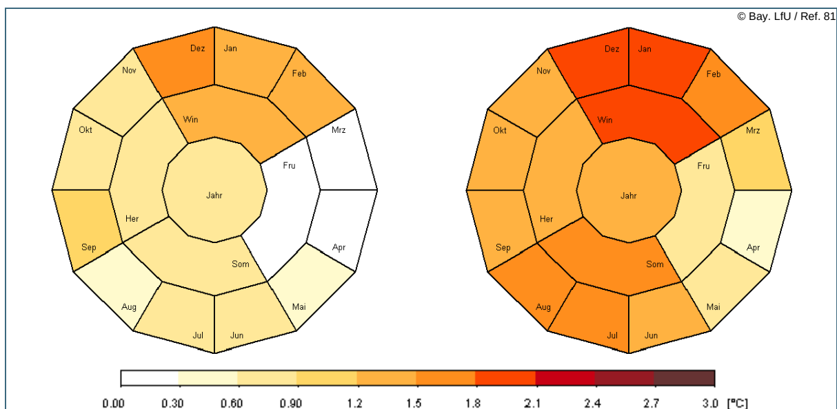
Abb. 7: Veränderung der Mitteltemperaturen 2021–2050 gegenüber 1971–2000 in [°C] bei WETTREG2006 (links) und WETTREG2010 (rechts) für die Region Unterer Main. Darstellung der jährlichen (innerer Ring), der jahreszeitlichen (mittlerer Ring) und der monatlichen Änderungen (äußerer Ring).
