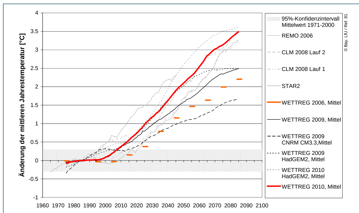
Abb. 5: Änderung des 30-jährigen, gleitenden Mittelwerts der Jahrestemperatur gegenüber dem Kontrollzeitraum 1971–2000 in [\text{°C}] für die Region Unterer Main. Der Vertrauensbereich des Mittelwerts 1971–2000 ( \pm 0,3\text{ °C} , graues Band) berücksichtigt die natürliche Variabilität der Jahreswerte dieses Zeitraums und dient als Hinweis auf die Signifikanz des Änderungssignals. WETTREG2010 (rot, durchgezogene Linie) liegt im oberen, WETTREG2006 (orange, gestrichelt) im unteren Bereich der Bandbreite; für die WETTREG-Projektionen ist der Mittelwert aus zehn Realisationen dargestellt. Wenn nicht anders angegeben, ist ECHAM5 als antreibendes Globalmodell genutzt.
