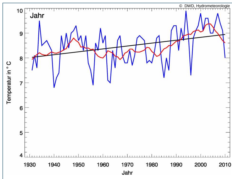
Abb. 2: Verlauf der Jahresmitteltemperatur im Flussgebiet Unterer Main (blau); gleitender zehnjähriger Mittelwert (rot) und linearer Trend (schwarz) 1931–2010
