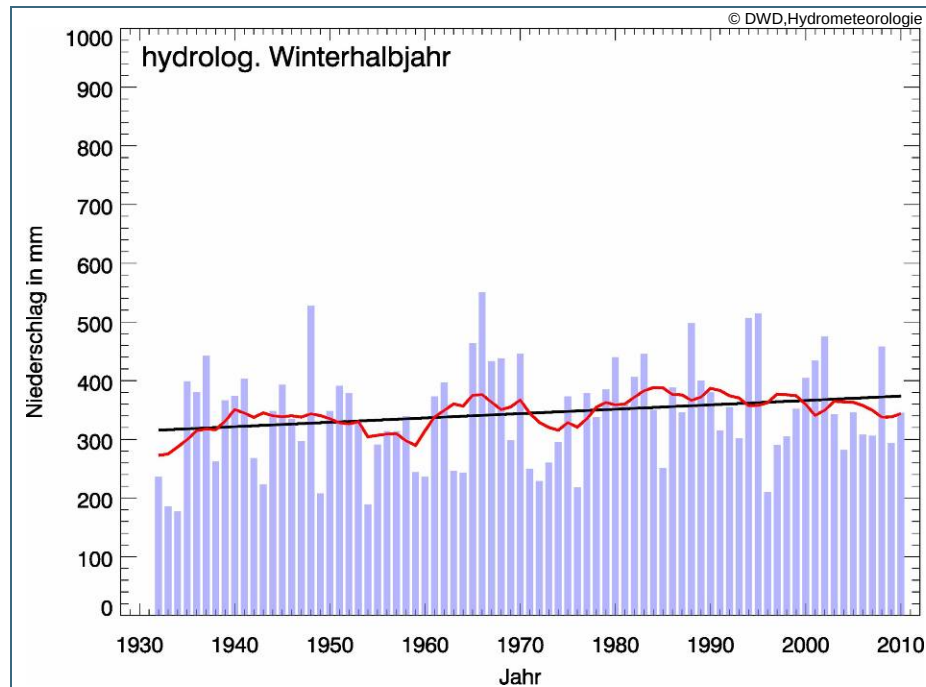
Abb. 3: Verlauf des mittleren Gebietsniederschlags im Flussgebiet Unterer Main (blau), gleitender zehnjähriger Mittelwert (rot) und linearer Trend (schwarz) für das hydrologische Winter- halbjahr, Zeitreihe 1931–2010
