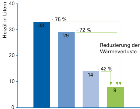
Vergleich des jährlichen Wärmeverlustes unterschiedlicher Fenstertypen pro m^2 Fensterfläche (umgerechnet in Liter Heizöl)
