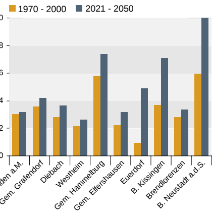
Unter dem Einfluss des Klimawandels auf das bisherige 100jährige Hochwasser sind zukünftig teilweise erheblich höhere Schäden in den Städten und Gemeinden zu erwarten.
