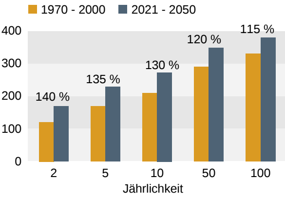
Erhöhung der Hochwasserabflüsse unterschiedlicher Jährlichkeiten durch den Klimawandel (Pegel Bad Kissingen)
