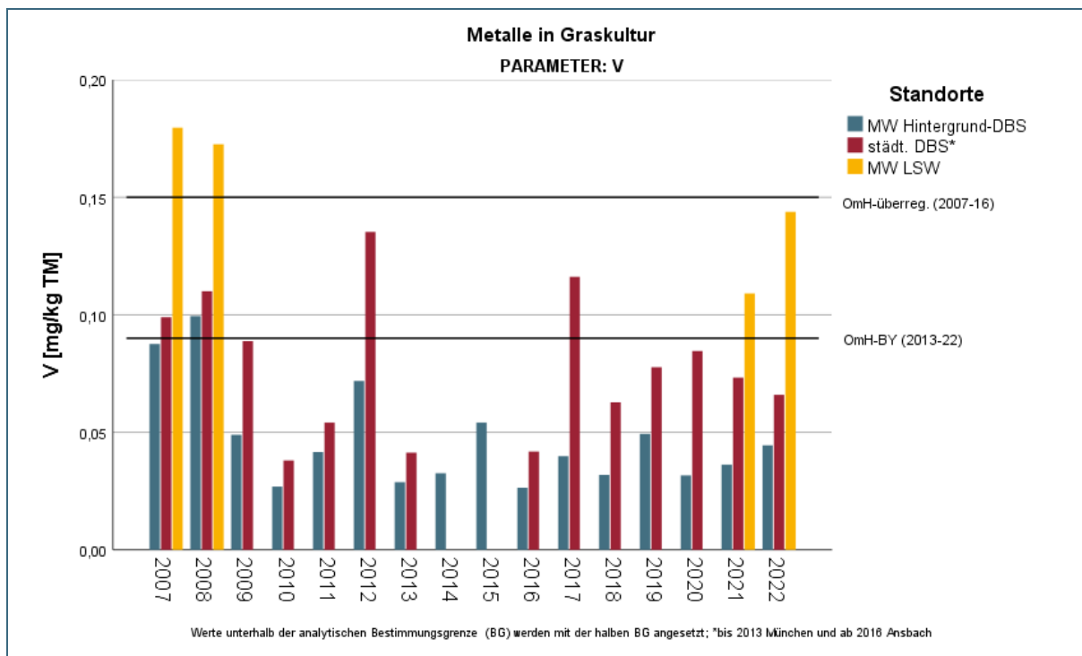
Abb. 42: Jahresmittelwerte der Vanadium-Gehalte in Graskulturen
