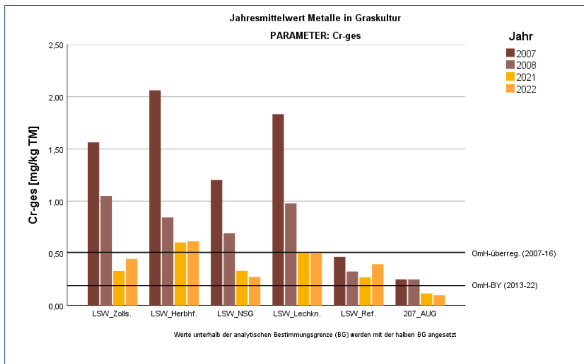
Abb. 39: Jahresmittelwerte der Chrom-Gehalte in Graskulturen im Umfeld der LSW und an der DBS Augsburg
