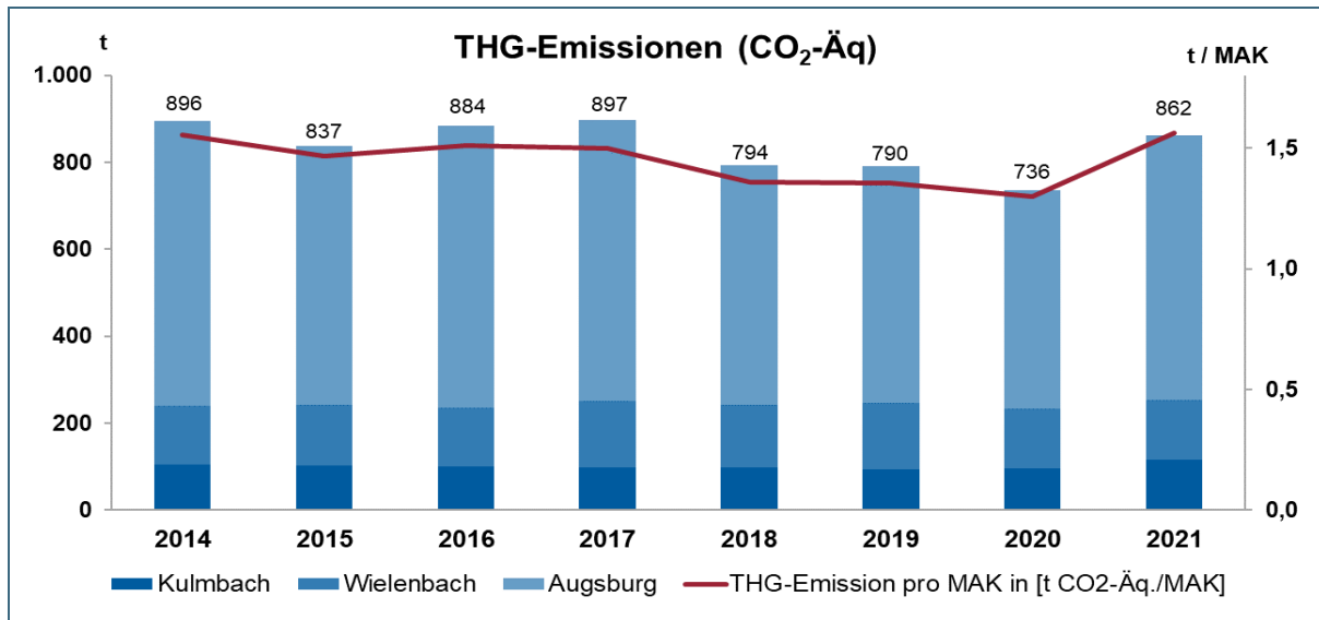
Abb. 16: Entwicklung der Treibhausgasemissionen für die Standorte Augsburg, Kulmbach und Wielenbach
