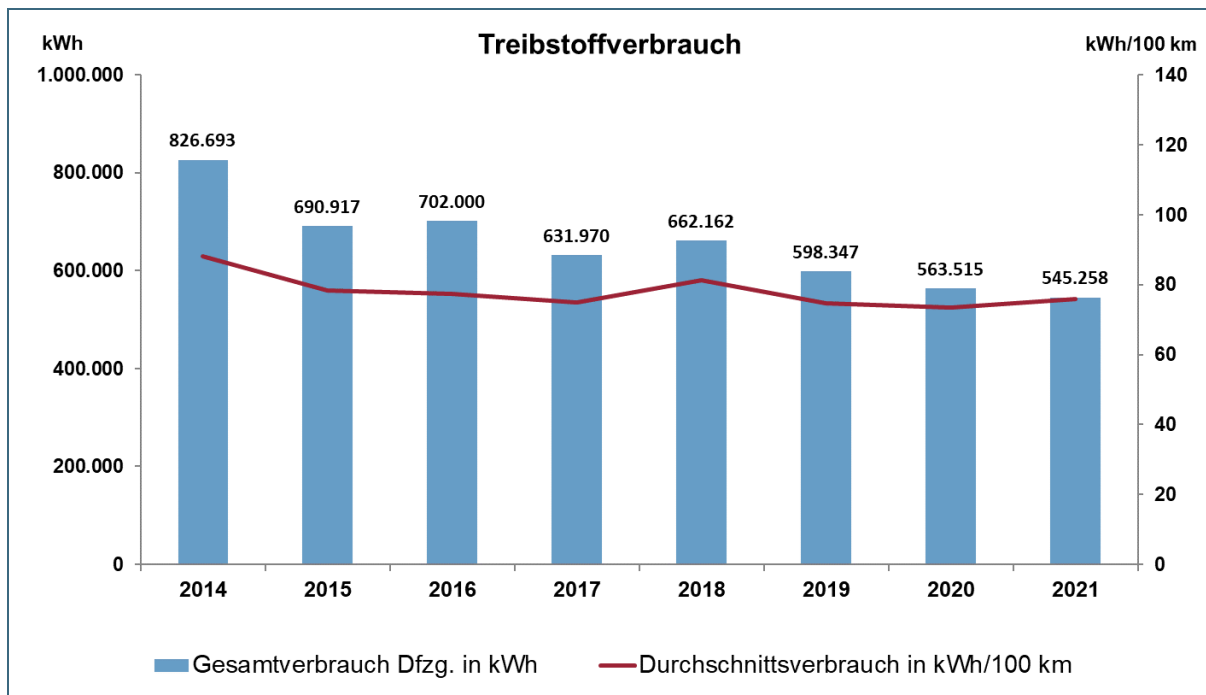
Abb. 13: Entwicklung des Treibstoffverbrauches für Dienstfahrzeuge
