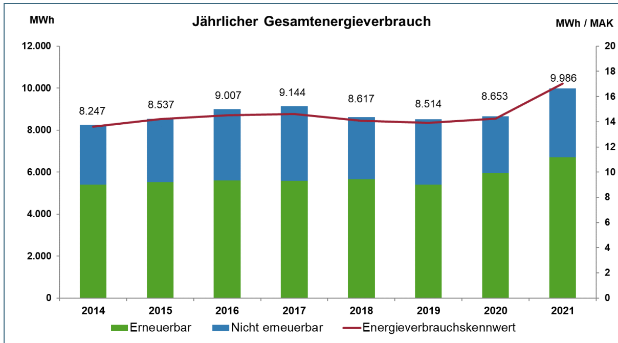
Abb. 11: Jährlicher Gesamtenergieverbrauch der Standorte Augsburg, Kulmbach und Wielenbach
