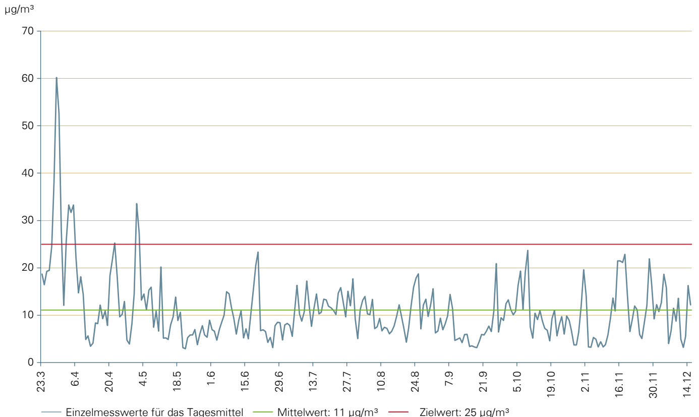
Verlauf der Feinstaub-Konzentration über den Messzeitraum vom 23. März bis 15. Dezember 2013: Einzelmesswerte für das Tagesmittel, der Mittelwert und der Zielwert über den gesamten Messzeitraum
