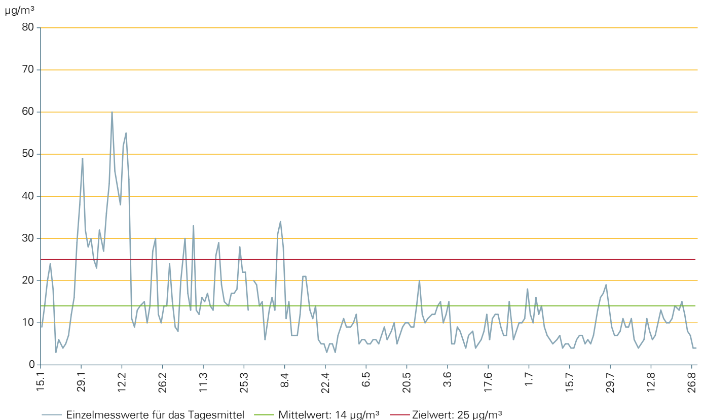
Verlauf der Feinstaub-Konzentration über den Messzeitraum vom 15. Januar bis 27. August 2012: Einzelmesswerte für das Tagesmittel, der Mittelwert und der Zielwert über den gesamten Messzeitraum
