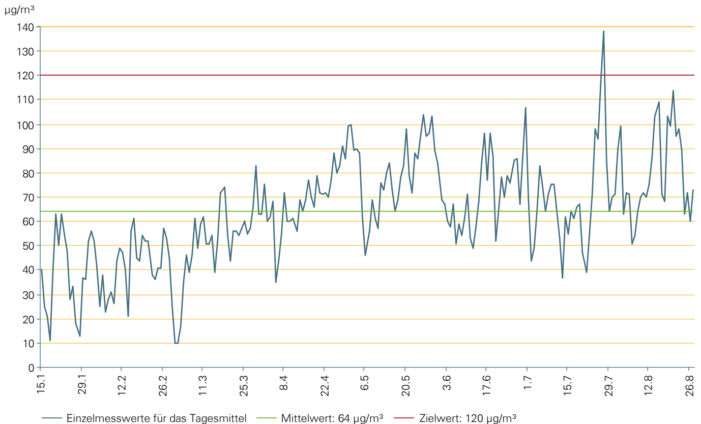
Verlauf der Ozon-Konzentration über den Messzeitraum vom 15. Januar bis 27. August 2012: Einzelmesswerte für das Tagesmittel, der Mittelwert und der Zielwert über den gesamten Messzeitraum
