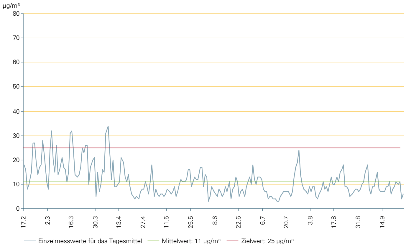
Verlauf der Feinstaub-Konzentration über den Messzeitraum vom 17. Februar bis 26. September 2012: Einzelmesswerte für das Tagesmittel, der Mittelwert und der Zielwert über den gesamten Messzeitraum
