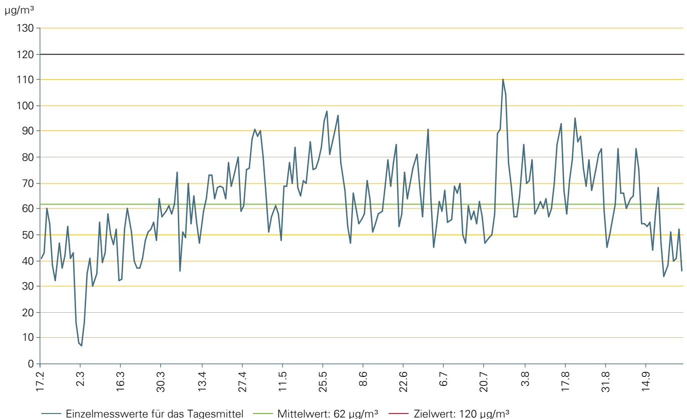
Verlauf der Ozon-Konzentration über den Messzeitraum über den Messzeitraum vom 17. Februar bis 26. September 2012: Einzelmesswerte für das Tagesmittel, der Mittelwert und der Zielwert über den gesamten Messzeitraum
