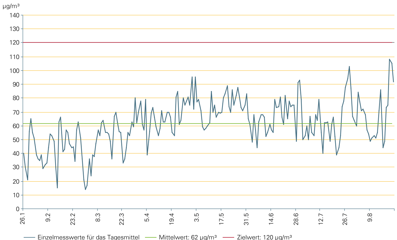
Verlauf der Ozon-Konzentration über den Messzeitraum vom 26. Januar bis 22. August 2012: Einzelmesswerte für das Tagesmittel, der Mittelwert und der Zielwert über den gesamten Messzeitraum
