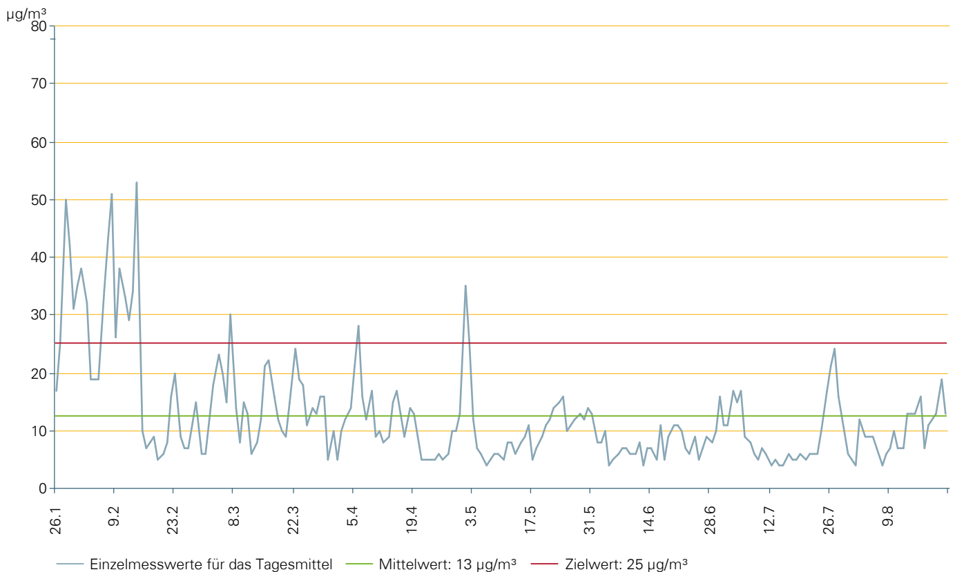
Verlauf der Feinstaub-Konzentration über den Messzeitraum vom 26. Januar bis 22. August 2012: Einzelmesswerte für das Tagesmittel, der Mittelwert und der Zielwert über den gesamten Messzeitraum
