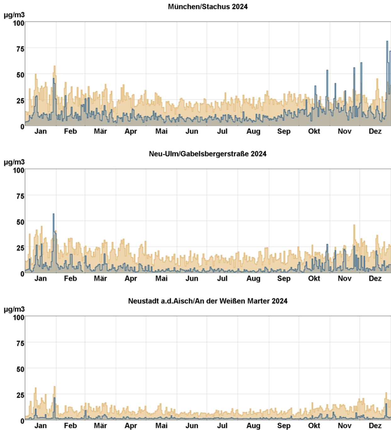
Abb. 11: Tagesmittelwertverläufe von Stickstoffmonoxid (blaue Stufenlinie) und Stickstoffdioxid (hellbraune Stufenlinie) an den mit Stickoxidmonitoren ausgestatteten LÜB-Messstationen.
