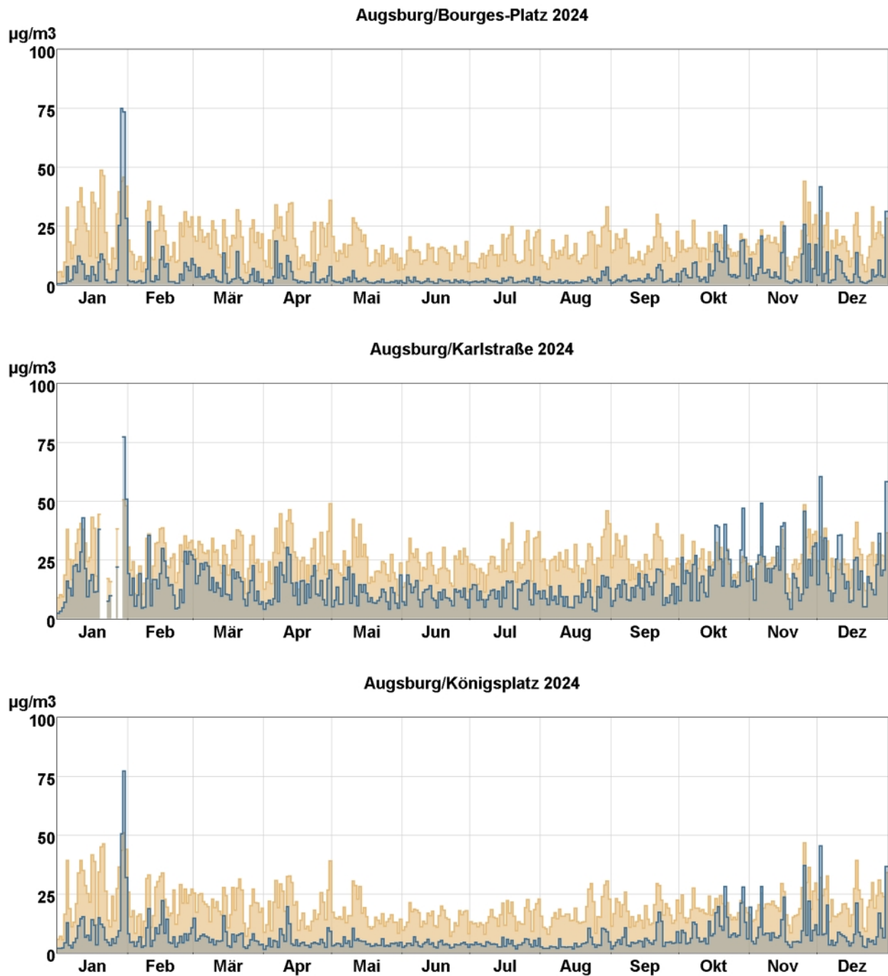
Abb. 3: Tagesmittelwertverläufe von Stickstoffmonoxid (blaue Stufenlinie) und Stickstoffdioxid (hellbraune Stufenlinie) an den mit Stickoxidmonitoren ausgestatteten LÜB-Messstationen.
