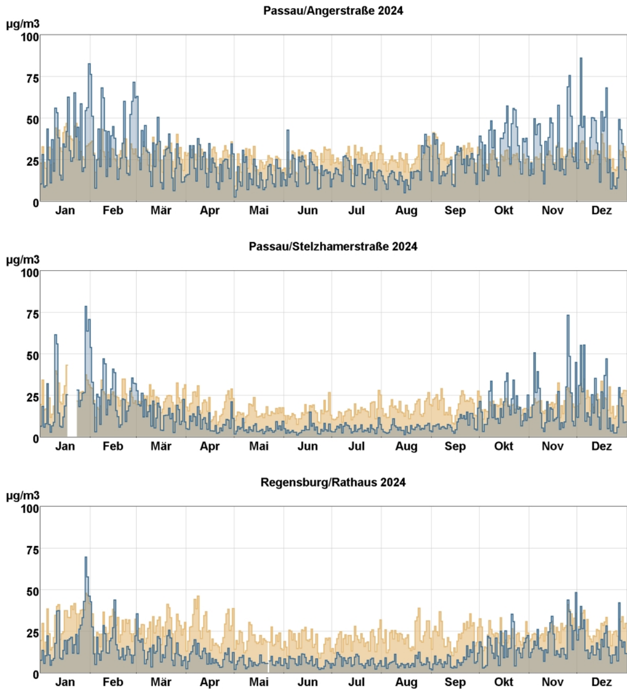
Abb. 14: Tagesmittelwertverläufe von Stickstoffmonoxid (blaue Stufenlinie) und Stickstoffdioxid (hellbraune Stufenlinie) an den mit Stickoxidmonitoren ausgestatteten LÜB-Messtationen.
