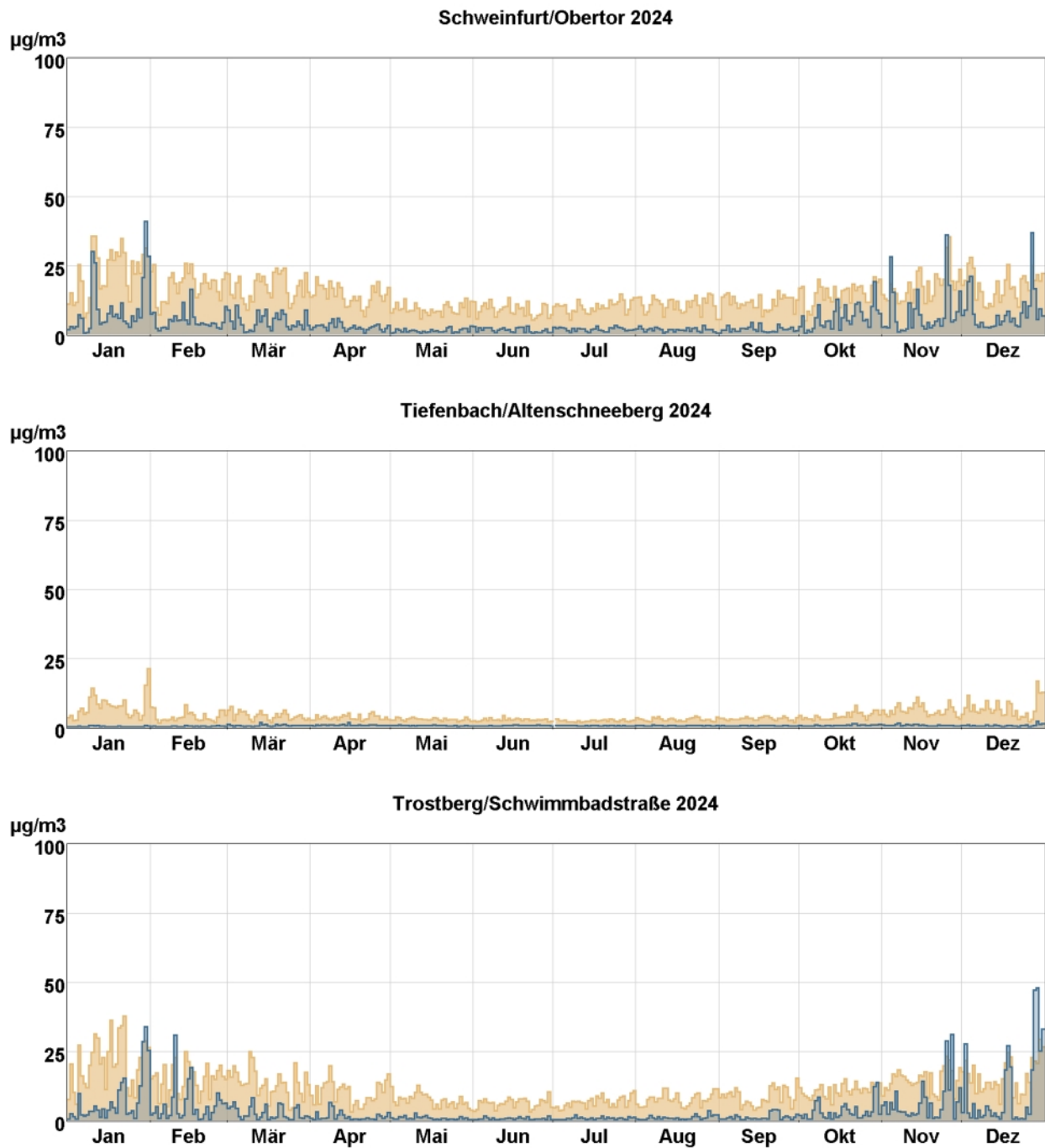
Abb. 16: Tagesmittelwertverläufe von Stickstoffmonoxid (blaue Stufenlinie) und Stickstoffdioxid (hellbraune Stufenlinie) an den mit Stickoxidmonitoren ausgestatteten LÜB-Messstationen.
