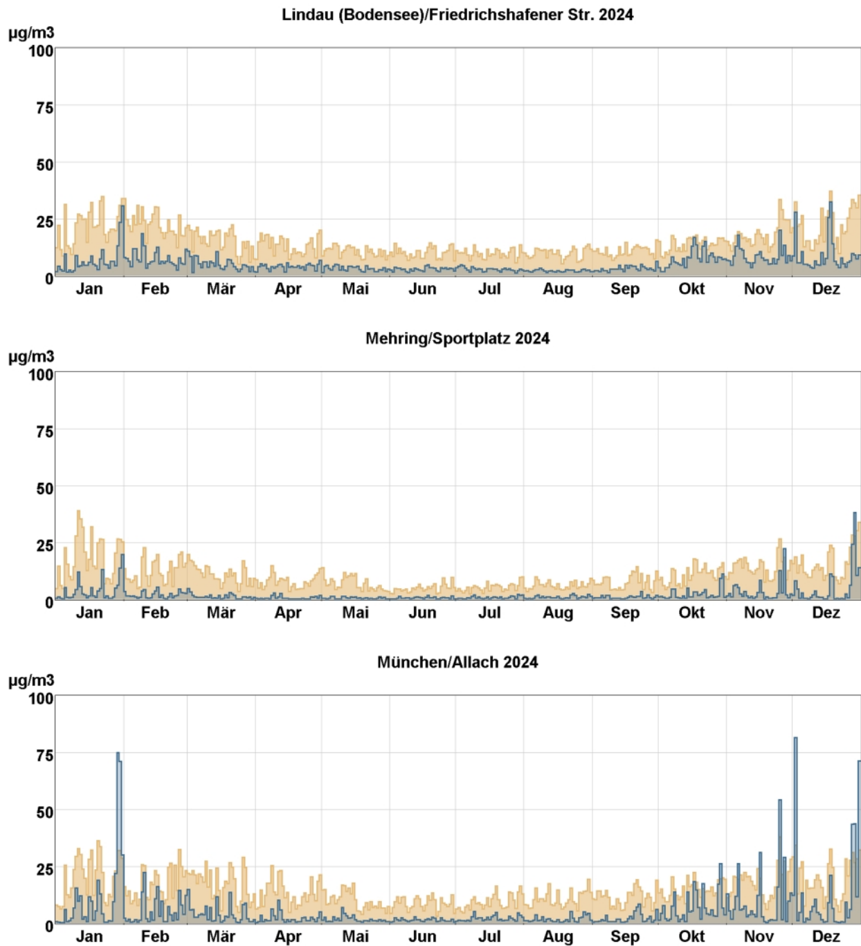
Abb. 9: Tagesmittelwertverläufe von Stickstoffmonoxid (blaue Stufenlinie) und Stickstoffdioxid (hellbraune Stufenlinie) an den mit Stickoxidmonitoren ausgestatteten LÜB-Messstationen.
