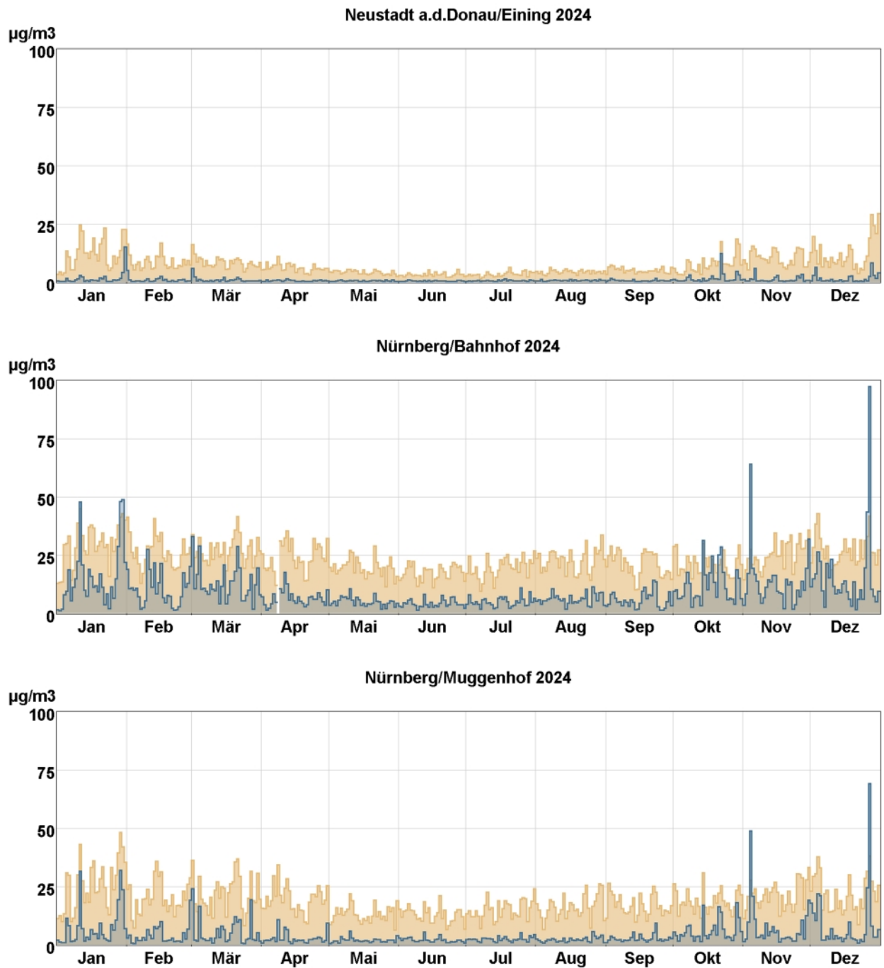
Abb. 12: Tagesmittelwertverläufe von Stickstoffmonoxid (blaue Stufenlinie) und Stickstoffdioxid (hellbraune Stufenlinie) an den mit Stickoxidmonitoren ausgestatteten LÜB-Messstationen.
