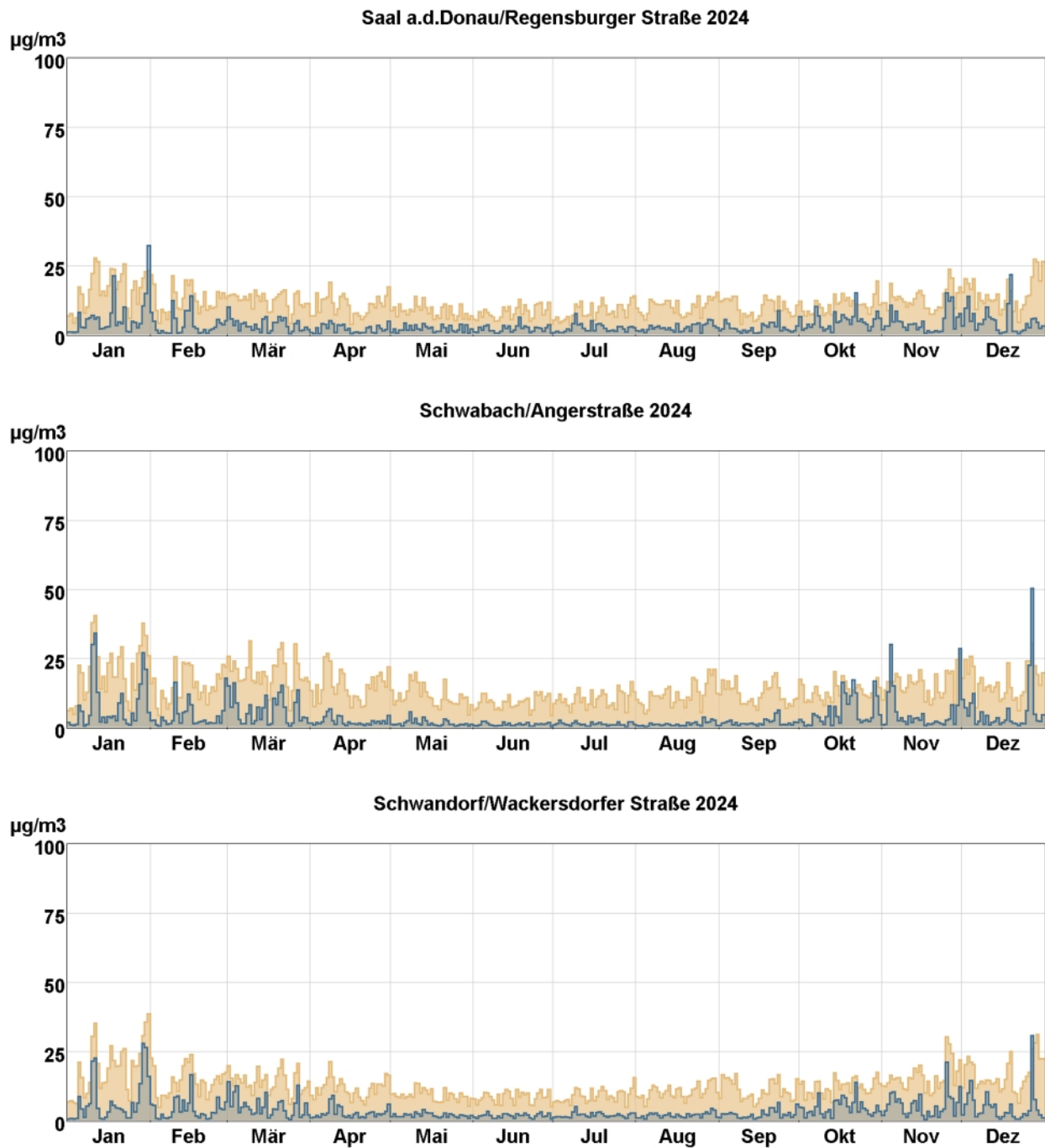
Abb. 15: Tagesmittelwertverläufe von Stickstoffmonoxid (blaue Stufenlinie) und Stickstoffdioxid (hellbraune Stufenlinie) an den mit Stickoxidmonitoren ausgestatteten LÜB-Messstationen.
