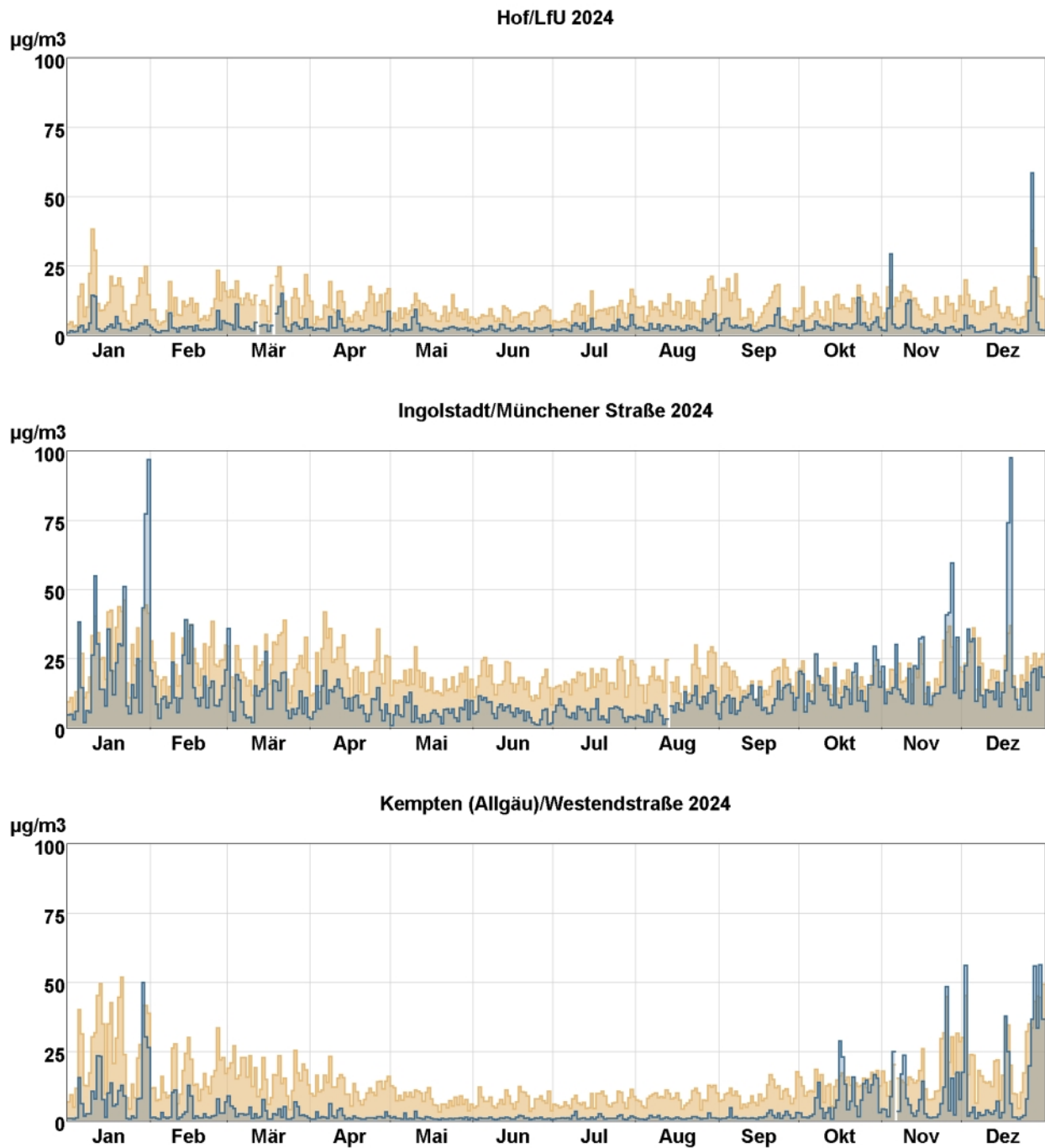
Abb. 7: Tagesmittelwertverläufe von Stickstoffmonoxid (blaue Stufenlinie) und Stickstoffdioxid (hellbraune Stufenlinie) an den mit Stickoxidmonitoren ausgestatteten LÜB-Messstationen.
