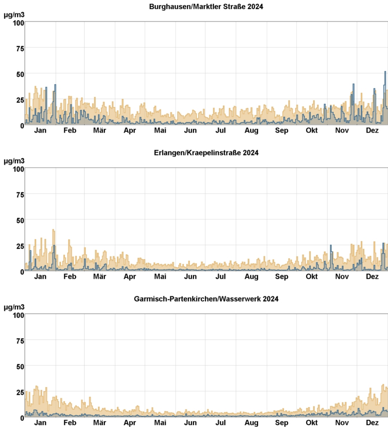
Abb. 6: Tagesmittelwertverläufe von Stickstoffmonoxid (blaue Stufenlinie) und Stickstoffdioxid (hellbraune Stufenlinie) an den mit Stickoxidmonitoren ausgestatteten LÜB-Messstationen.
