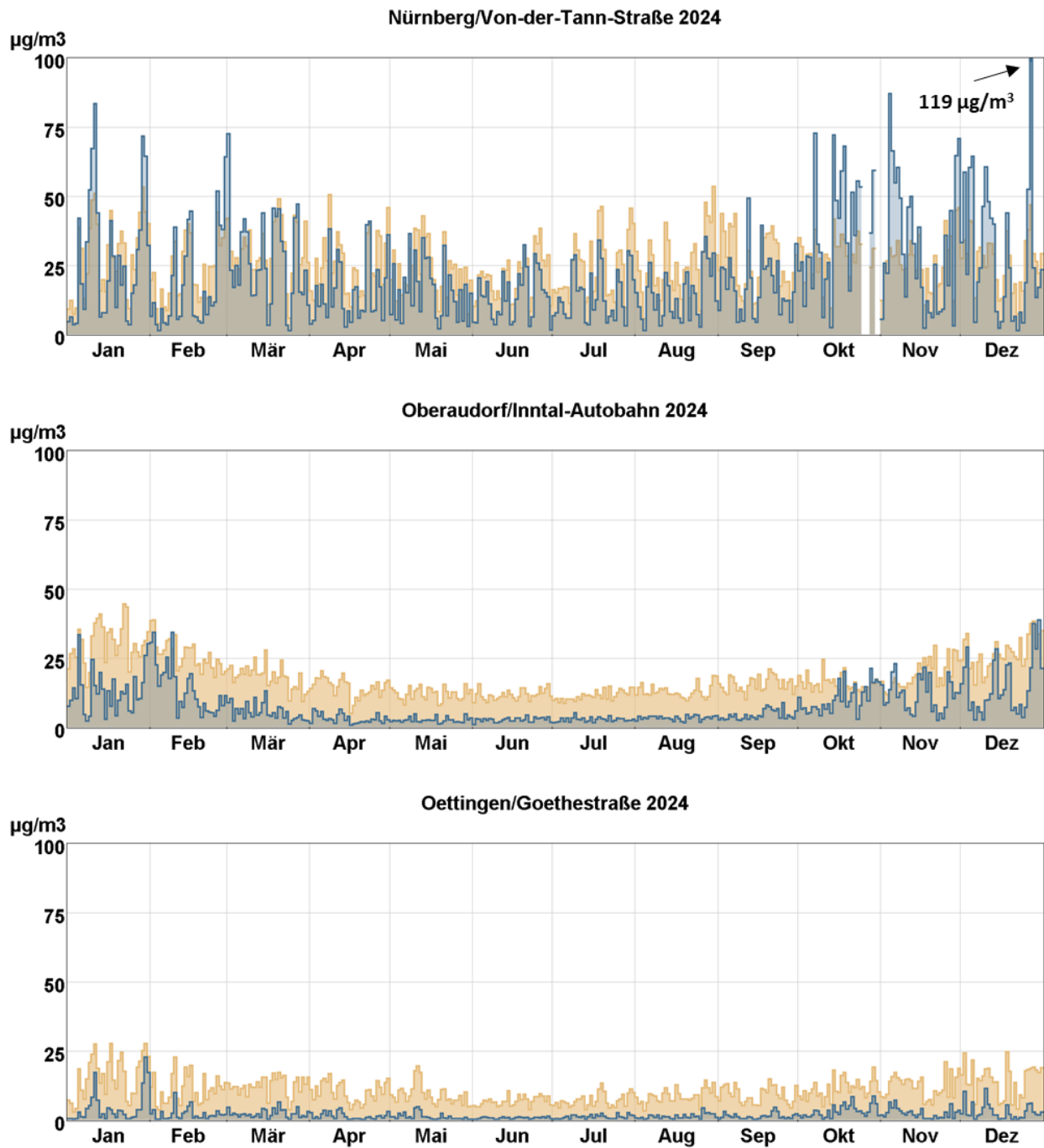
Abb. 13: Tagesmittelwertverläufe von Stickstoffmonoxid (blaue Stufenlinie) und Stickstoffdioxid (hellbraune Stufenlinie) an den mit Stickoxidmonitoren ausgestatteten LÜB-Messstationen.
