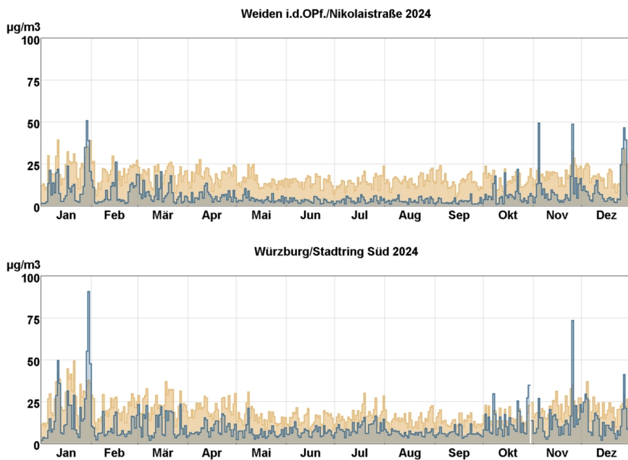
Abb. 17: Tagesmittelwertverläufe von Stickstoffmonoxid (blaue Stufenlinie) und Stickstoffdioxid (hellbraune Stufenlinie) an den mit Stickoxidmonitoren ausgestatteten LÜB-Messstationen.
