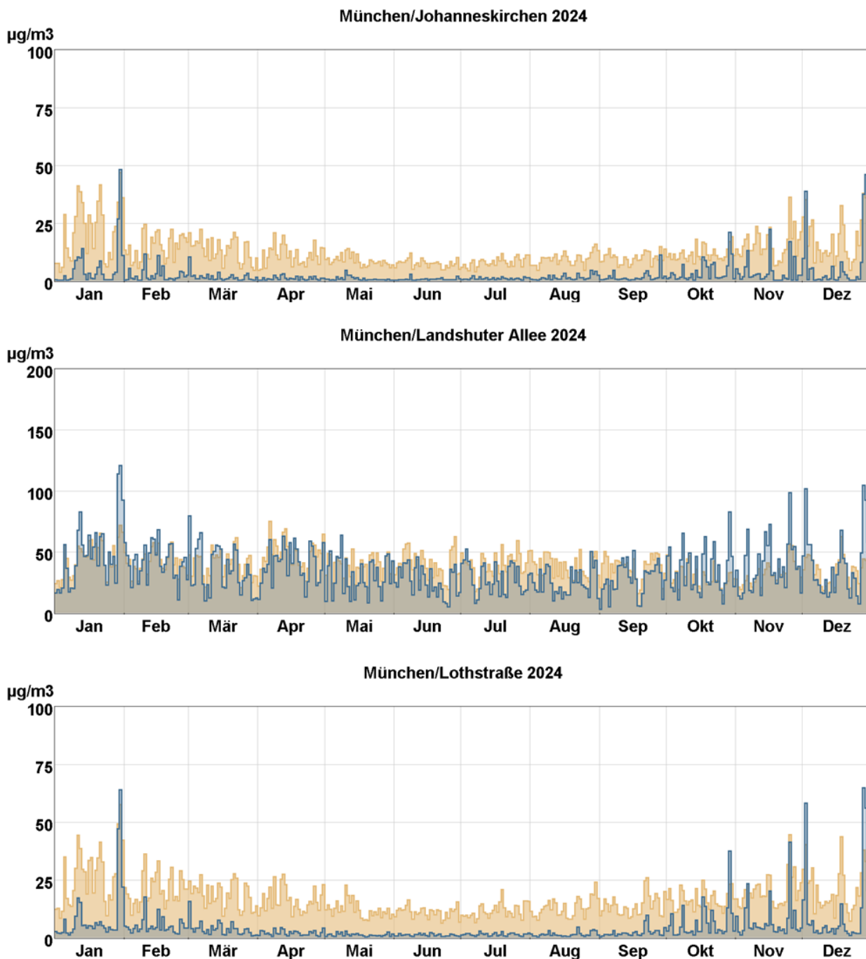
Abb. 10: Tagesmittelwertverläufe von Stickstoffmonoxid (blaue Stufenlinie) und Stickstoffdioxid (hellbraune Stufenlinie) an den mit Stickoxidmonitoren ausgestatteten LÜB-Messstationen.
