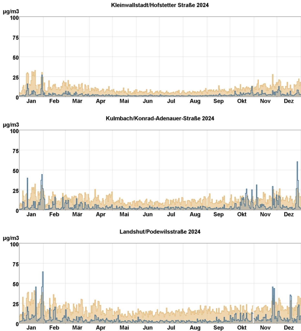
Abb. 8: Tagesmittelwertverläufe von Stickstoffmonoxid (blaue Stufenlinie) und Stickstoffdioxid (hellbraune Stufenlinie) an den mit Stickoxidmonitoren ausgestatteten LÜB-Messstationen.
