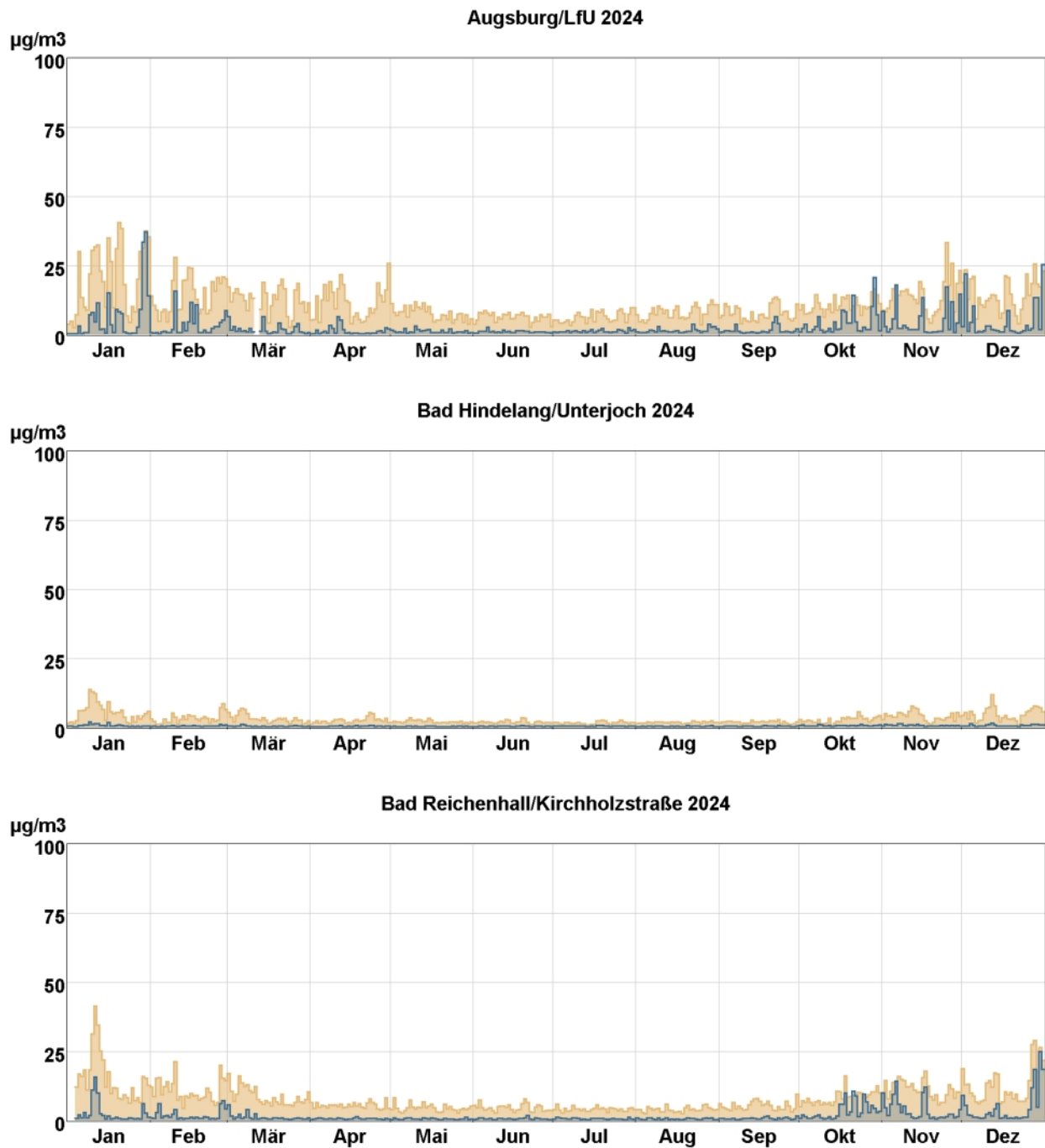
Abb. 4: Tagesmittelwertverläufe von Stickstoffmonoxid (blaue Stufenlinie) und Stickstoffdioxid (hellbraune Stufenlinie) an den mit Stickoxidmonitoren ausgestatteten LÜB-Messstationen.
