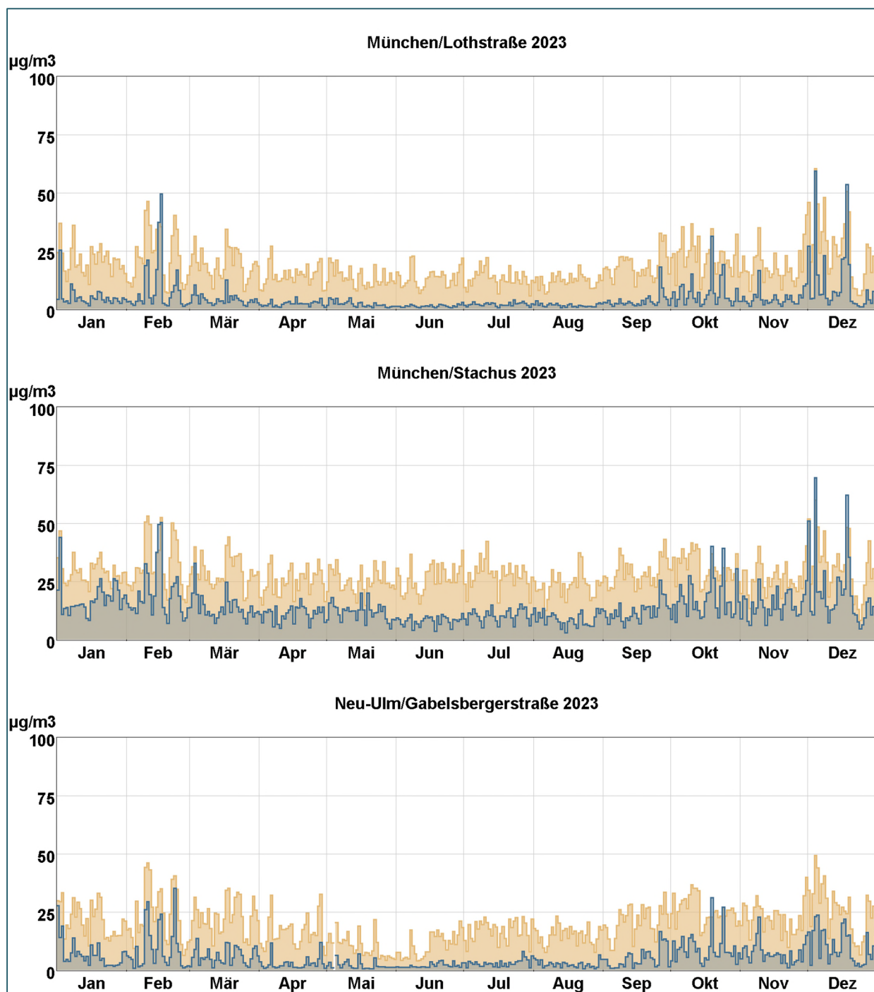
Abb. 11: Tagesmittelwertverläufe von Stickstoffmonoxid (blaue Stufenlinie) und Stickstoffdioxid (hellbraune Stufenlinie) an den mit Stickoxidmonitoren ausgestatteten LÜB-Messstationen.
