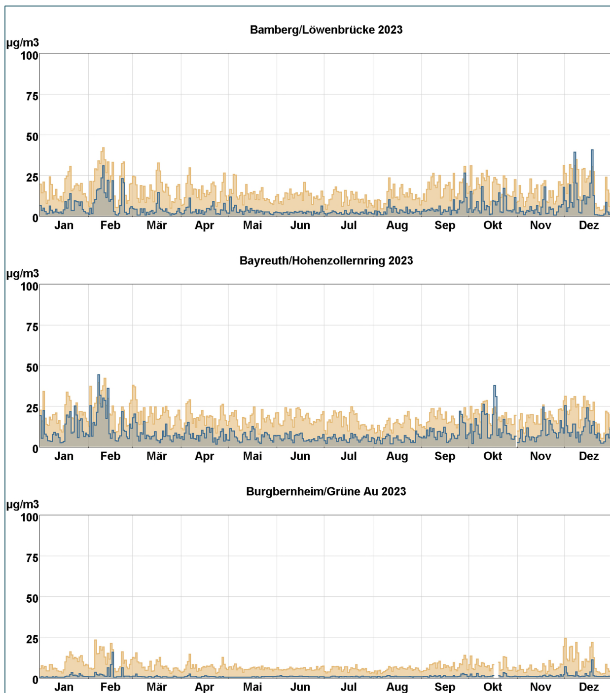
Abb. 5: Tagesmittelwertverläufe von Stickstoffmonoxid (blaue Stufenlinie) und Stickstoffdioxid (hellbraune Stufenlinie) an den mit Stickoxidmonitoren ausgestatteten LÜB-Messstationen.
