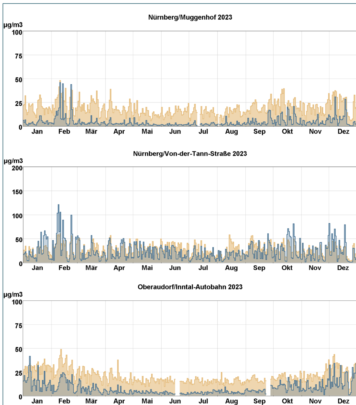
Abb. 13: Tagesmittelwertverläufe von Stickstoffmonoxid (blaue Stufenlinie) und Stickstoffdioxid (hellbraune Stufenlinie) an den mit Stickoxidmonitoren ausgestatteten LÜB-Messstationen.
