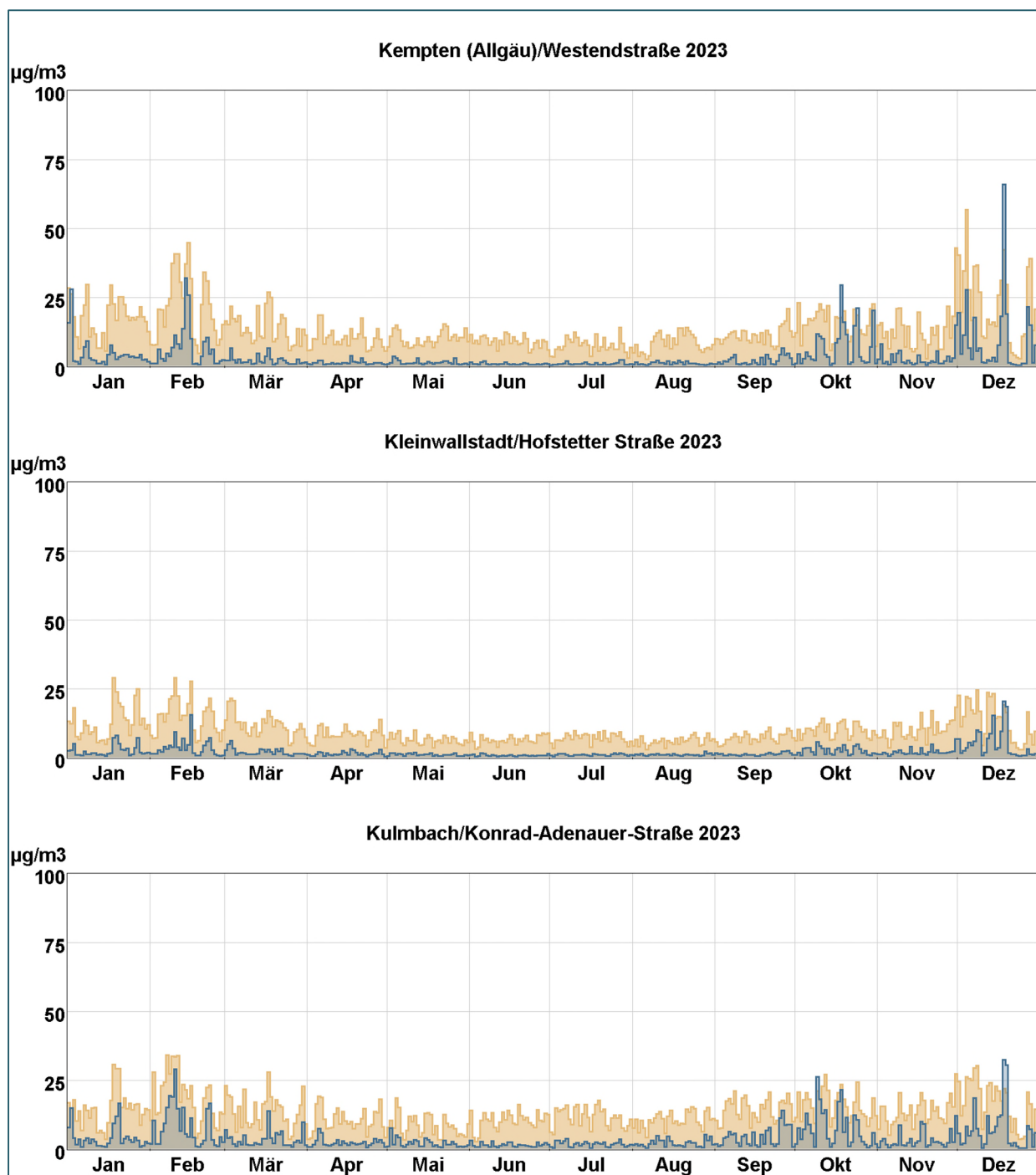
Abb. 8: Tagesmittelwertverläufe von Stickstoffmonoxid (blaue Stufenlinie) und Stickstoffdioxid (hellbraune Stufenlinie) an den mit Stickoxidmonitoren ausgestatteten LÜB-Messstationen.
