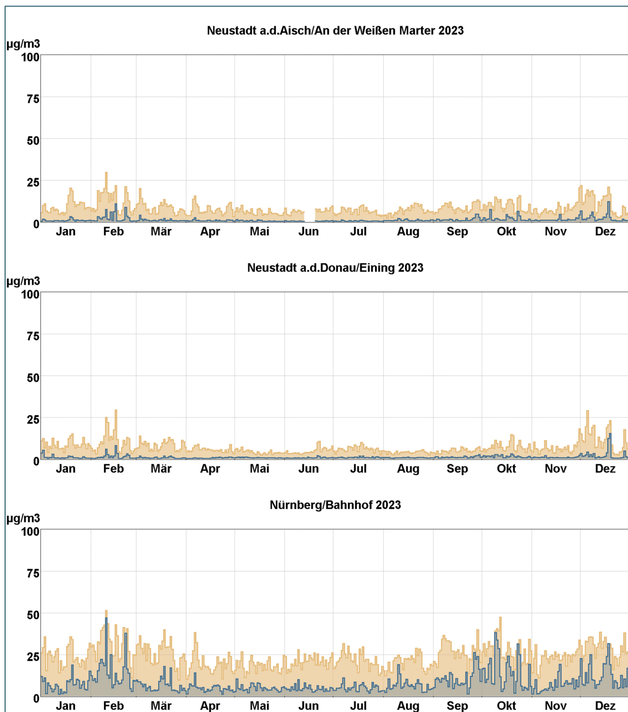
Abb. 12: Tagesmittelwertverläufe von Stickstoffmonoxid (blaue Stufenlinie) und Stickstoffdioxid (hellbraune Stufenlinie) an den mit Stickoxidmonitoren ausgestatteten LÜB-Messstationen.
