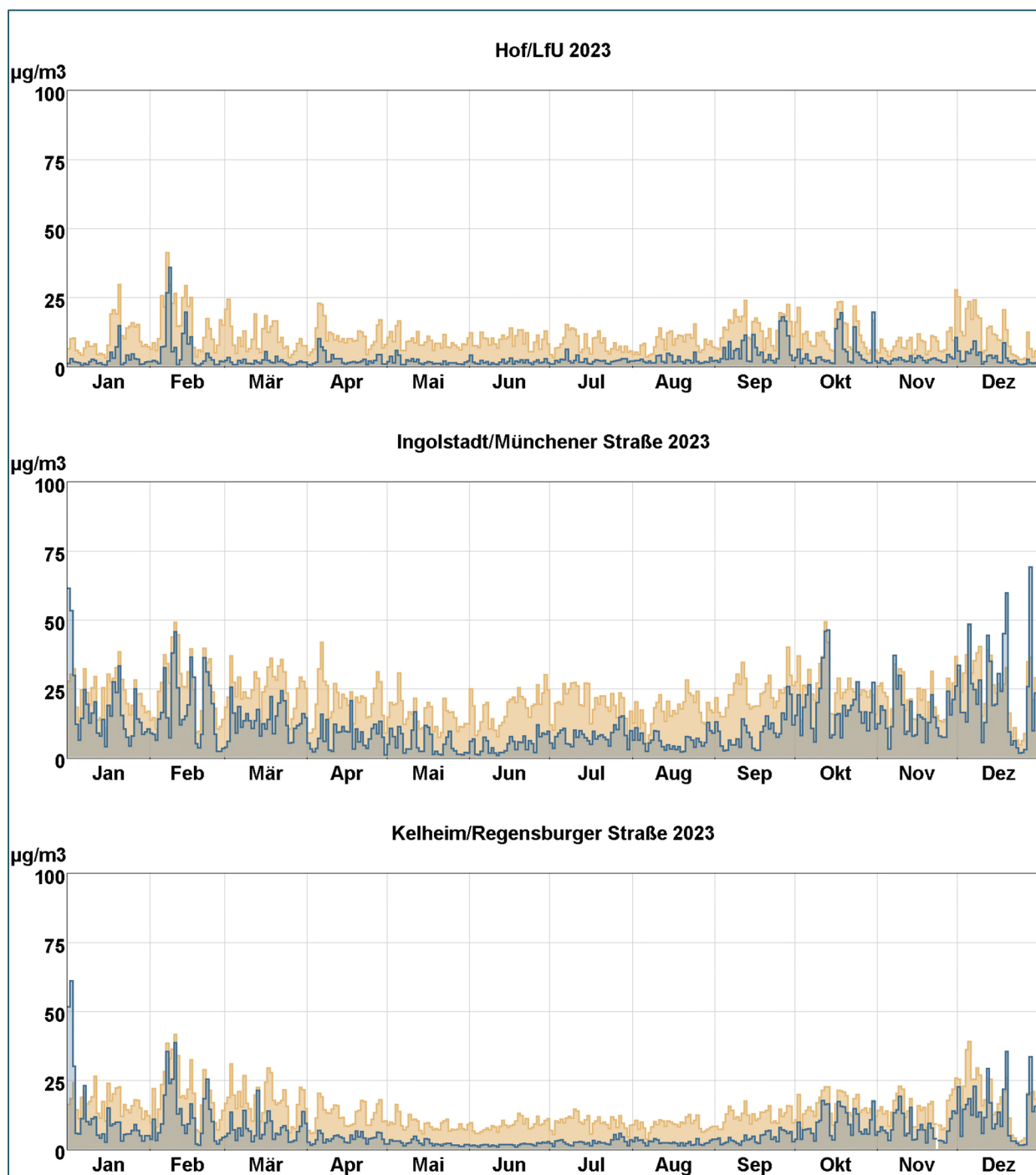
Abb. 7: Tagesmittelwertverläufe von Stickstoffmonoxid (blaue Stufenlinie) und Stickstoffdioxid (hellbraune Stufenlinie) an den mit Stickoxidmonitoren ausgestatteten LÜB-Messstationen.
