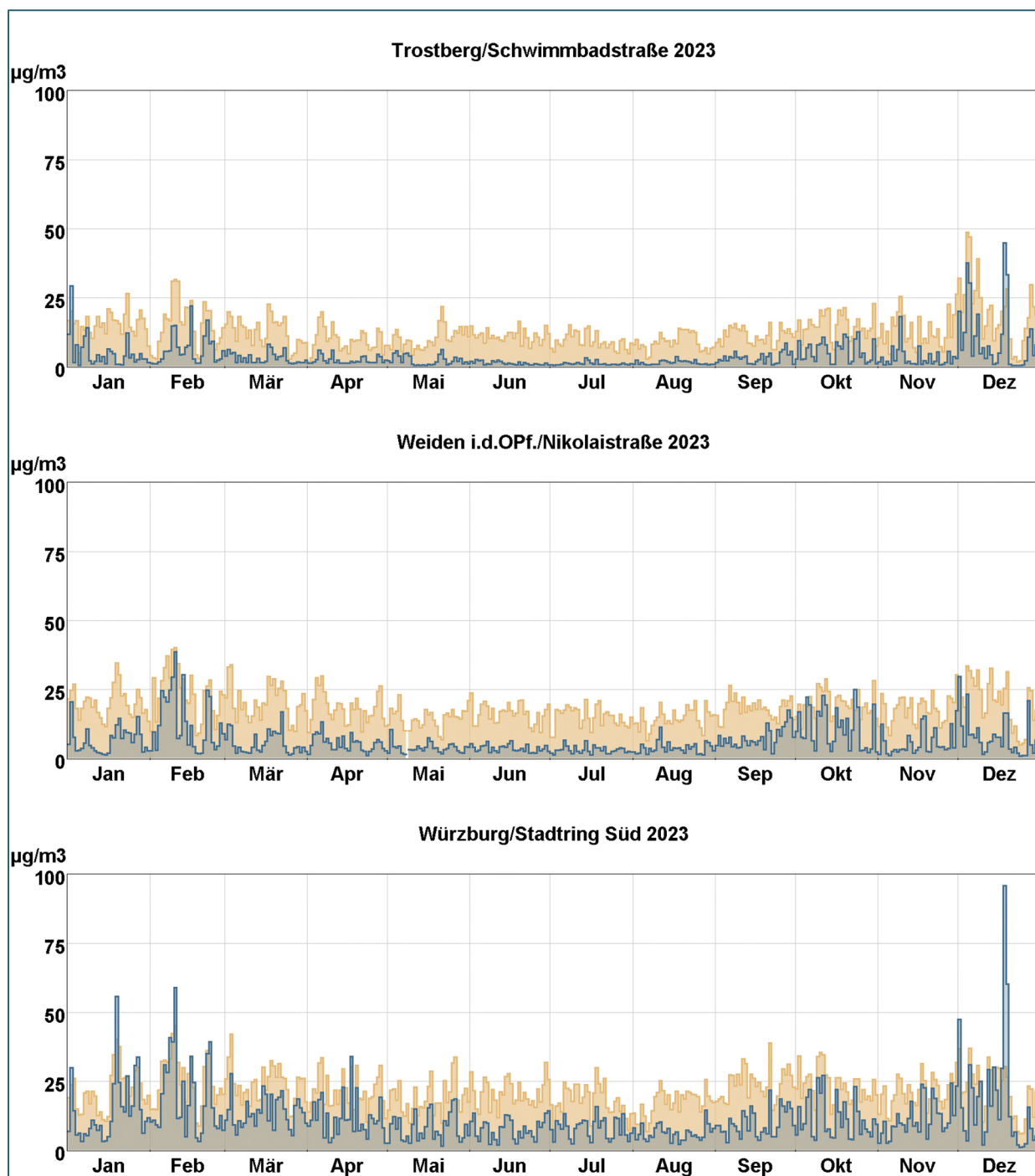
Abb. 17: Tagesmittelwertverläufe von Stickstoffmonoxid (blaue Stufenlinie) und Stickstoffdioxid (hellbraune Stufenlinie) an den mit Stickoxidmonitoren ausgestatteten LÜB-Messstationen.
