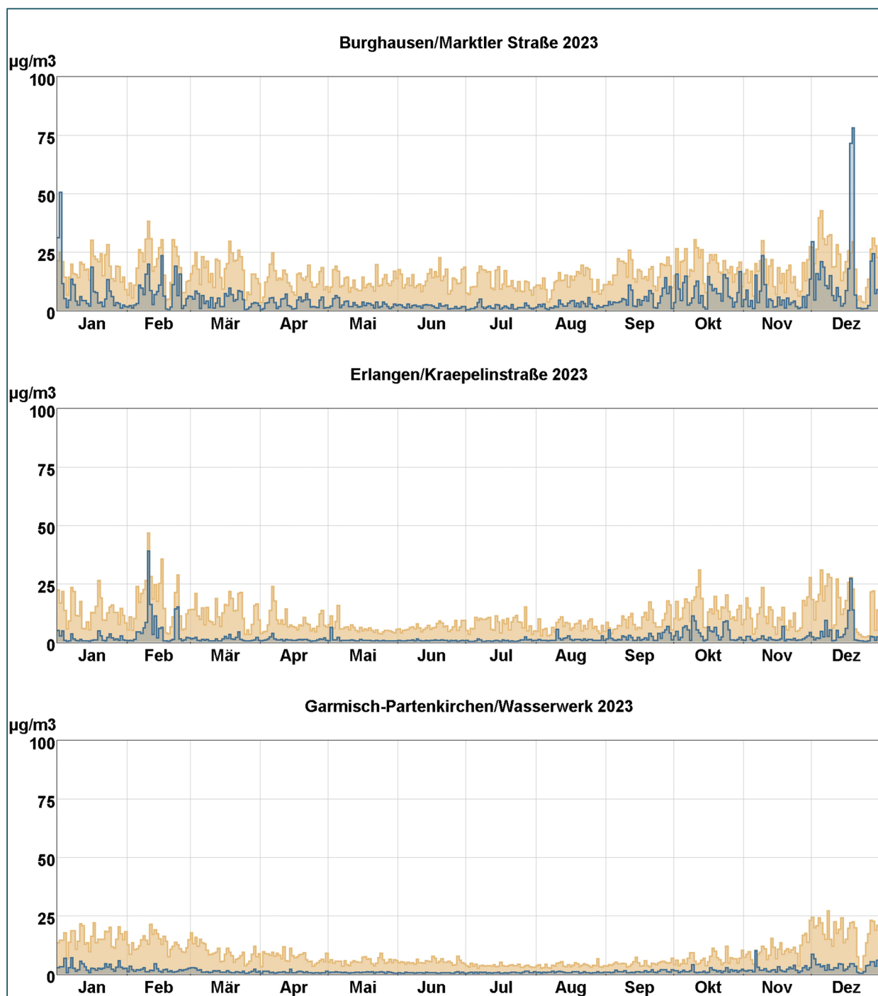
Abb. 6: Tagesmittelwertverläufe von Stickstoffmonoxid (blaue Stufenlinie) und Stickstoffdioxid (hellbraune Stufenlinie) an den mit Stickoxidmonitoren ausgestatteten LÜB-Messstationen.
