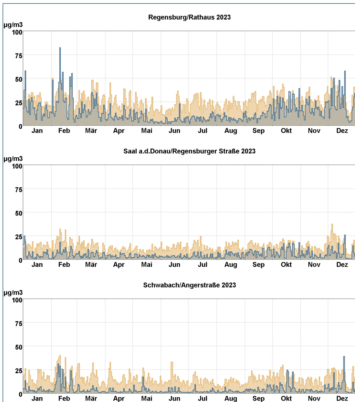
Abb. 15: Tagesmittelwertverläufe von Stickstoffmonoxid (blaue Stufenlinie) und Stickstoffdioxid (hellbraune Stufenlinie) an den mit Stickoxidmonitoren ausgestatteten LÜB-Messstationen.
