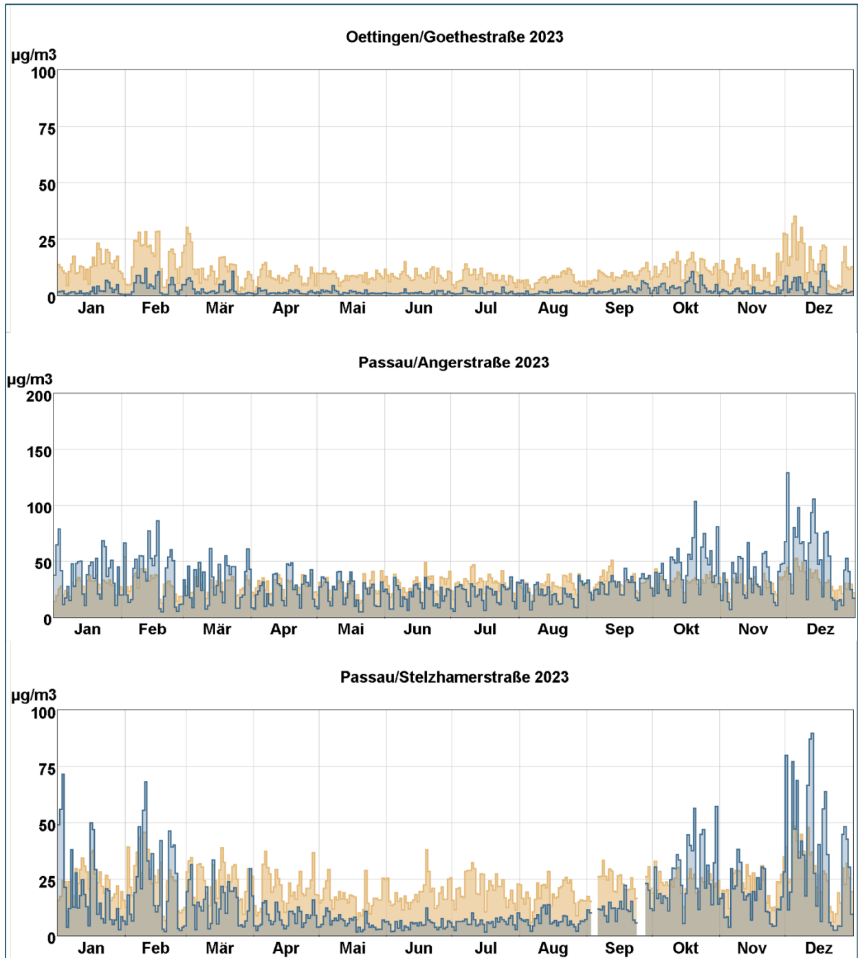
Abb. 14: Tagesmittelwertverläufe von Stickstoffmonoxid (blaue Stufenlinie) und Stickstoffdioxid (hellbraune Stufenlinie) an den mit Stickoxidmonitoren ausgestatteten LÜB-Messstationen.
