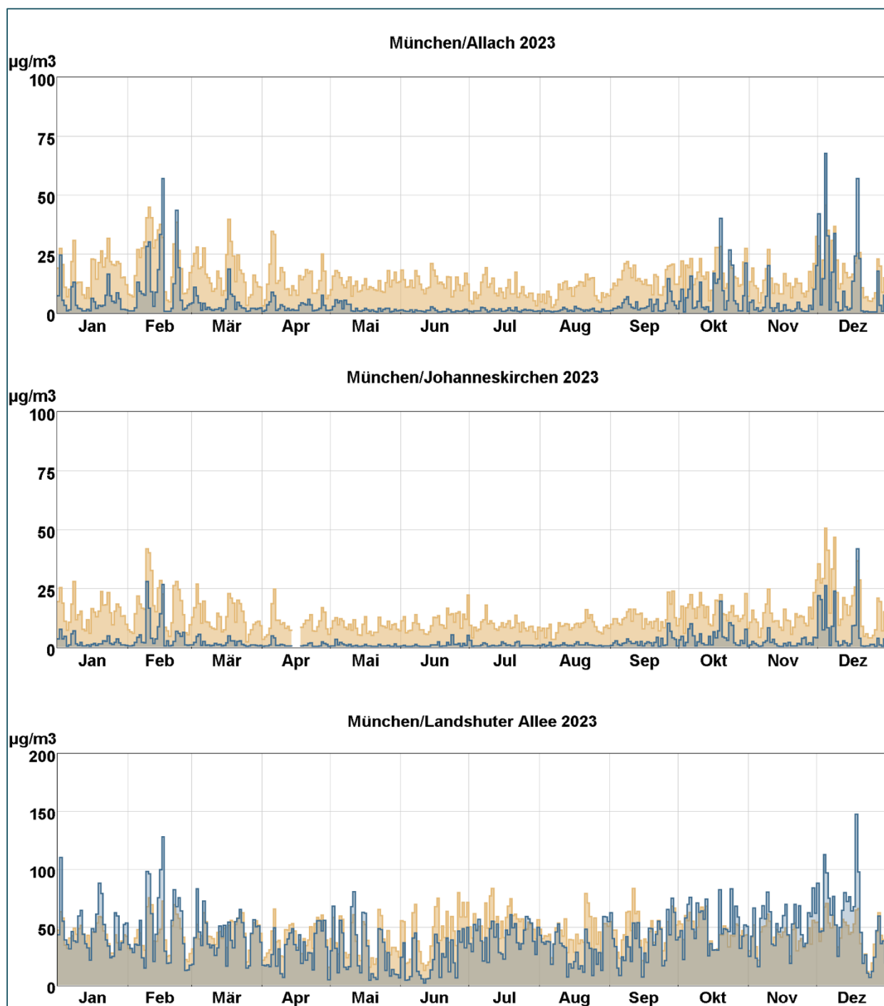
Abb. 10: Tagesmittelwertverläufe von Stickstoffmonoxid (blaue Stufenlinie) und Stickstoffdioxid (hellbraune Stufenlinie) an den mit Stickoxidmonitoren ausgestatteten LÜB-Messstationen.
