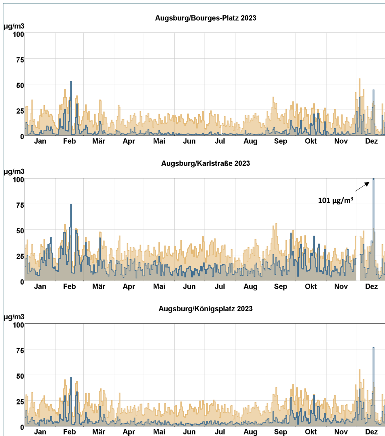
Abb. 3: Tagesmittelwertverläufe von Stickstoffmonoxid (blaue Stufenlinie) und Stickstoffdioxid (hellbraune Stufenlinie) an den mit Stickoxidmonitoren ausgestatteten LÜB-Messstationen.
