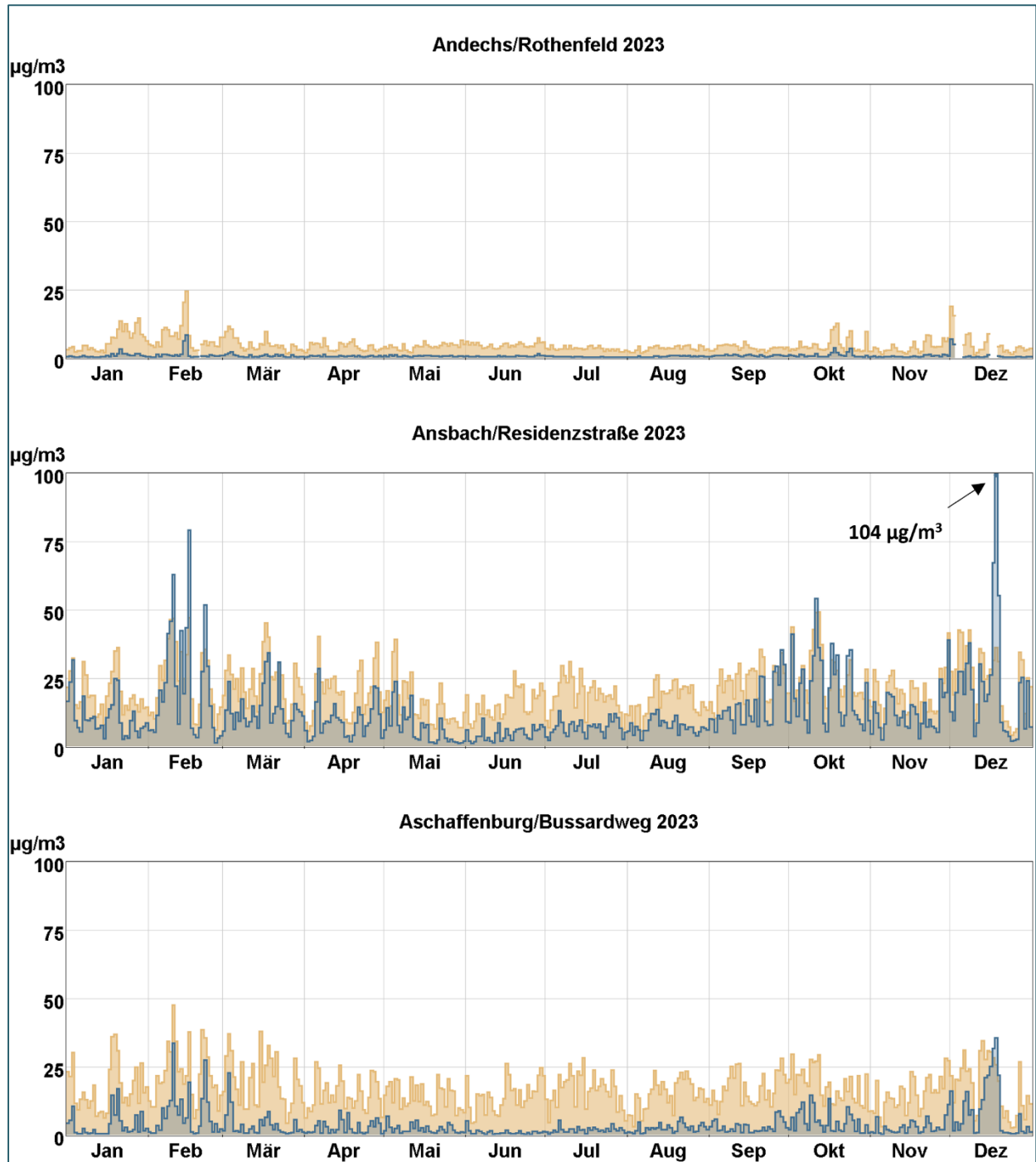
Abb. 2: Tagesmittelwertverläufe von Stickstoffmonoxid (blaue Stufenlinie) und Stickstoffdioxid (hellbraune Stufenlinie) an den mit Stickoxidmonitoren ausgestatteten LÜB-Messstationen.
