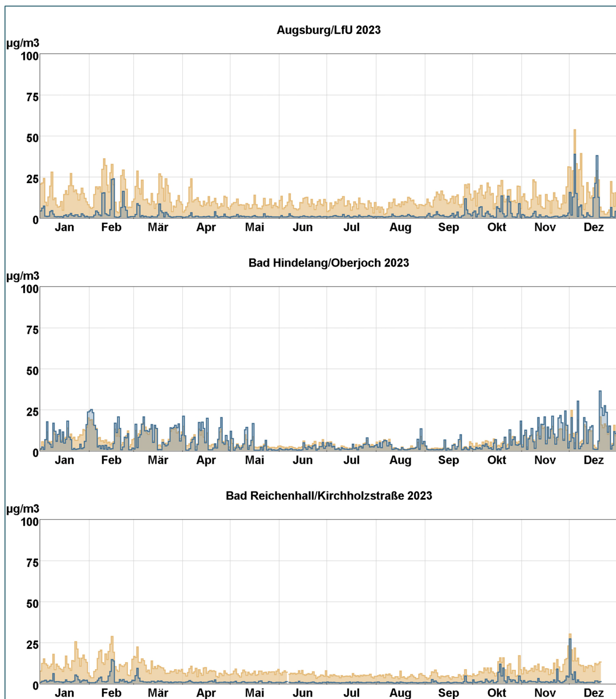
Abb. 4: Tagesmittelwertverläufe von Stickstoffmonoxid (blaue Stufenlinie) und Stickstoffdioxid (hellbraune Stufenlinie) an den mit Stickoxidmonitoren ausgestatteten LÜB-Messstationen.
