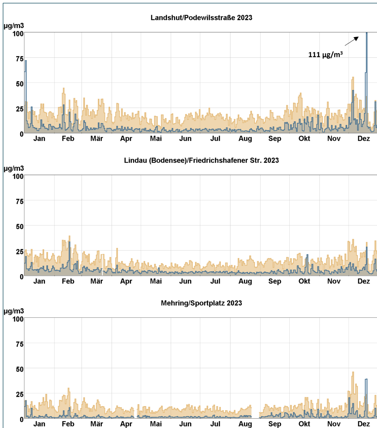
Abb. 9: Tagesmittelwertverläufe von Stickstoffmonoxid (blaue Stufenlinie) und Stickstoffdioxid (hellbraune Stufenlinie) an den mit Stickoxidmonitoren ausgestatteten LÜB-Messstationen.
