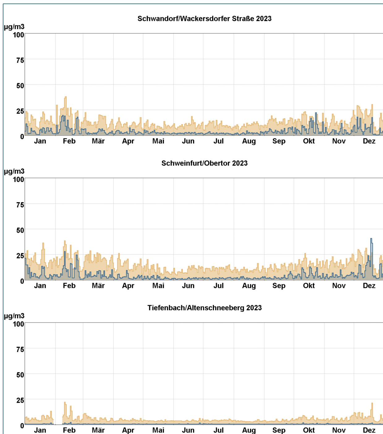
Abb. 16: Tagesmittelwertverläufe von Stickstoffmonoxid (blaue Stufenlinie) und Stickstoffdioxid (hellbraune Stufenlinie) an den mit Stickoxidmonitoren ausgestatteten LÜB-Messstationen.
