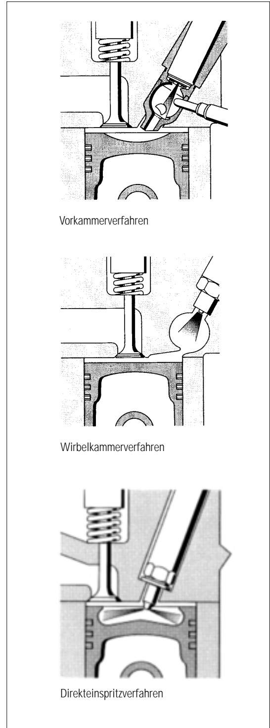
Abb. 4: Verbrennungsverfahren (Quelle: Bosch GmbH)
