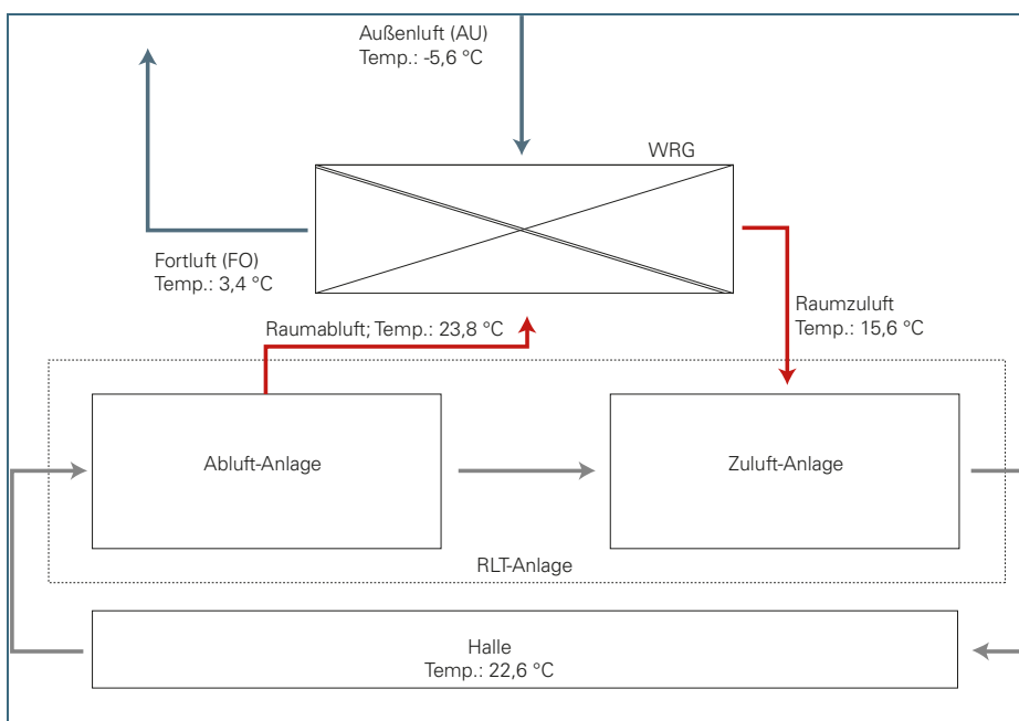
Abb. 6: Mithilfe der Wärmerückgewinnung aus der Raumabluft (23,8 °C) wird die Außenluft auf 15,6 °C angewärmt.
