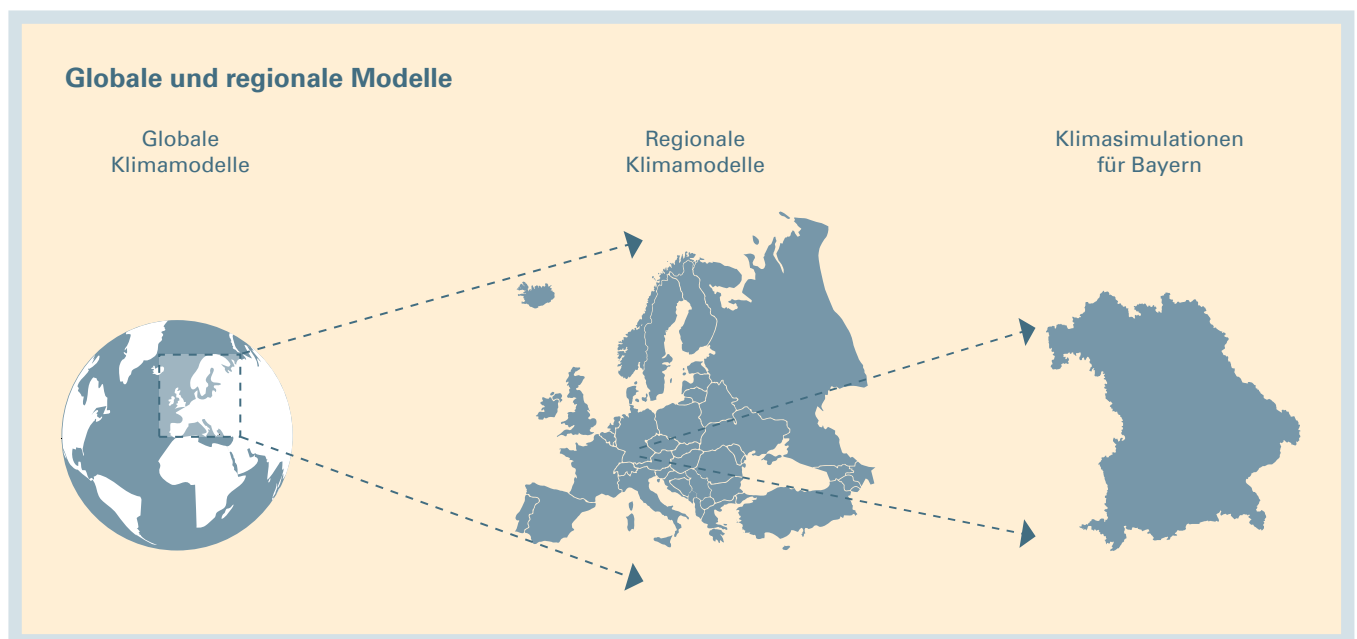
Abb. 6: Um sich vor Ort wirksam an den Klimawandel anzupassen, sind regio- nal spezifische Aussagen notwendig. Dazu werden mehrere Modelle kombiniert, um auch regionale Be- sonderheiten zu berücksichtigen.
