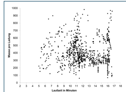
Abb. 10: In unbelastetem Grundwasser können wie in diesem Fall rund 1.000 Signale gemessen werden. Jedes Signal entspricht einer Substanz, die meisten sind unbekannt.
