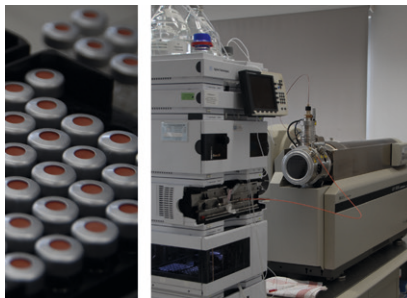
Abb. 8: Die Wasserproben werden in kleine Fläschchen abgefüllt und mit dem LC-MS-Gerät analysiert.
