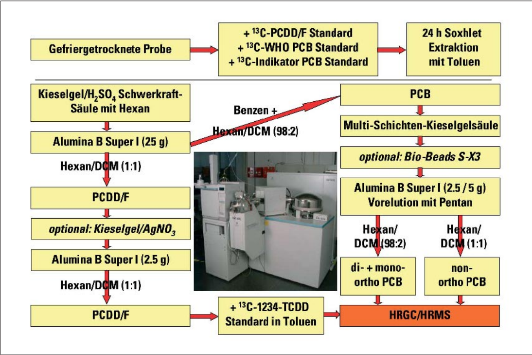
Abb. 1: Probenvorbereitung zur Bestimmung der PCDD/PCDF und PCB
