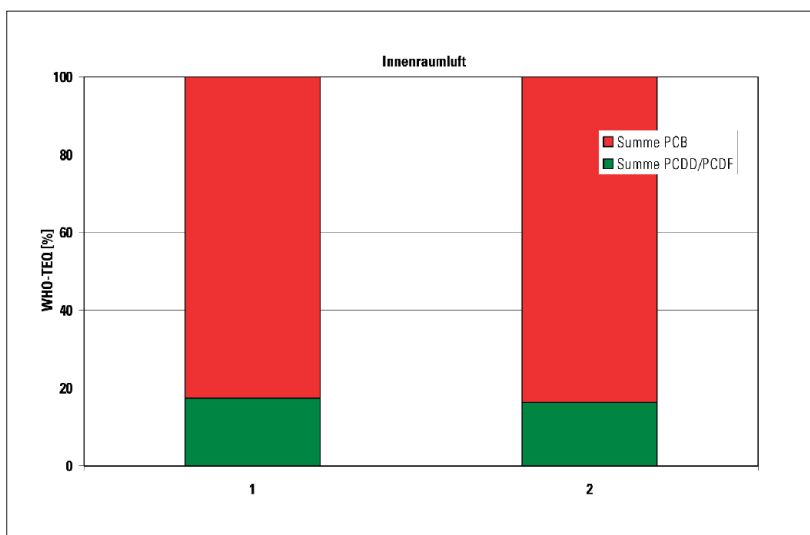
Abb. 20: TEQ-Beitrag der PCB zum Gesamtoxitätsäquivalent in belasteten Innenräumen
