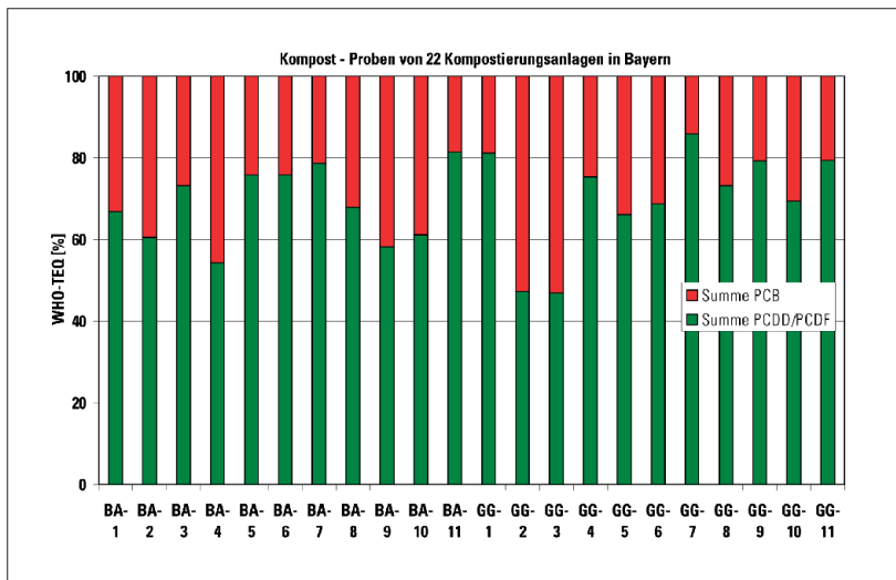
Abb. 14: TEQ Verteilung auf PCB und PCDD/PCDF Kompostproben von 22 bayerischen Kompostierungsanlagen 2002 – 1. Beprobung
