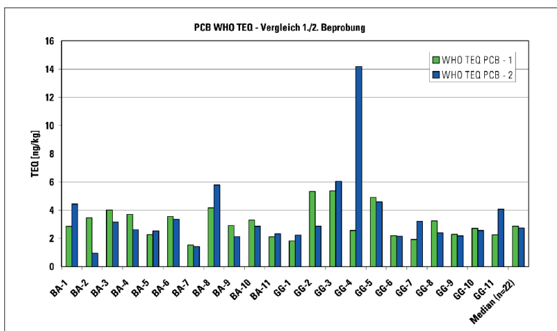
Abb. 15: Vergleich der PCB WHO TEQ der beiden Probenahmen an 22 bayerischen Kompostierungsanlagen 2002
