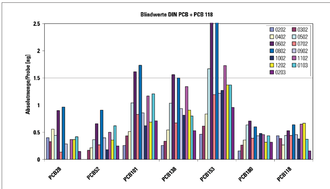
Abb. 4: Laborblindwerte [ng/Probe] der Indikator-kongener und von PCB 118 von Februar 2002 bis Februar 2003
