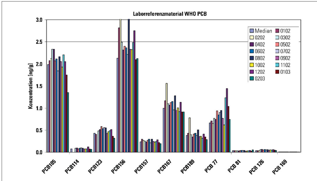
Abb. 3: Konzentrationen der dioxinähnlichen PCB im Klärschlammreferenzmaterial – Aufarbeitungen Januar 2002 – Februar 2003
