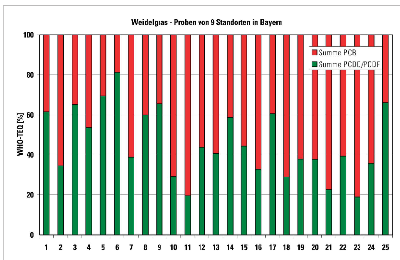
Abb. 11: TEQ Verteilung auf PCB und PCDD/PCDF in den Weidelgrasproben 2001
