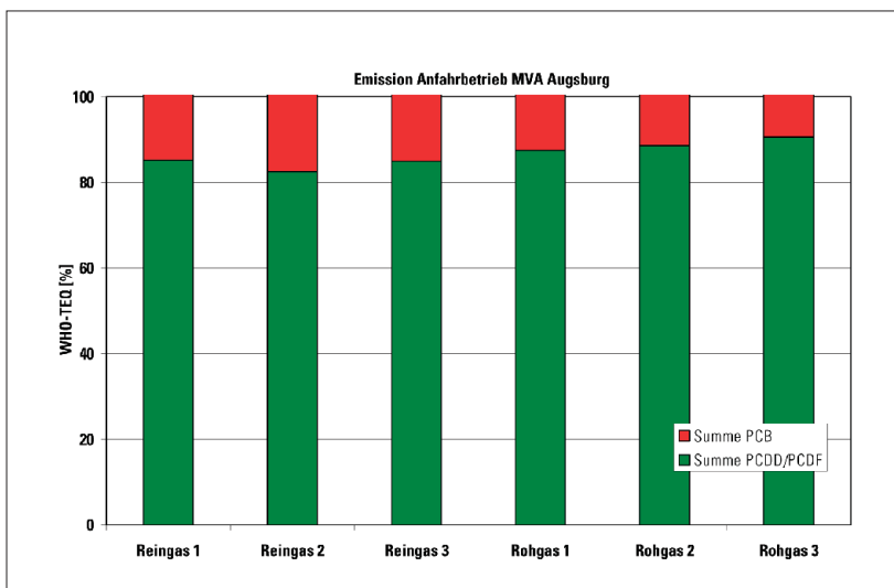
Abb. 18: TEQ Beitrag der PCB und PCDD/PCDF in Emissionsproben der MVA Augsburg im Anfahrbetrieb
