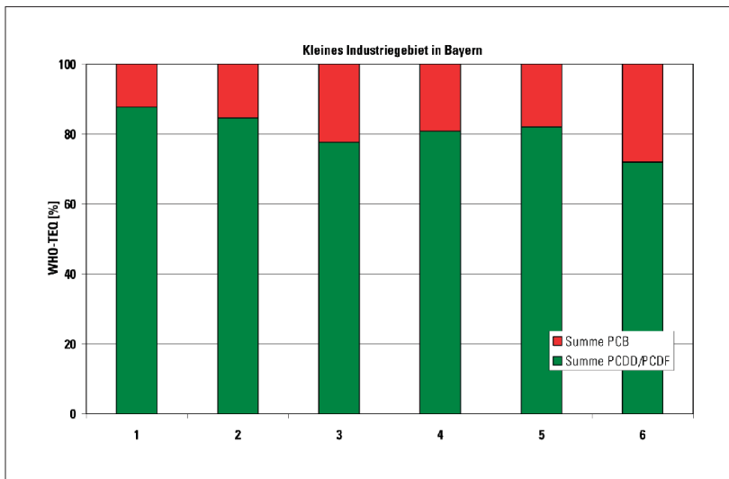
Abb. 17: TEQ Beitrag der PCB und PCDD/PCDF in Außenluftproben
