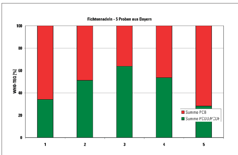
Abb. 13: TEQ Verteilung auf PCB und PCDD/PCDF in Fichtennadeln der Herbstbeprobung 2001
