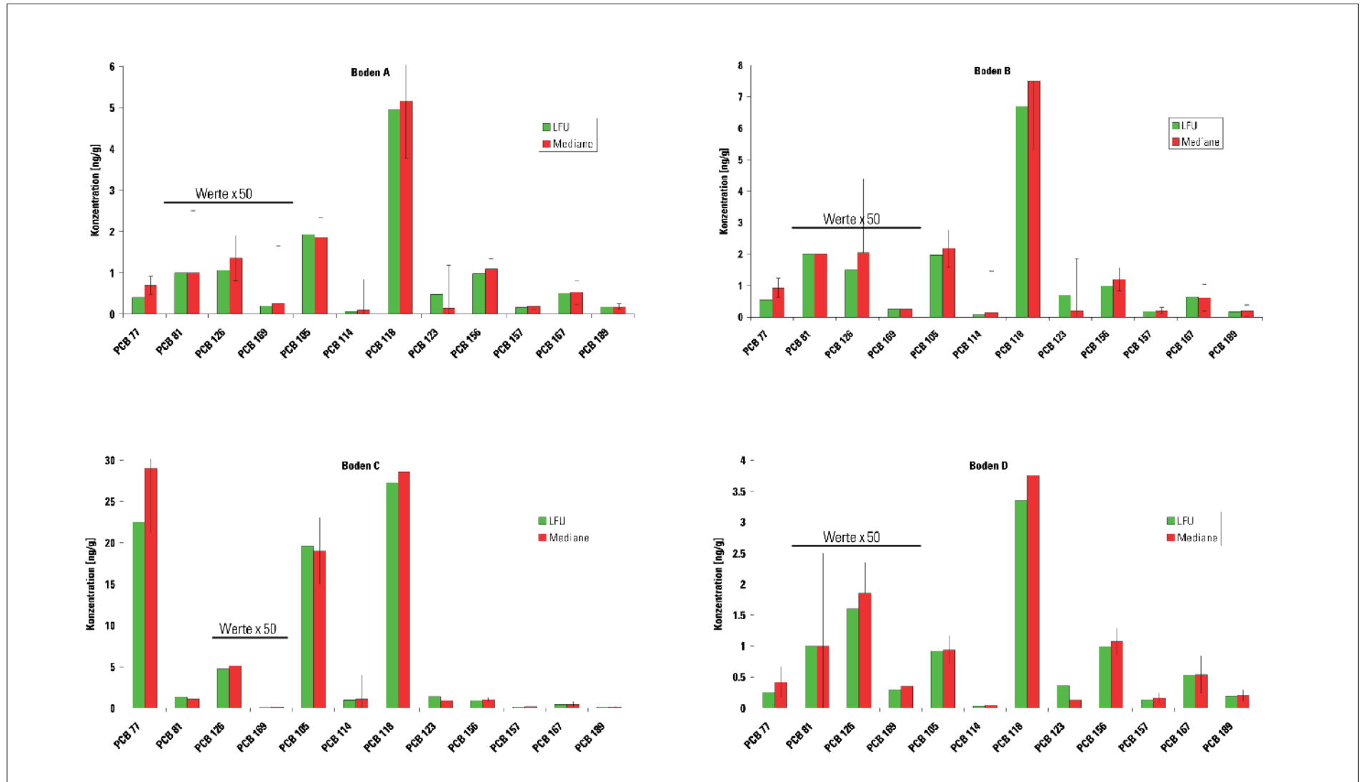
Abb. 8: Vergleich der vom LfU ermittelten Konzentrationen [ng/g] mit den ausreißerbereinigten Labormedianen (+/- Standardabweichung) für die vier untersuchten Boden- und Sedimentproben. Der besseren Übersicht halber wurden hier die Konzentrationen einiger Kongenere mit einem Faktor 50 multipliziert.
