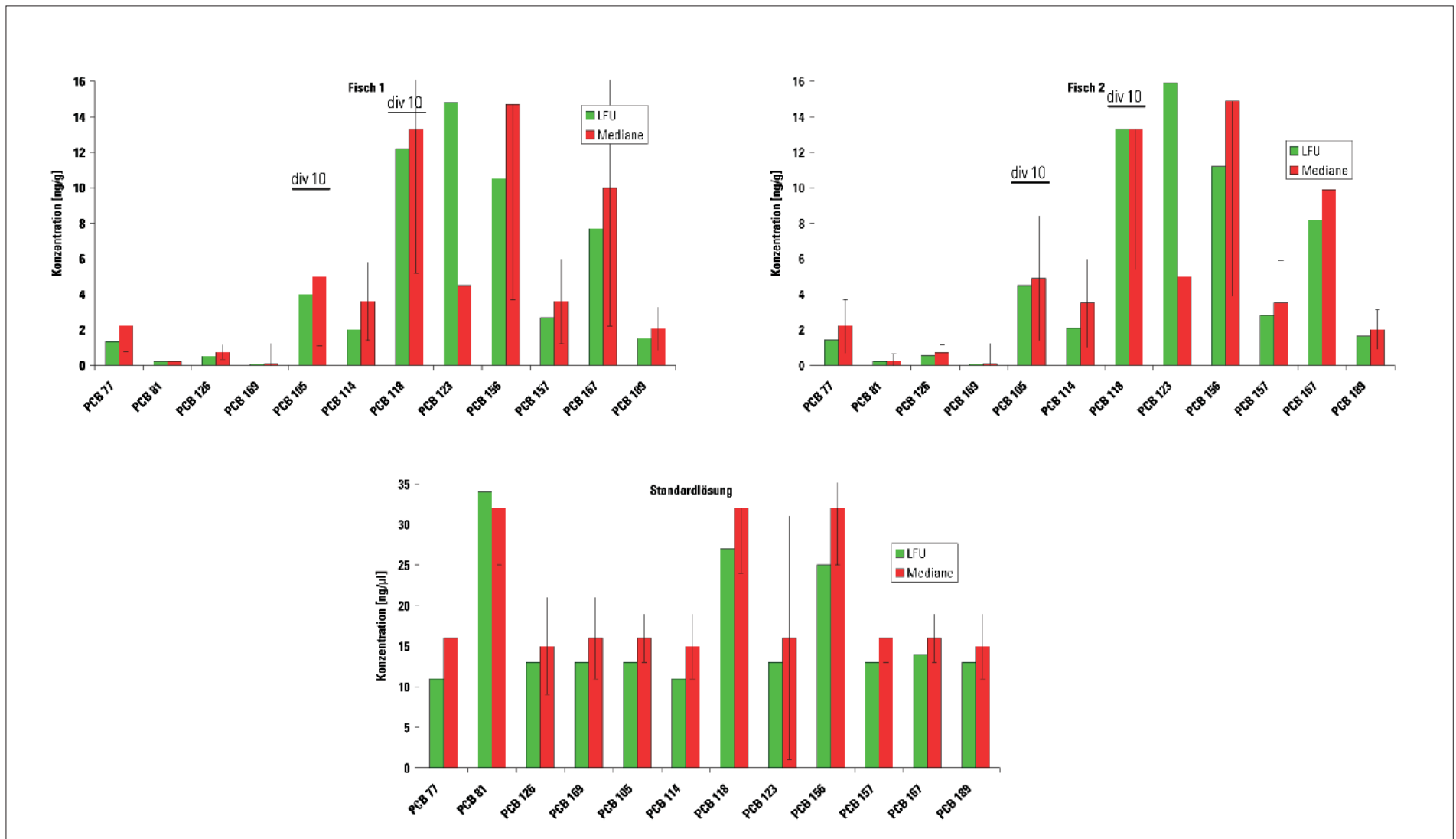
Abb. 9: Vergleich der vom LfU ermittelten Konzentrationen [ng/g] mit den ausreißerbereinigten Labormedianen für die untersuchten Fischproben und die Standardlösung. Der besseren Übersicht halber wurden hier die Konzentrationen einiger Kongenere in den Fischproben durch 10 dividiert.
