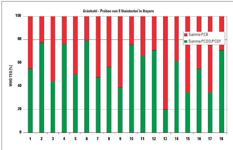
Abb. 12: TEQ Verteilung auf PCB und PCDD/PCDF in den Grünkohlproben 2001
