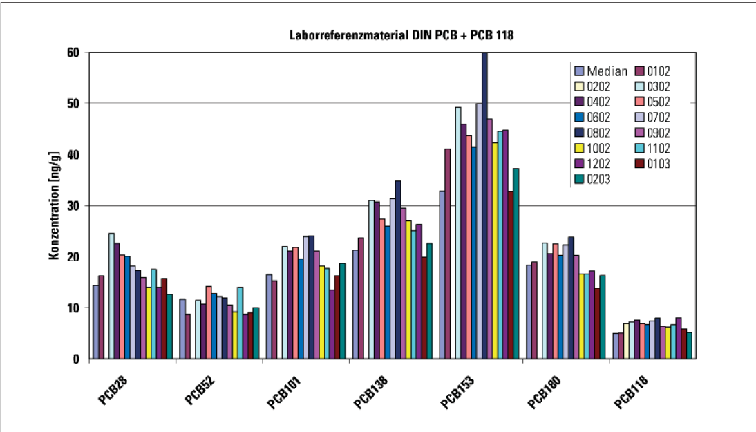
Abb. 2: Konzentrationen der Indikatorkongenere sowie von PCB 118 im Klärschlammreferenzmaterial – Aufarbeitungen Januar 2002 – Februar 2003
