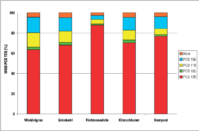
Abb. 21: Beitrag der einzelnen dioxinähnlichen PCB zum Toxizitätsäquivalent der PCB
