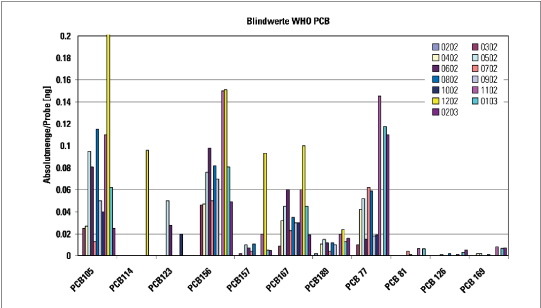
Abb. 5: Laborblindwerte der dioxinähnlichen PCB [ng/Probe] seit Februar 2002
