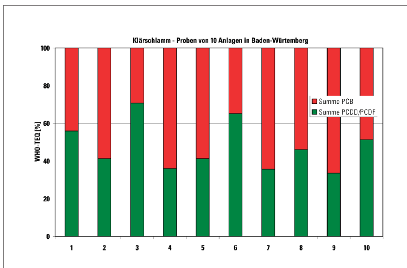
Abb. 16: TEQ Verteilung auf PCB und PCDD/PCDF von Klärschlämmen aus kommunalen Kläranlagen – Baden-Württemberg
