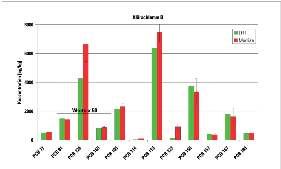
Abb. 7: Vergleich der vom LfU ermittelten Konzentrationen [ng/kg] mit den ausreißerbereinigten Labormedianen (+/- Standardabweichung) für Klärschlammprobe B. Der besseren Übersicht halber wurden auch hier die Konzentrationen der drei non-ortho PCB 81, 126 und 169 mit einem Faktor 50 multipliziert.
