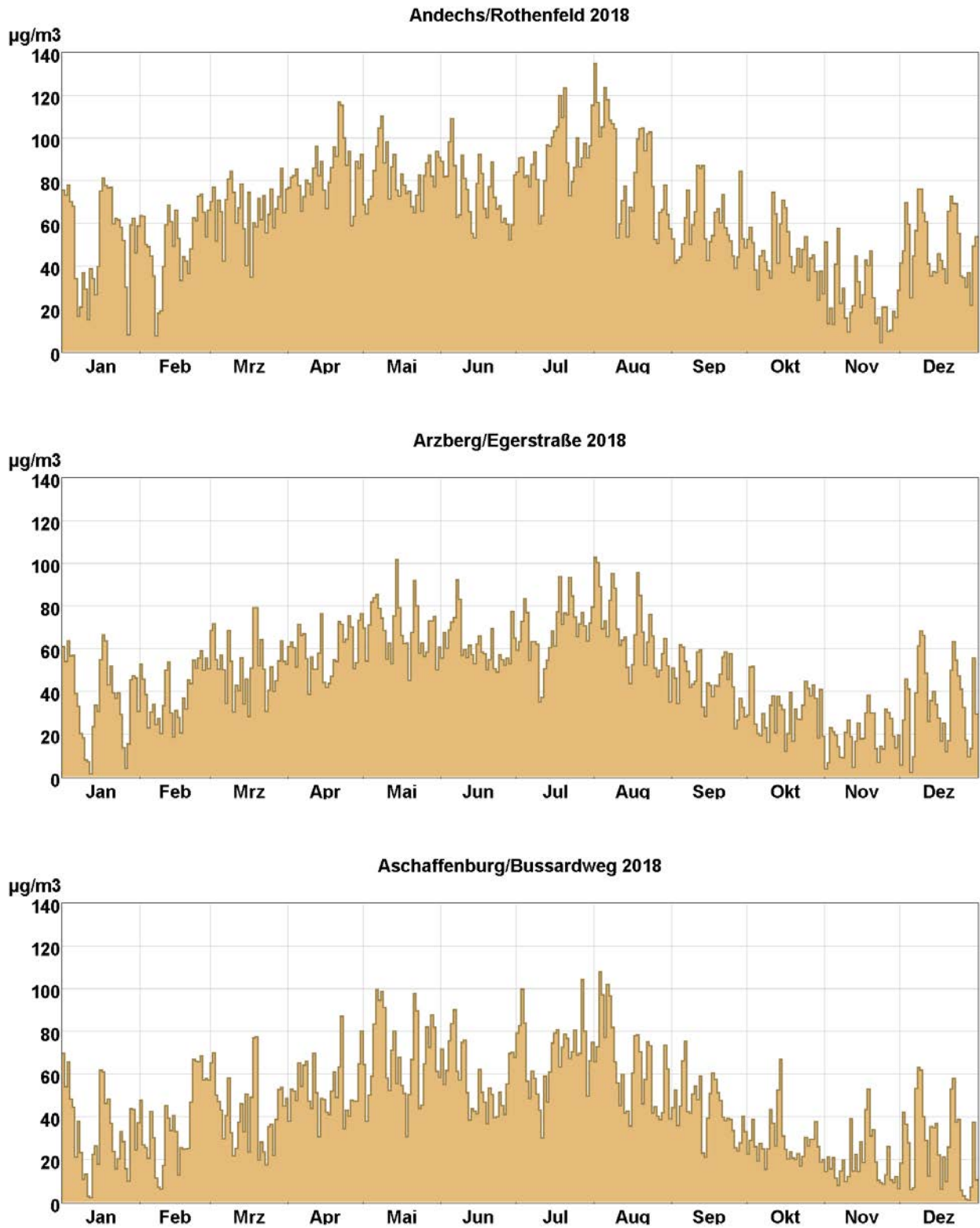
Abb. 2: Tagesmittelwertverläufe von Ozon an den mit Ozonmonitoren ausgestatteten LÜB-Messtationen.
