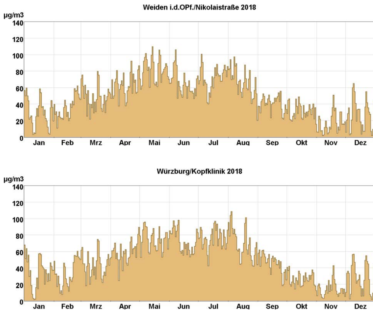
Abb. 2 (Forts.): Tagesmittelwertverläufe von Ozon an den mit Ozonmonitoren ausgestatteten LÜB-Messtationen.
