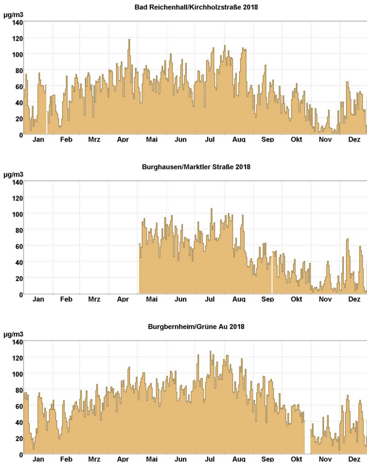
Abb. 2 (Forts.): Tagesmittelwertverläufe von Ozon an den mit Ozonmonitoren ausgestatteten LÜB-Messtationen.
