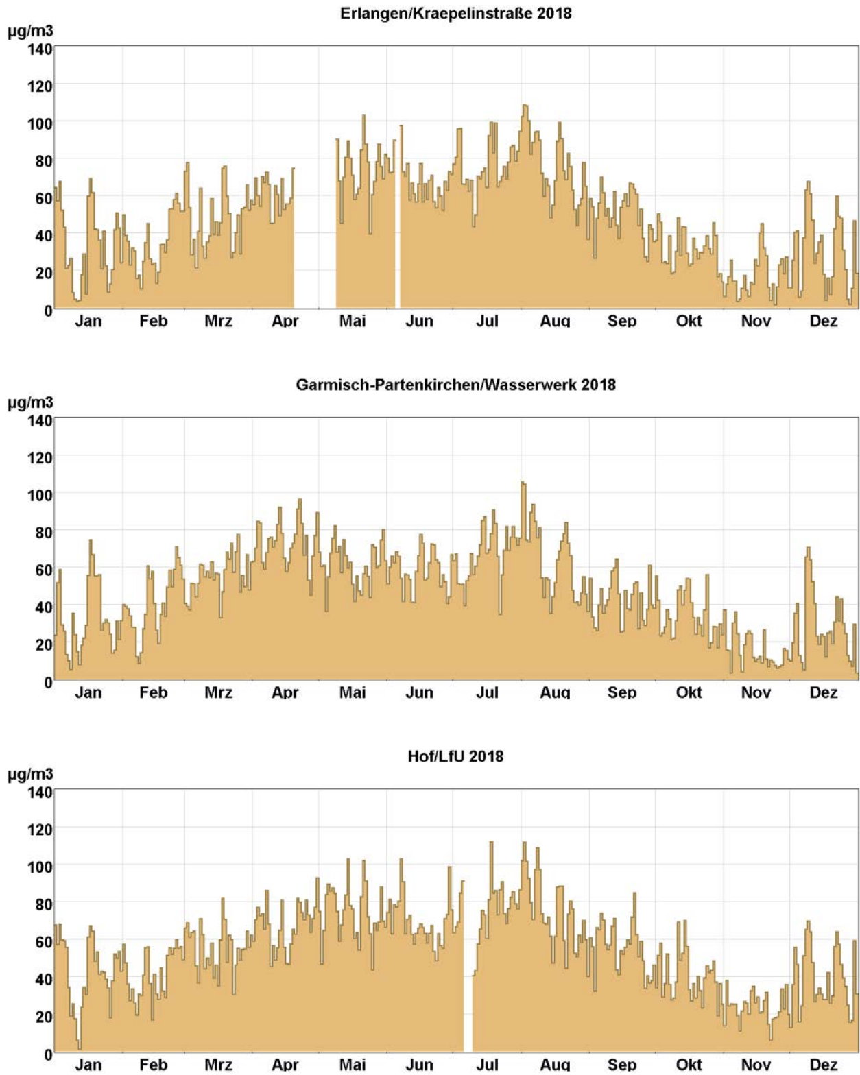
Abb. 2 (Forts.): Tagesmittelwertverläufe von Ozon an den mit Ozonmonitoren ausgestatteten LÜB-Messstationen.
