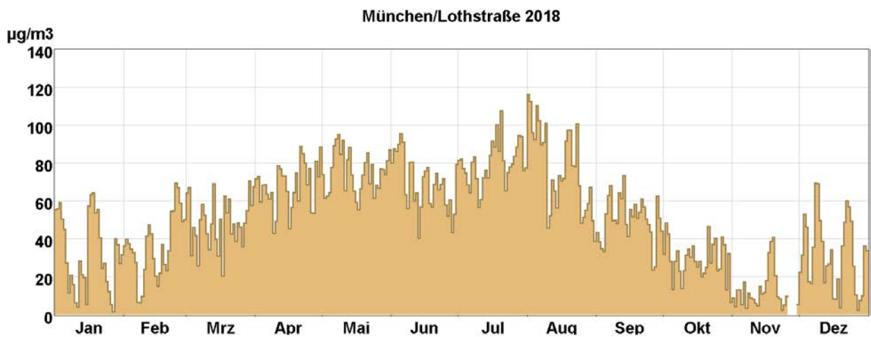
Abb. 2 (Forts.): Tagesmittelwertverläufe von Ozon an den mit Ozonmonitoren ausgestatteten LÜB-Messstationen.
