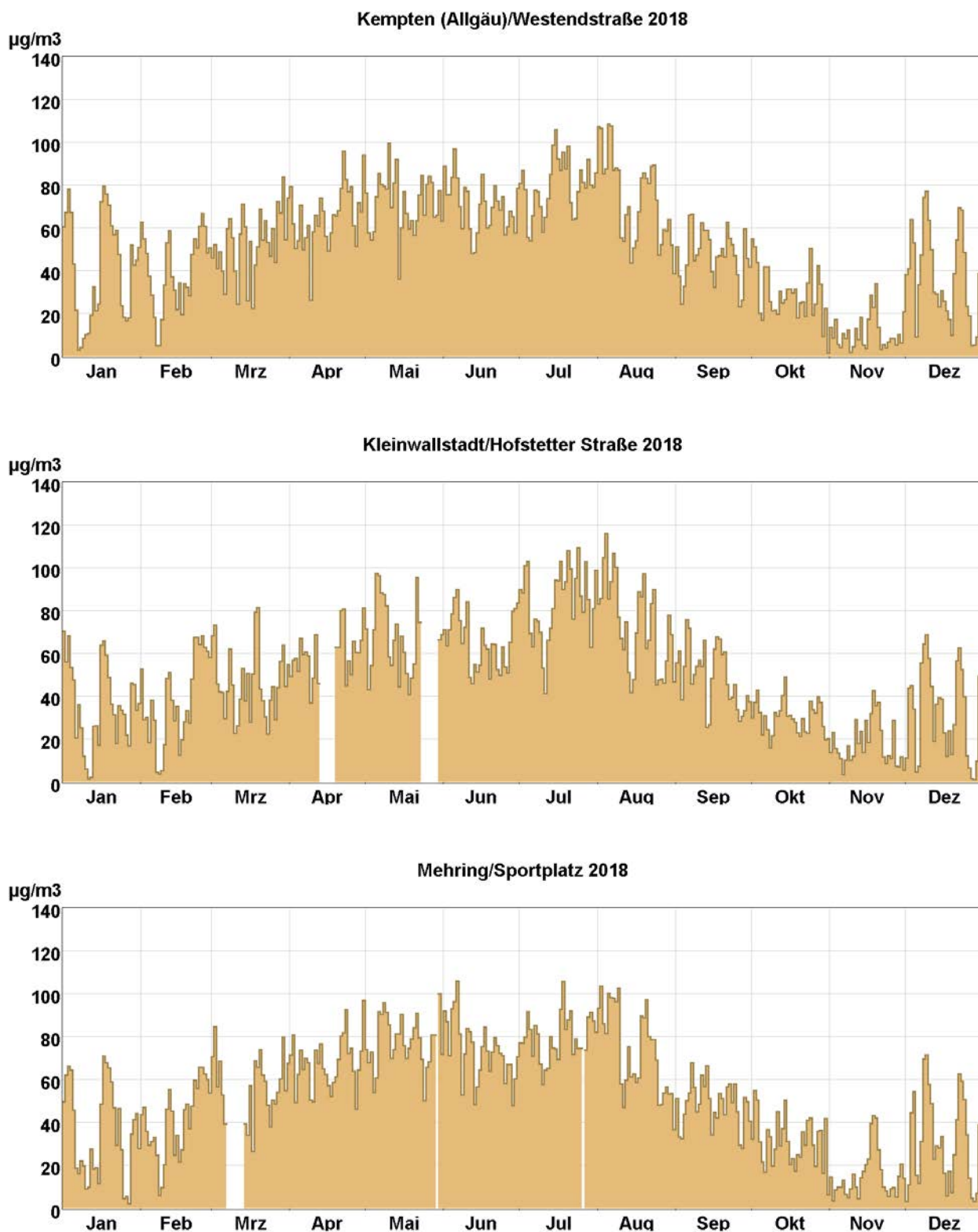
Abb. 2 (Forts.): Tagesmittelwertverläufe von Ozon an den mit Ozonmonitoren ausgestatteten LÜB-Messstationen.
