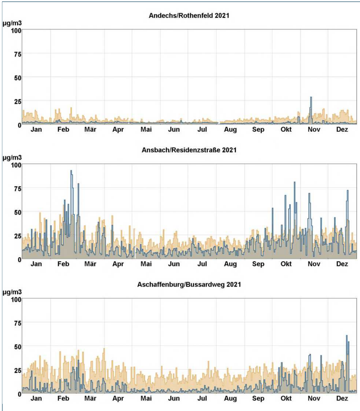
Abb. 2: Tagesmittelwertverläufe von Stickstoffmonoxid (blaue Stufenlinie) und Stickstoffdioxid (hellbraune Stufenlinie) an den mit Stickoxidmonitoren ausgestatteten LÜB-Messstationen.
