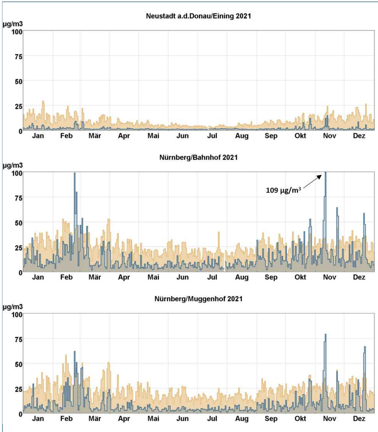
Abb. 12: Tagesmittelwertverläufe von Stickstoffmonoxid (blaue Stufenlinie) und Stickstoffdioxid (hellbraune Stufenlinie) an den mit Stickoxidmonitoren ausgestatteten LÜB-Messtationen.
