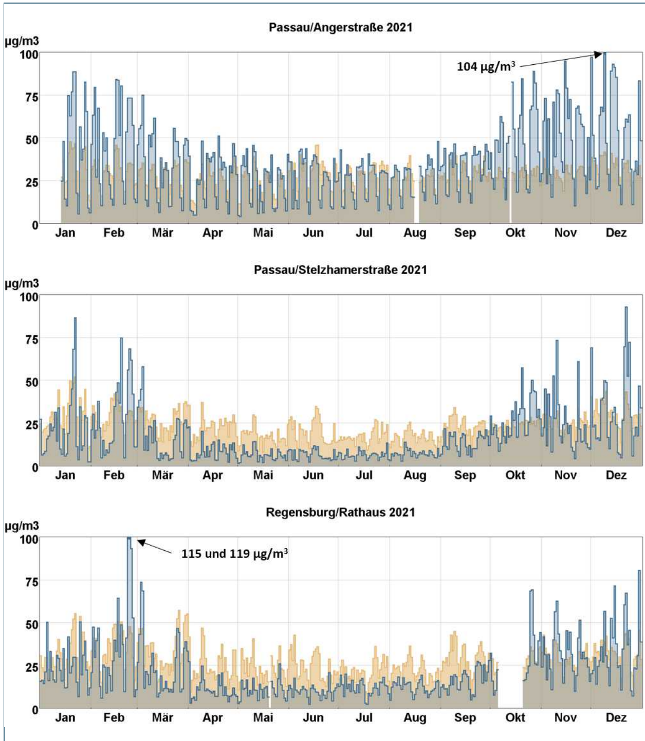
Abb. 14: Tagesmittelwertverläufe von Stickstoffmonoxid (blaue Stufenlinie) und Stickstoffdioxid (hellbraune Stufenlinie) an den mit Stickoxidmonitoren ausgestatteten LÜB-Messstationen.
