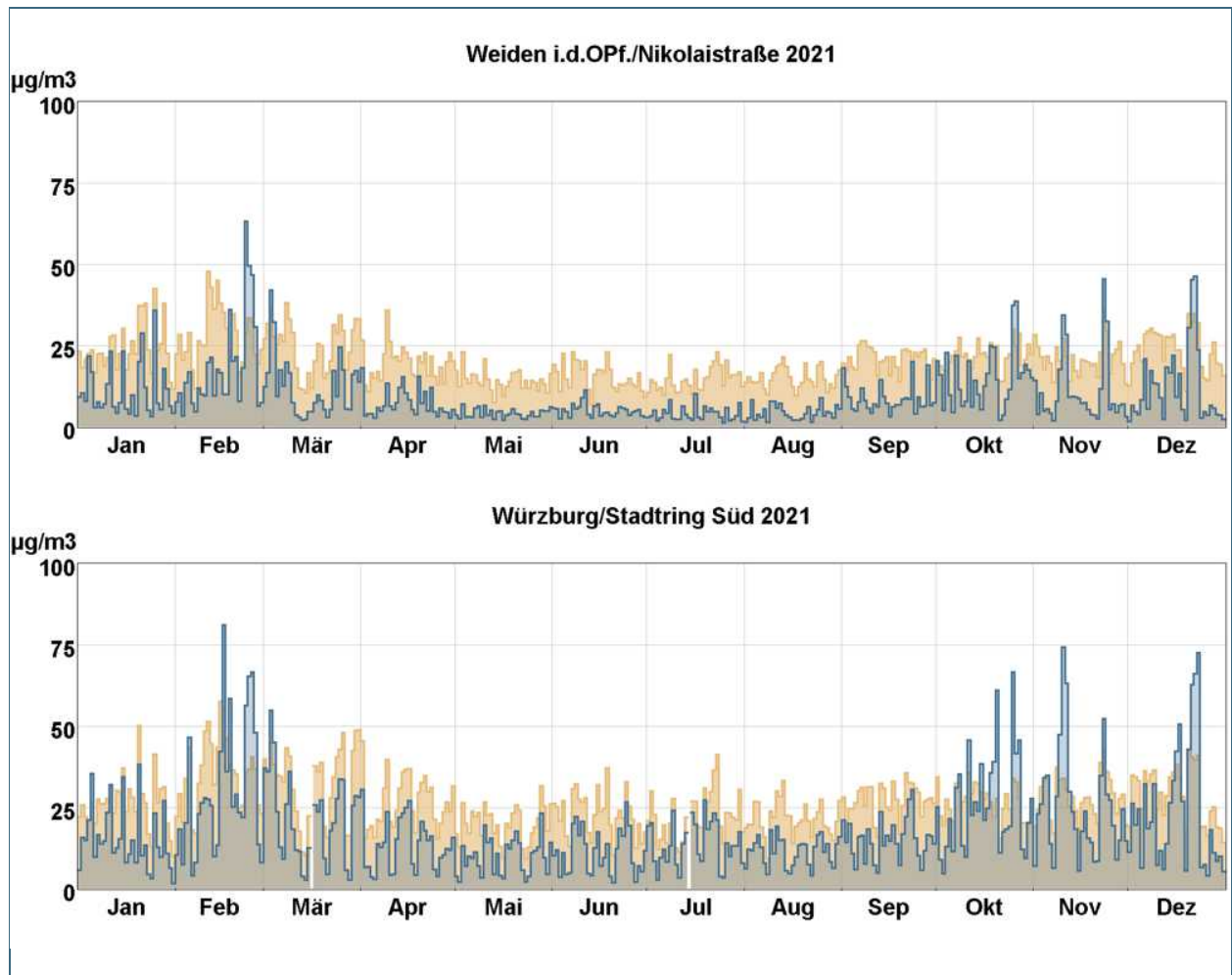
Abb. 17: Tagesmittelwertverläufe von Stickstoffmonoxid (blaue Stufenlinie) und Stickstoffdioxid (hellbraune Stufenlinie) an den mit Stickoxidmonitoren ausgestatteten LÜB-Messstationen.
