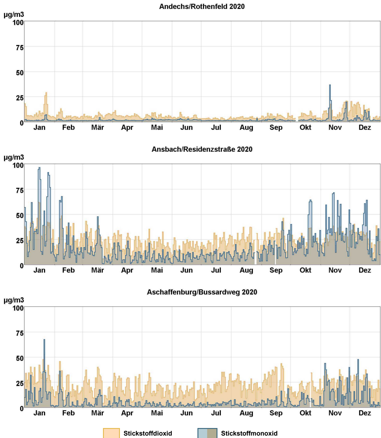
Abb. 2: Tagesmittelwertverläufe von Stickstoffmonoxid (NO) und Stickstoffdioxid (NO 2 ) an den mit Stickoxidmonitoren ausgestatteten LÜB-Messtationen
