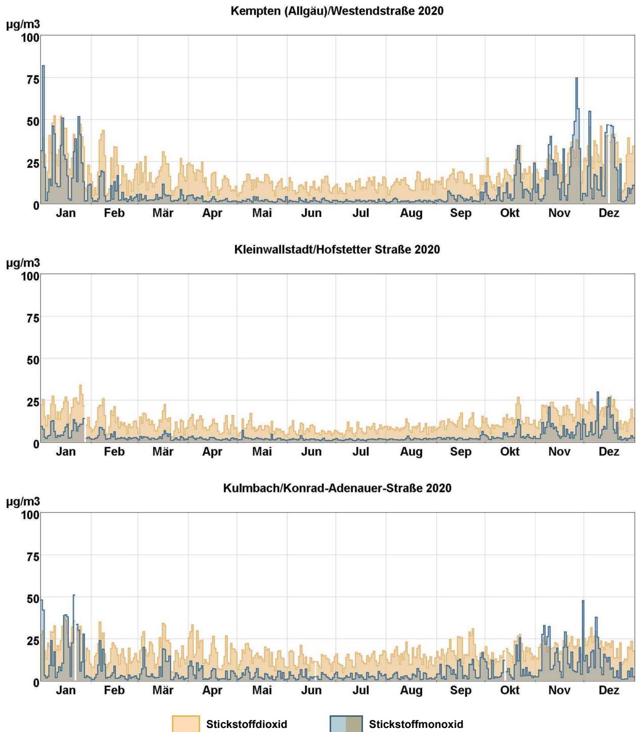
Abb. 2 (Forts.): Tagesmittelwertverläufe von Stickstoffmonoxid (NO) und Stickstoffdioxid (NO 2 ) an den mit Stickoxidmonitoren ausgestatteten LÜB-Messtationen.
