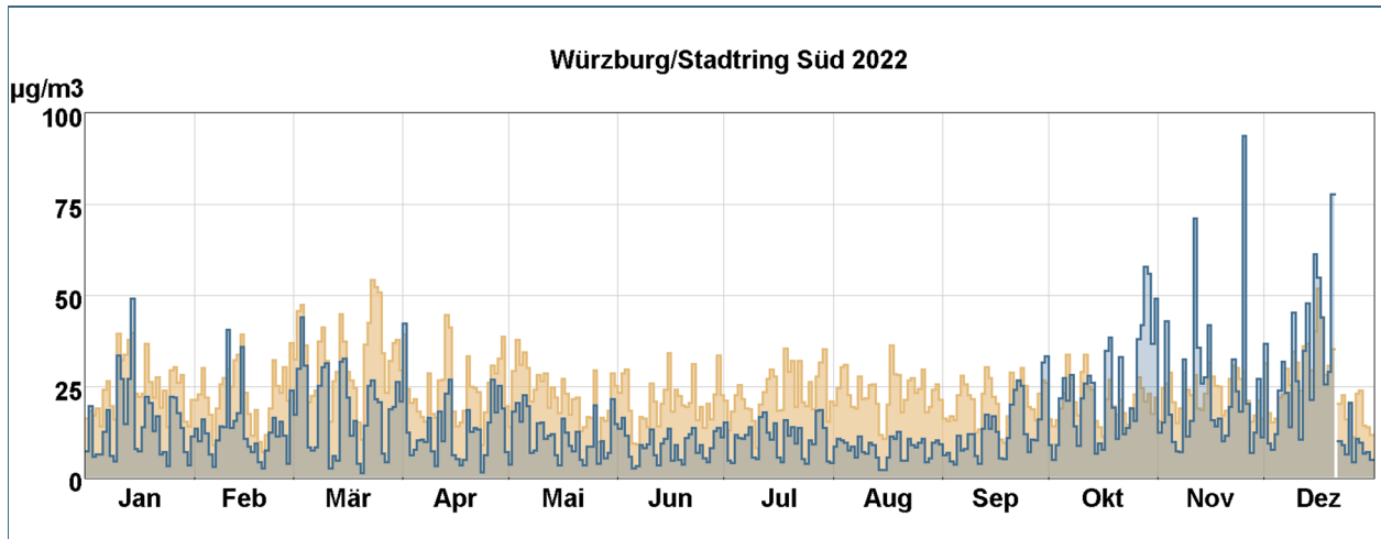
Abb. 18: Tagesmittelwertverläufe von Stickstoffmonoxid (blaue Stufenlinie) und Stickstoffdioxid (hellbraune Stufenlinie) an den mit Stickoxidmonitoren ausgestatteten LÜB-Messstationen.
