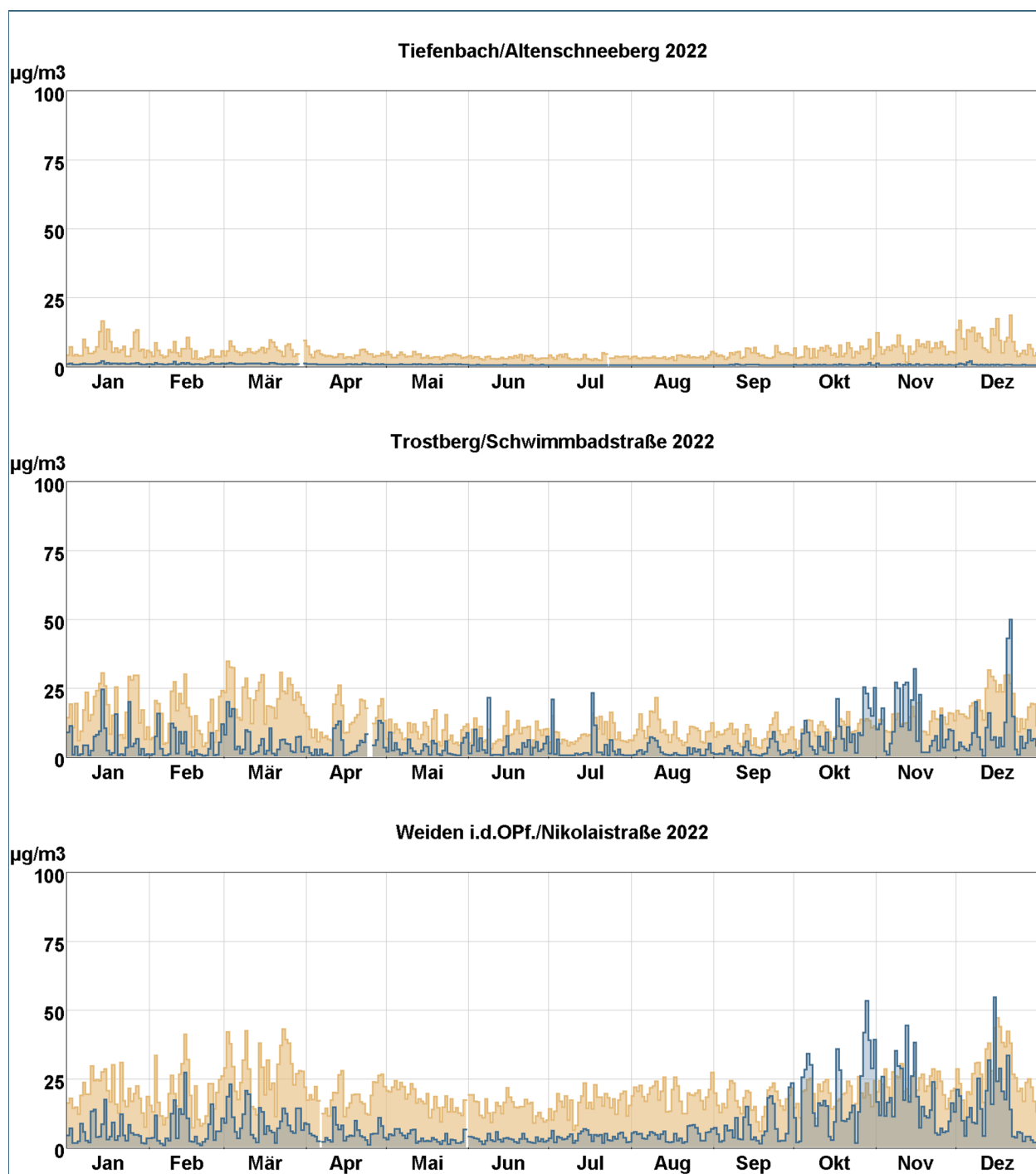
Abb. 17: Tagesmittelwertverläufe von Stickstoffmonoxid (blaue Stufenlinie) und Stickstoffdioxid (hellbraune Stufenlinie) an den mit Stickoxidmonitoren ausgestatteten LÜB-Messstationen.
